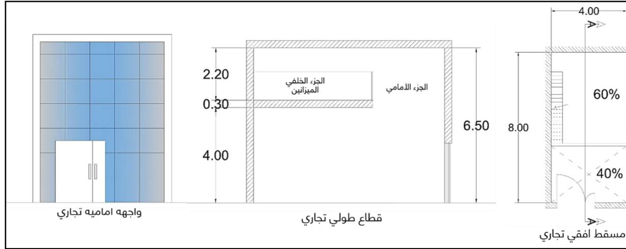
شكل رقم ١٨: طابق الميزانين في المحلات التجارية
