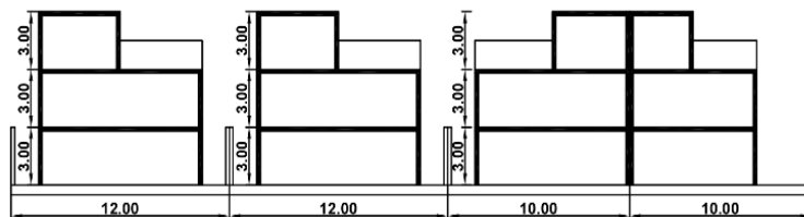
شكل رقم ٤: نماذج للفيلات المنفصلة والمتصلة
