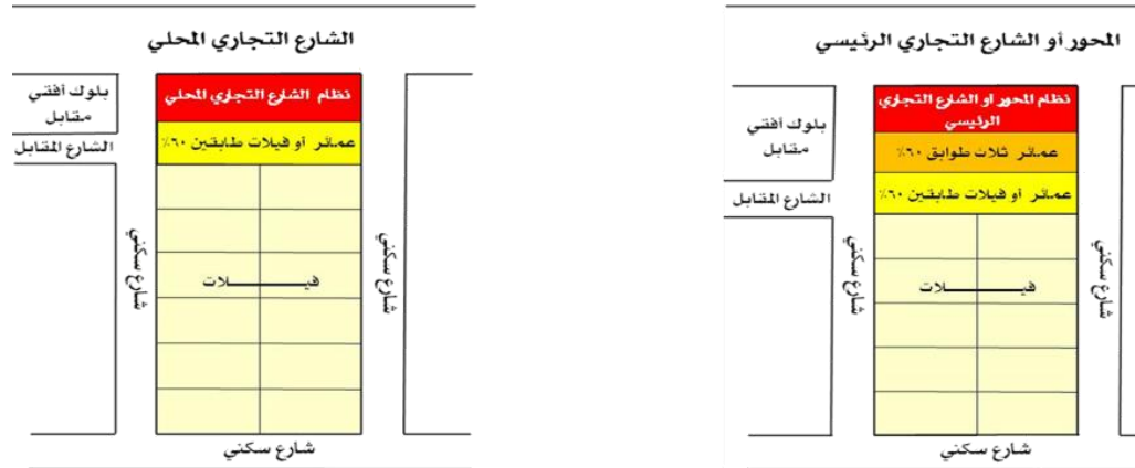
شكل رقم ٢٧: نظام البناء للقطع الخلفية للبلوكات العمودية بمنطقة الفيلات
