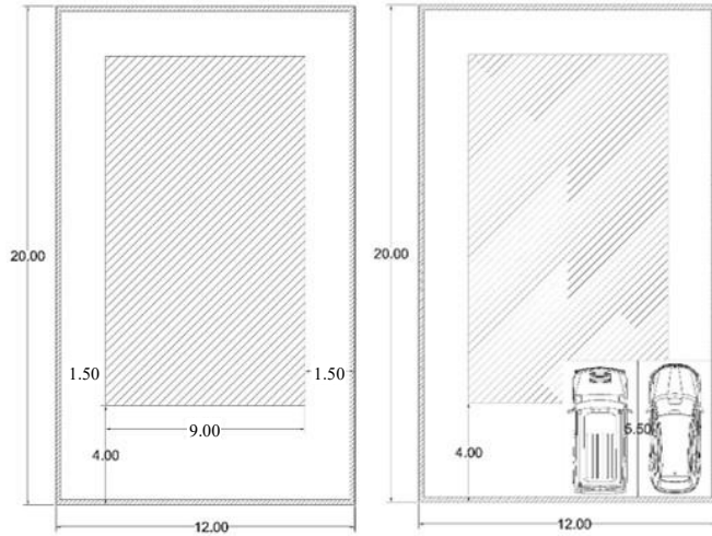
شكل رقم ٢٩: مواقف السيارات داخل حدود الملكية
