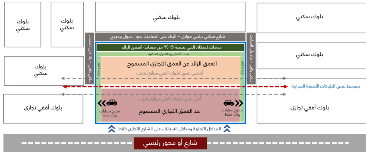
شكل رقم ٢٣: شكل توضيحي لموقع محاط بشوارع
