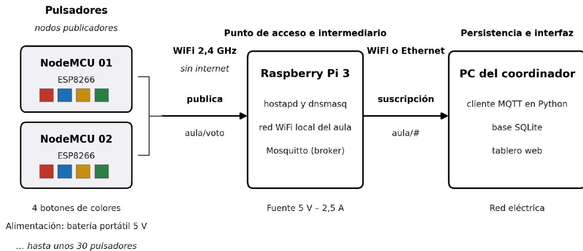
Figura 1. Esquema general de ClickAula: nodos publicadores, punto de acceso e intermediario de mensajes, y aplicación suscriptora.
