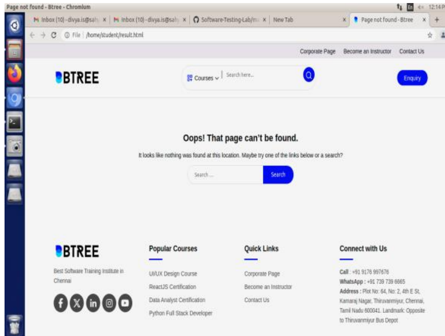
Figure1. Web Page
