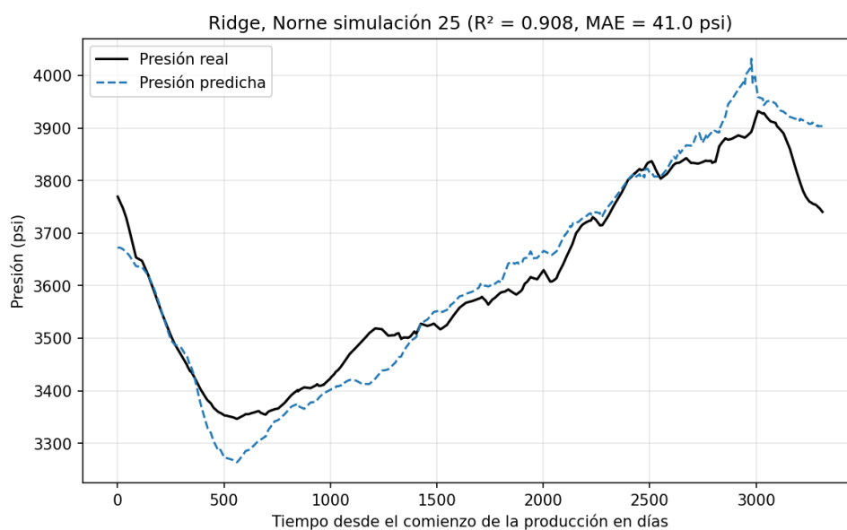
Figura 8: Comparación entre la presión real de Norne y la presión predicha por el modelo baseline
