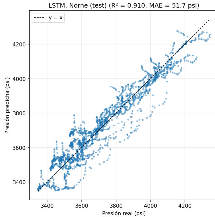
Figura 21: LSTM con encoder de PVT, test in-distribution sobre Norne: parity plot global.
