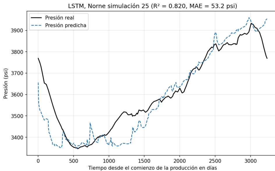
Figura 20: LSTM con encoder de PVT, test in-distribution sobre Norne: trayectoria de presión de una simulación representativa.
