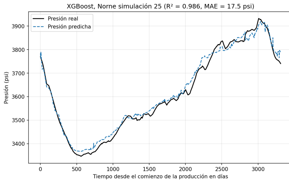
Figura 16: Comparación entre la presión real de Norne y la presión predicha por el modelo XGBoost
