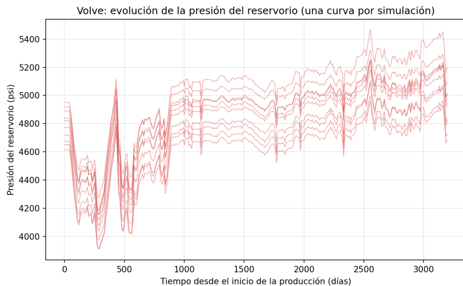
Figura 7: Presión en función del tiempo (simulaciones Volve)
