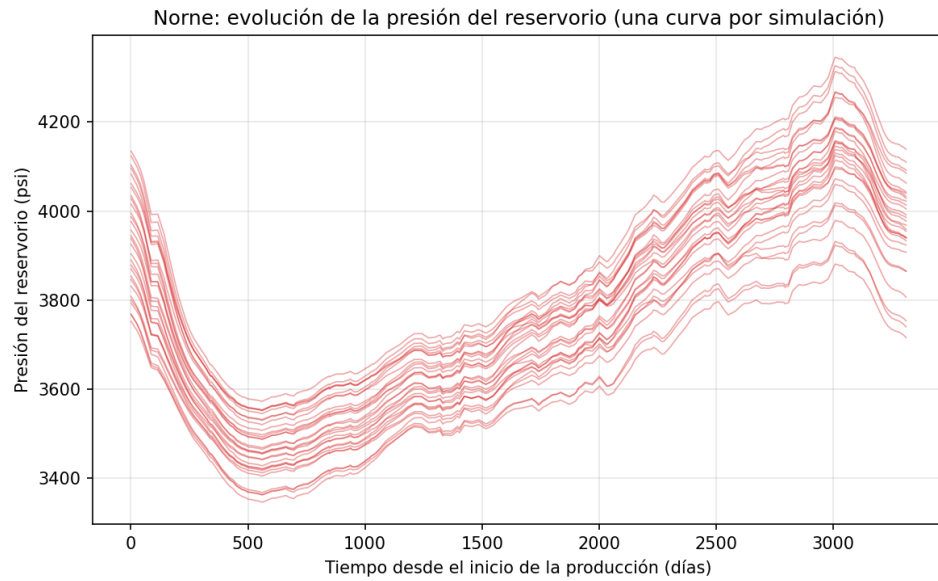
Figura 6: Presión en función del tiempo (simulaciones Norne)
