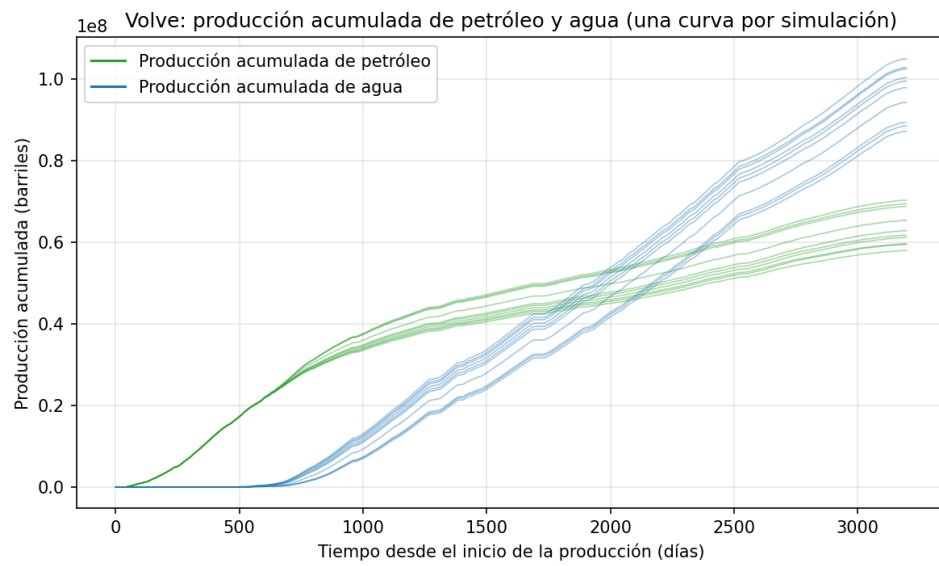
Figura 6: Producción acumulada de petróleo y agua (simulaciones Volve)
