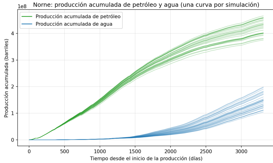
Figura 5: Producción acumulada de petróleo y agua (simulaciones Norne)
