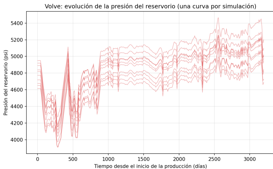
Figura 8: Presión en función del tiempo (simulaciones Volve)
