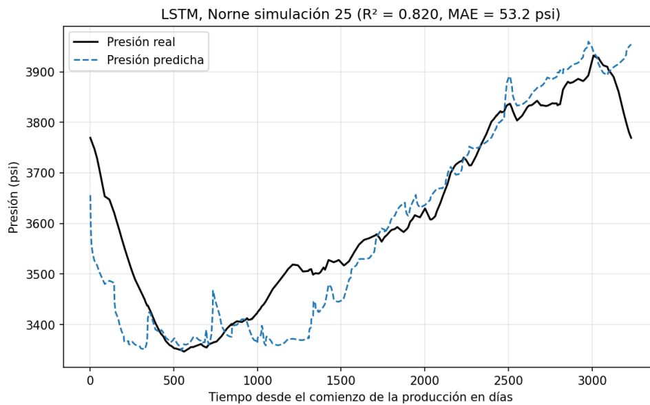
Figura 21: Comparación entre la presión real de Norne y la presión predicha por el modelo LSTM
