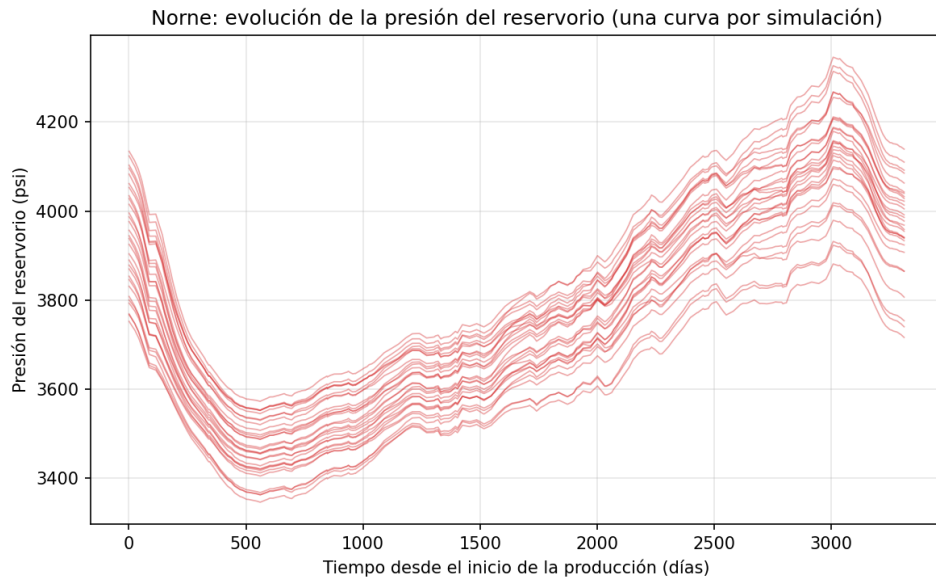
Figura 7: Presión en función del tiempo (simulaciones Norne)
