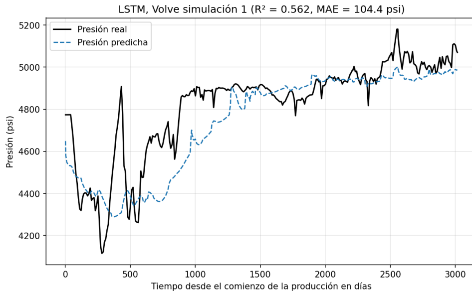
Figura 22: Comparación entre la presión real de Volve y la presión predicha por el modelo LSTM
