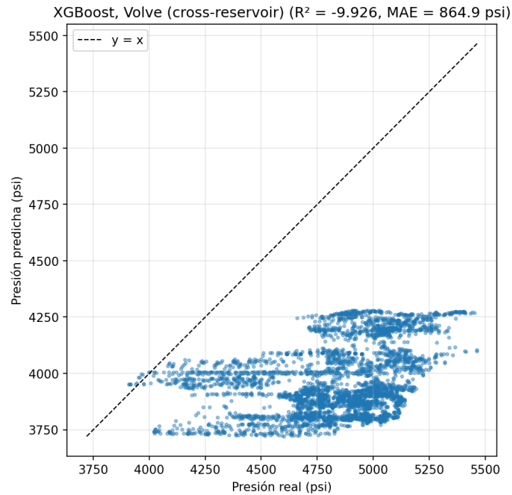
Figura 19: XGBoost, parity plot sobre Volve.
