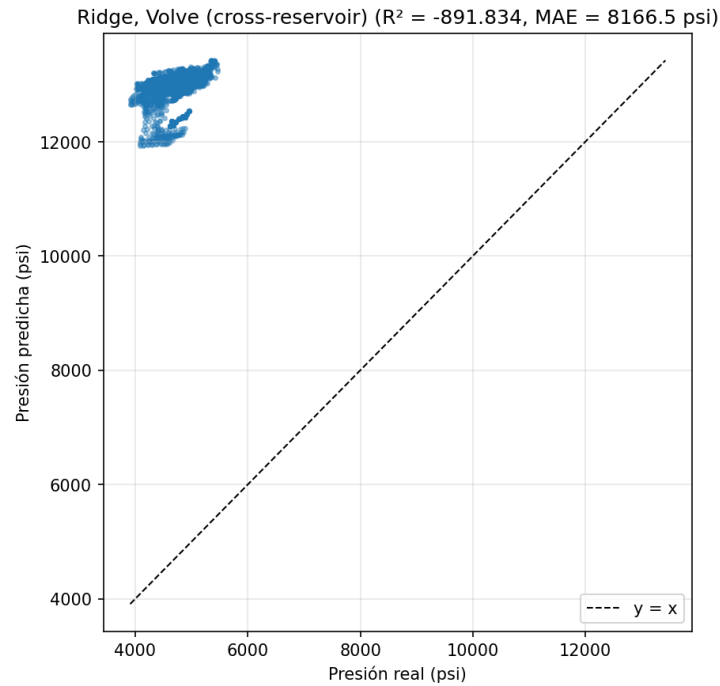
Figura 11: Baseline Ridge, parity plot sobre Volve. Las predicciones quedan muy por fuera del rango real de presión.
