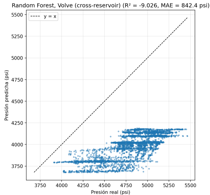
Figura 15: Random Forest, parity plot sobre Volve.
