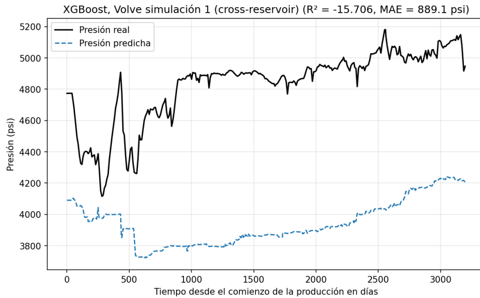
Figura 18: XGBoost, evaluación cross-reservoir sobre Volve: trayectoria de presión de una simulación representativa.
