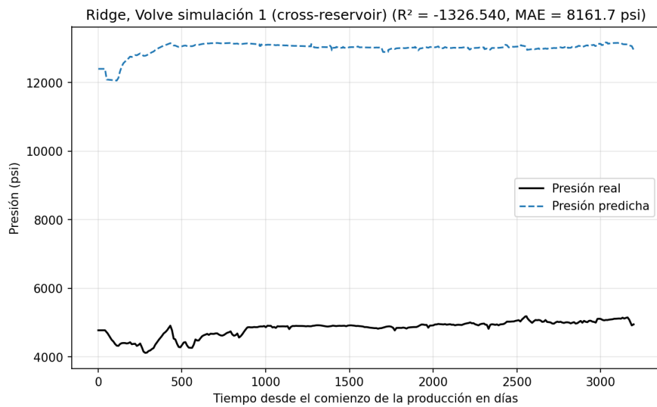
Figura 10: Baseline Ridge, evaluación cross-reservoir sobre Volve: trayectoria de presión de una simulación representativa.
