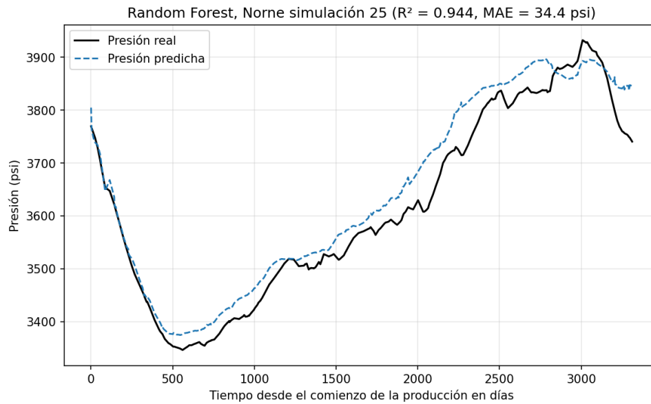
Figura 12: Random Forest, test in-distribution sobre Norne: trayectoria de presión de una simulación representativa.
