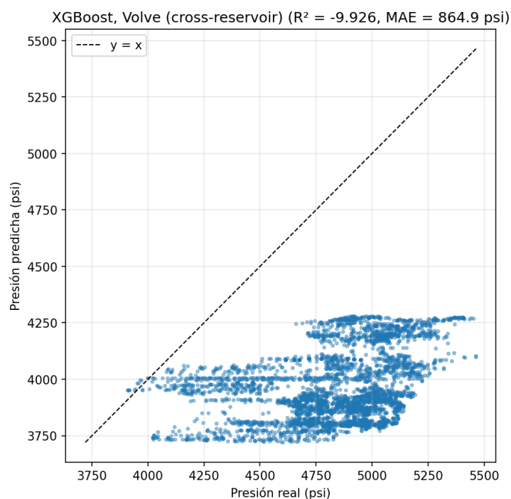
Figura 19: Parity plot entre la presión real de Volve vs. la presión predicha por el modelo XGBoost
