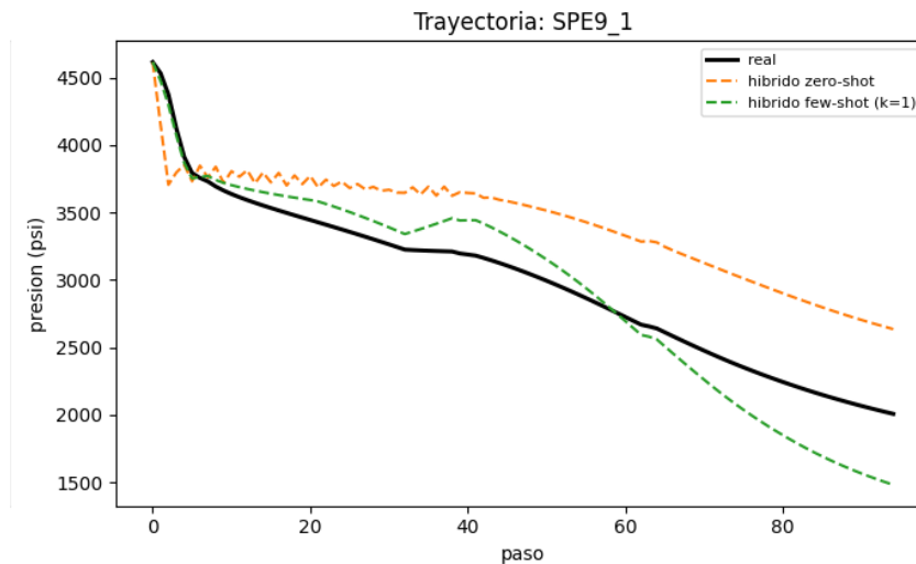
Figura 30: Trayectoria de presión en una simulación de SPE9 no usada para calibrar: real, híbrido zero-shot e híbrido few-shot (1 sim). La calibración de dos parámetros físicos corrige el sesgo del zero-shot y recupera la forma de la caída.
