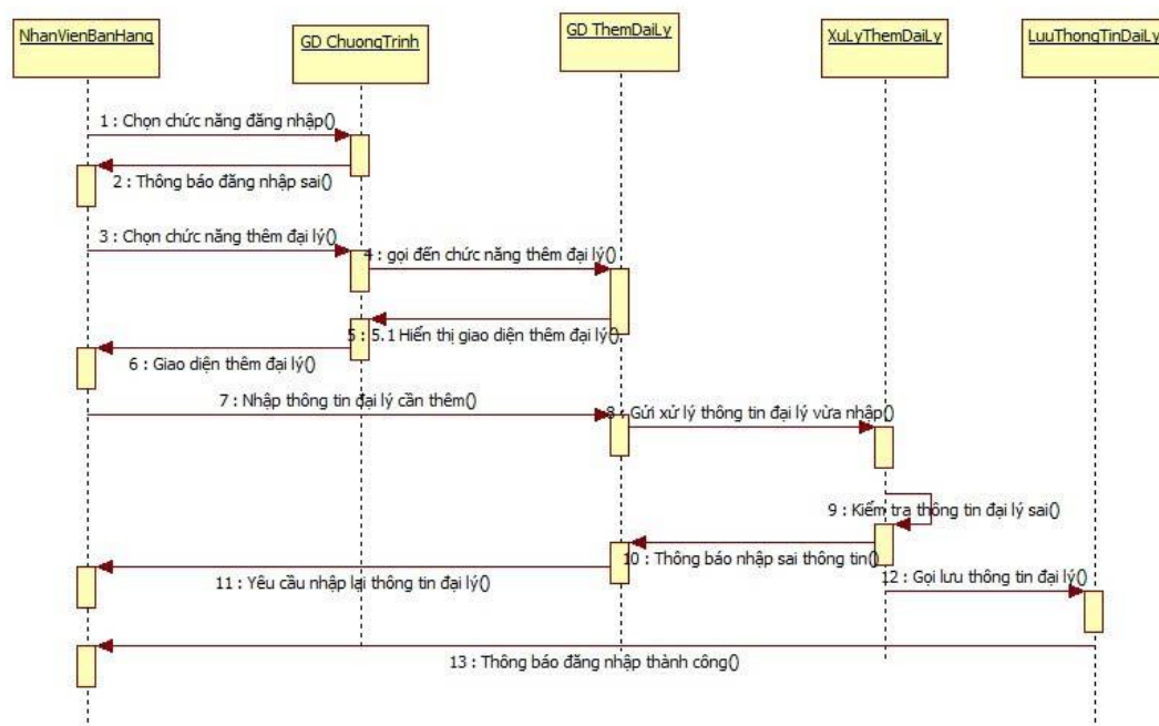
Hình 5. Sơ đồ tuần tự usecase Thêm mới thông tin đại lý
