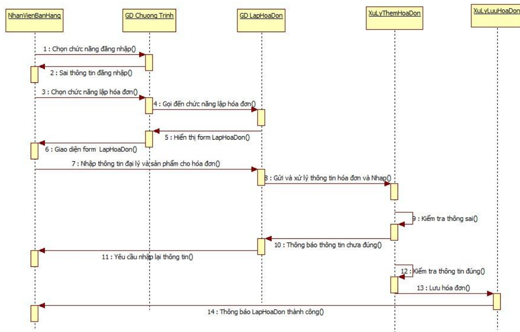
Hình 7. Sơ đồ tuần tự usecase Lập hóa đơn
