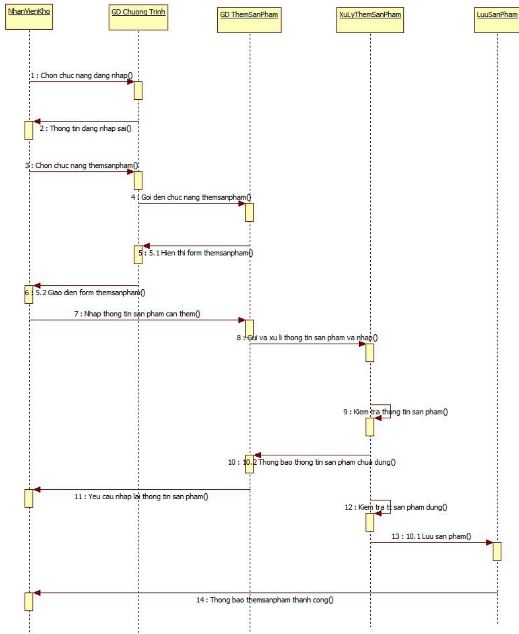
Hình 6. Sơ đồ tuần tự usecase Thêm thông tin sản phẩm.
