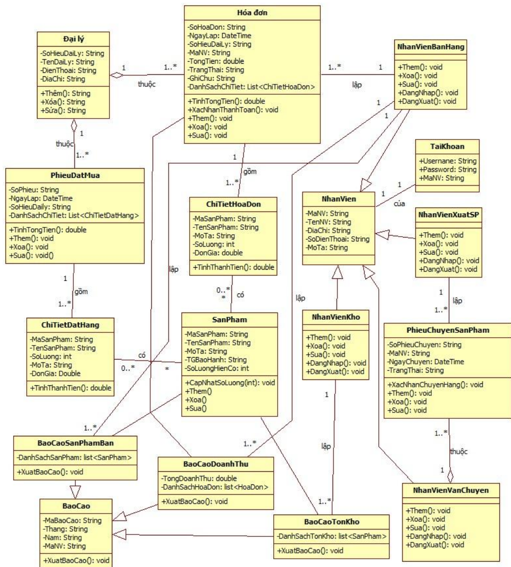
Hình 8. Sơ đồ lớp.
