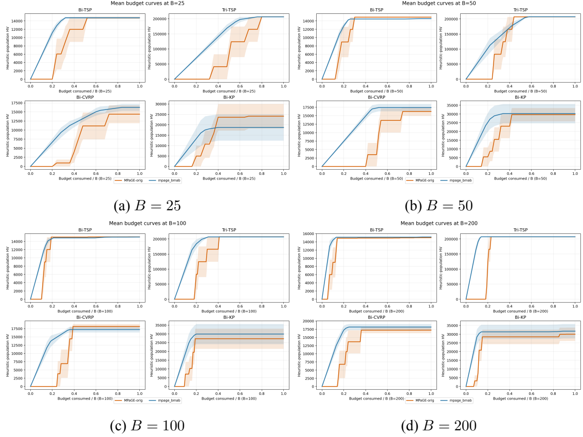
Hình 5.3: Đường cong HV theo ngân sách chuẩn hóa. Nguồn: các tệp budget_curves_B*.png trong mPage_bmb/experiments/results/images/ .
