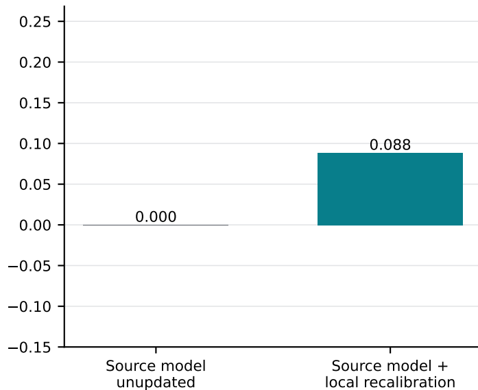
Update alpha
