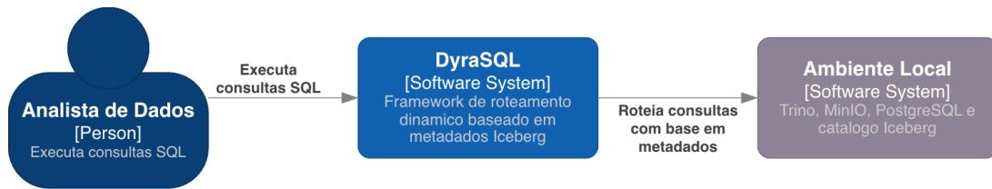
Figura 2 – Contexto do Sistema - DyraSQL
