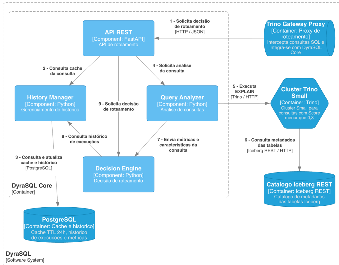
Figura 4 – Componentes do DyraSQL Core
