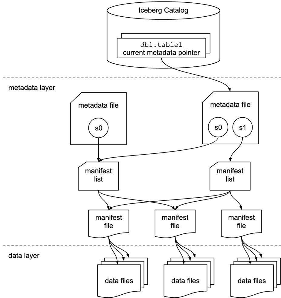
Figura 1 – Estrutura de Metadados do Apache Iceberg
