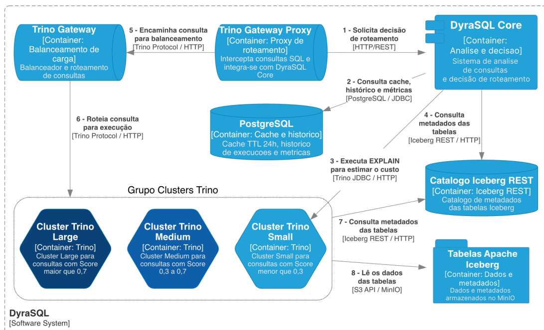
Figura 3 – Containers do Sistema - DyraSQL
