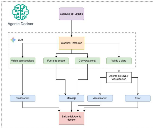
Figura 2: Diagrama de flujo del Agente Decisor. Según la clasificación de intención, el agente enruta la consulta hacia el pipeline de datos, solicita clarificación o emite un mensaje directo.
