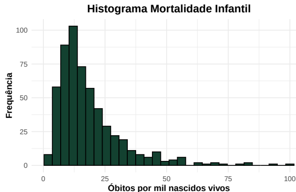
(a) Figura 15: Histograma mortalidade infantil
