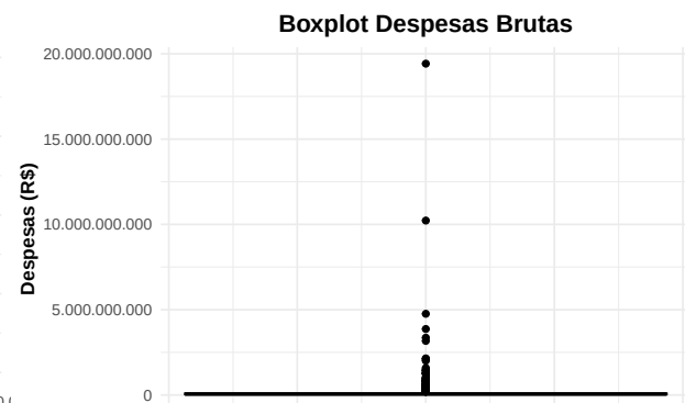
(a) Figura 20: Boxplot Despesas brutas
