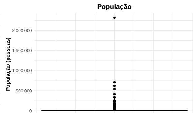
(a) Figura 6: Boxplot população
