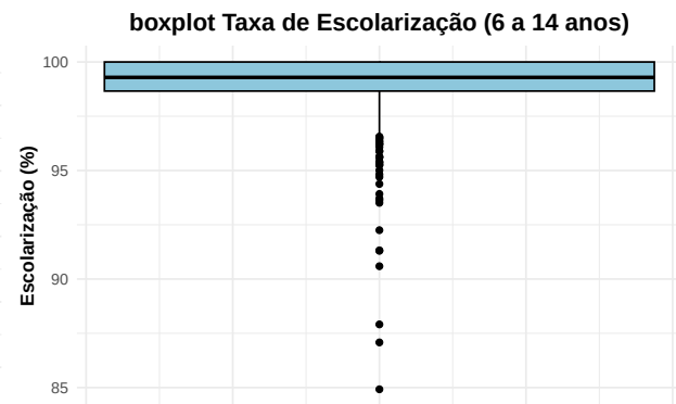
(a) Figura 12: Boxplot escolarização
