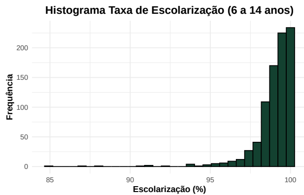
(a) Figura 11: Histograma escolarização
