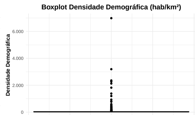
(a) Figura 8: Boxplot densidade demográfica
