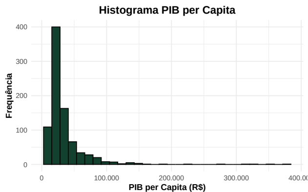
(a) Figura 21: Histograma PIB per capita
