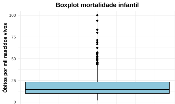
(a) Figura 16: Boxplot mortalidade infantil
