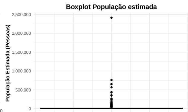
(a) Figura 10: Boxplot população estimada
