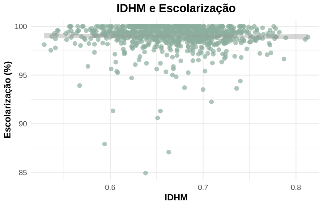
Figure 26: Figura 27: Gráfico de gráfico de dispersão com reta de regressão linear de IDHM e escolarização
