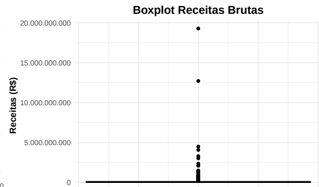
(a) Figura 18: Boxplot Receitas brutas
