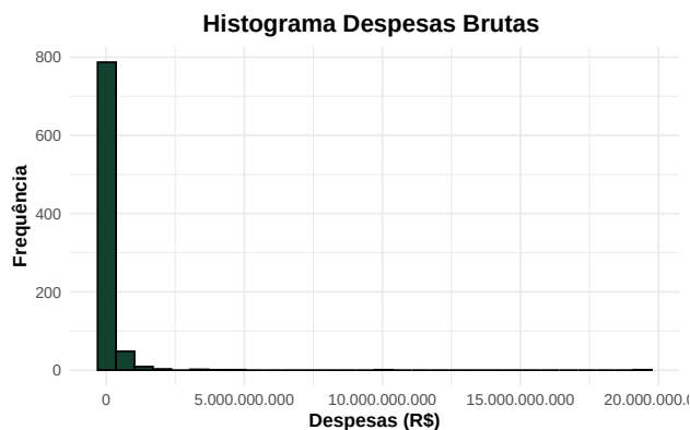
(a) Figura 19: Histograma Despesas brutas
