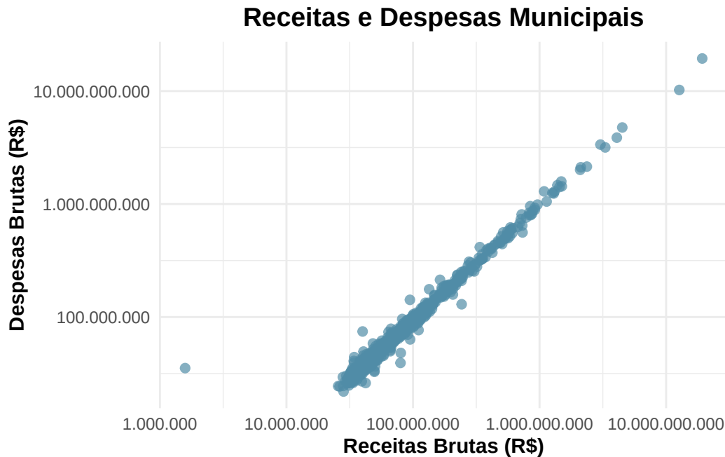
Figure 28: Figura 29: Gráfico de dispersão com escala logarítmica de Receitas e despesas municipais
