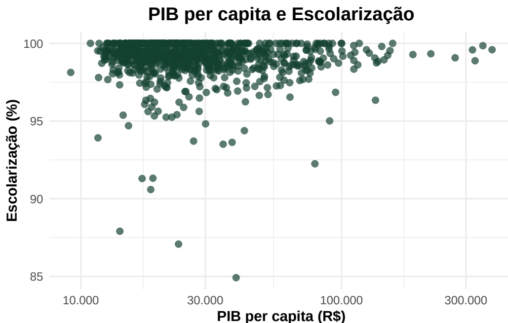
Figure 24: Figura 25: Gráfico de dispersão PIB per capita e escolarização
