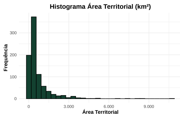
(a) Figura 3: Histograma área territorial
