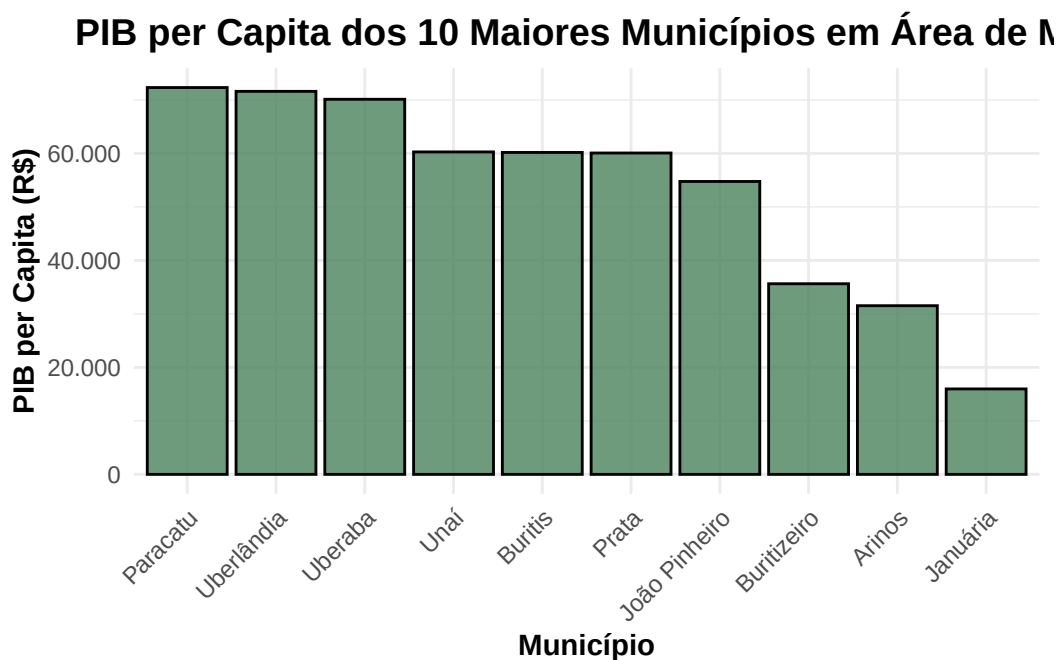
Figure 23: Figura 23: Gráfico de barras do PIB per capita dos 10 maiores municípios em área de MG
