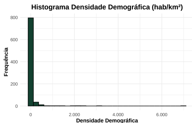
(a) Figura 7: Histograma densidade demográfica
