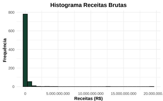
(a) Figura 17: Histograma Receitas brutas
