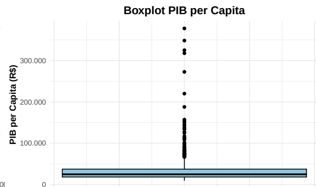
(a) Figura 22: Boxplot PIB per capita
