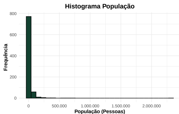
(a) Figura 5: Histograma população
