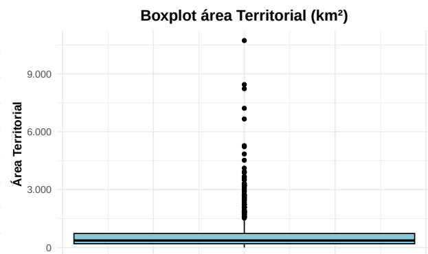
(a) Figura 4: Boxplot área territorial
