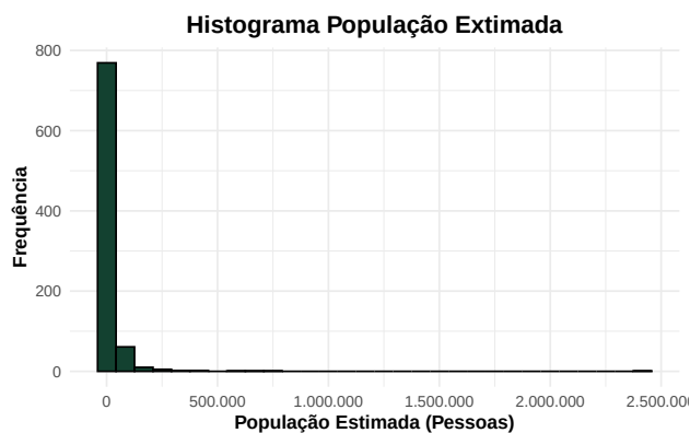
(a) Figura 9: Histograma população estimada
