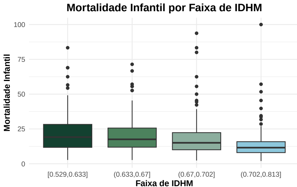
Figure 27: Figura 28: Gráfico boxplot de Mortalidade infantil por faixa de IDHM
