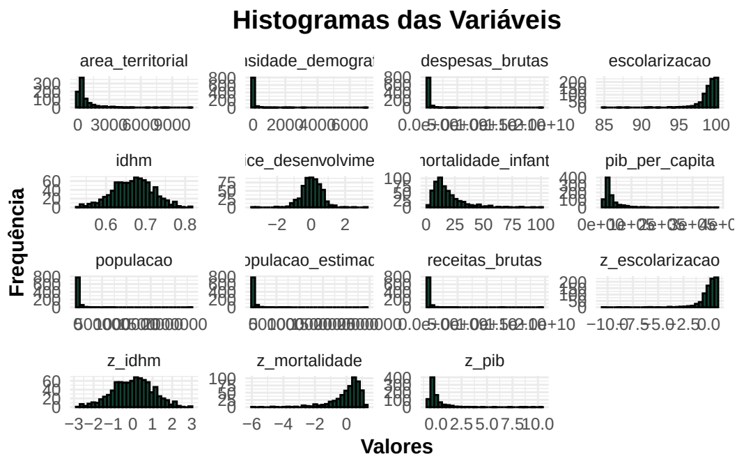
Figure 1: Figura 1: Histograma de todas as variáveis
