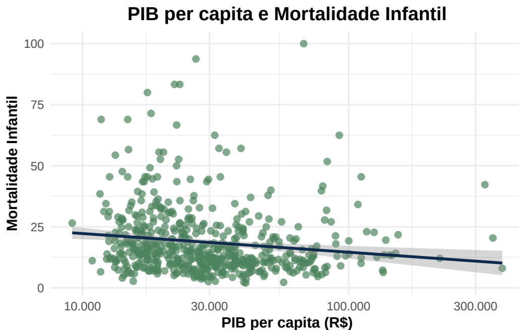
Figure 25: Figura 26: Gráfico de dispersão de PIB per capita e mortalidade infantil
