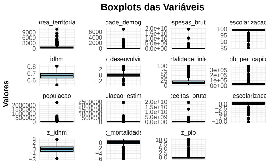
Figure 2: Figura 2: Boxplot de todas as variáveis
