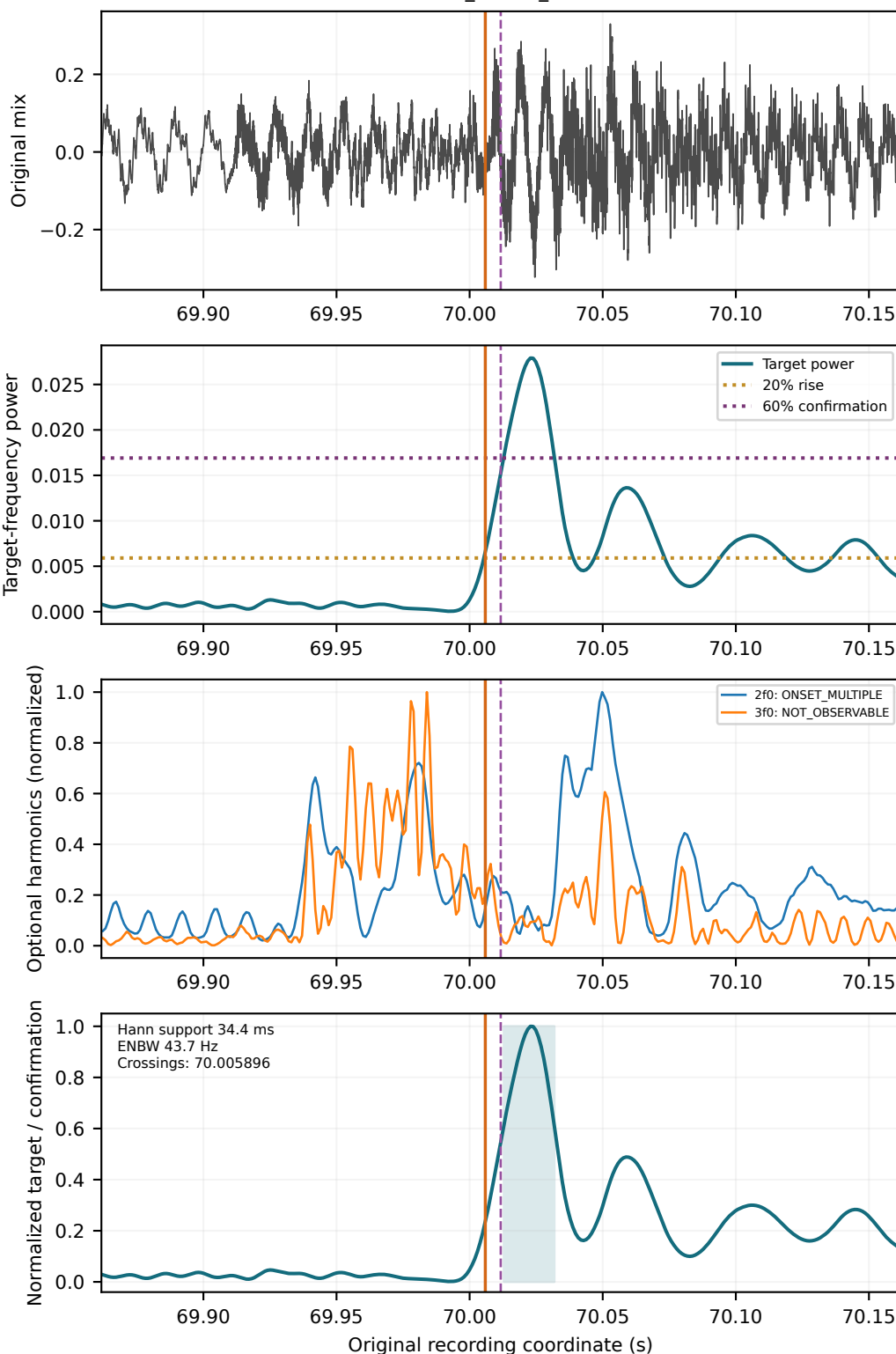
BP_0096 · A#2 · 116.54 Hz TARGET_ONSET_CLEAR
