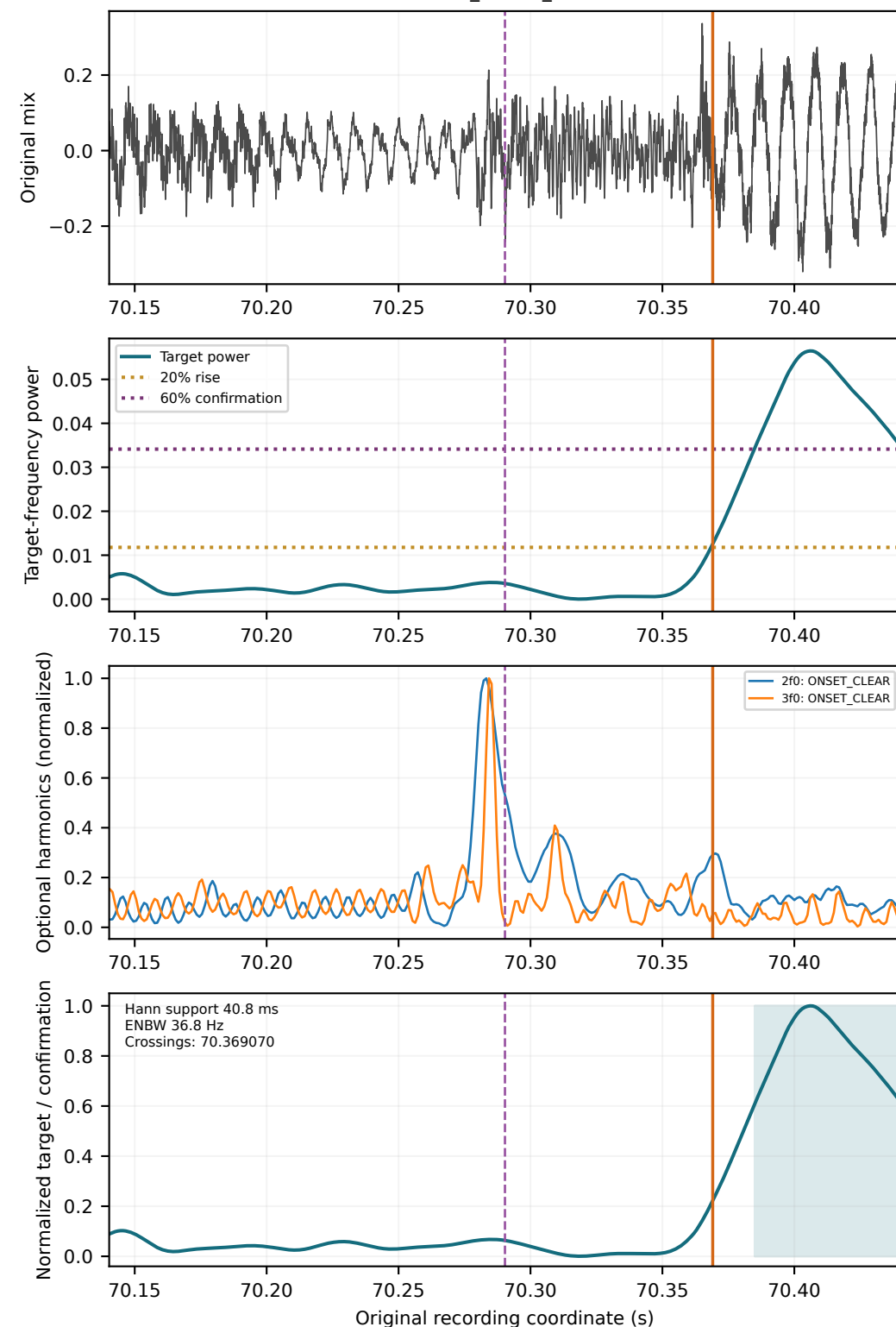
BP_0098 · G2 · 98.00 Hz TARGET_ONSET_CLEAR
