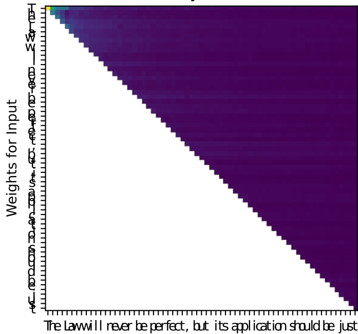
Input Layer 2
