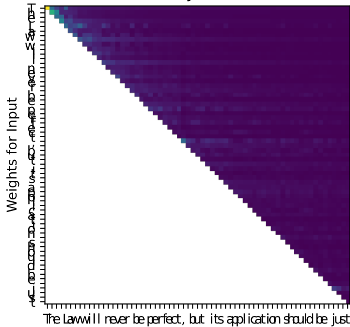
Input Layer 3
