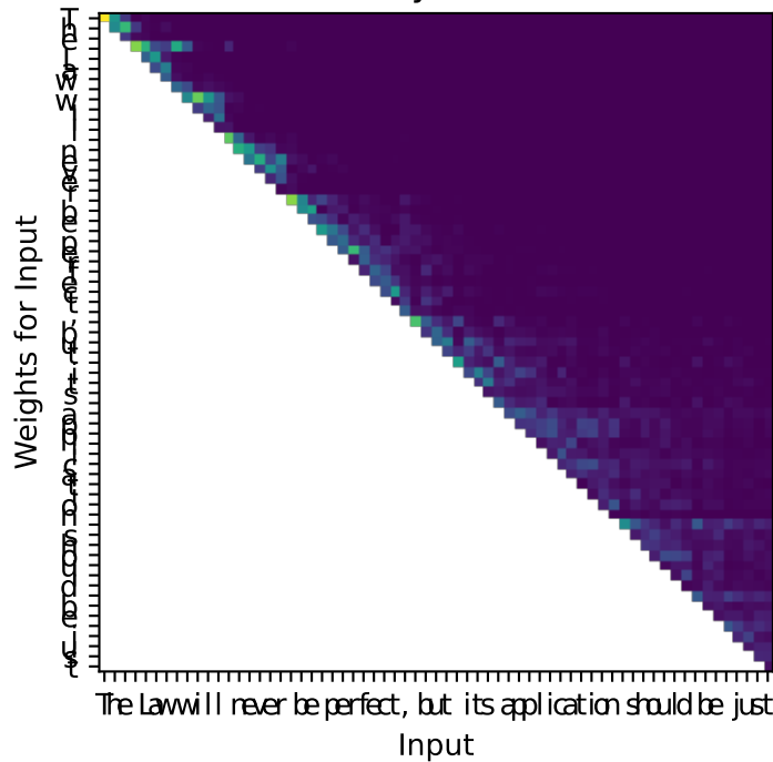
Input Layer 3
