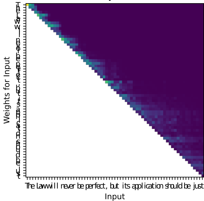
Input Layer 2
