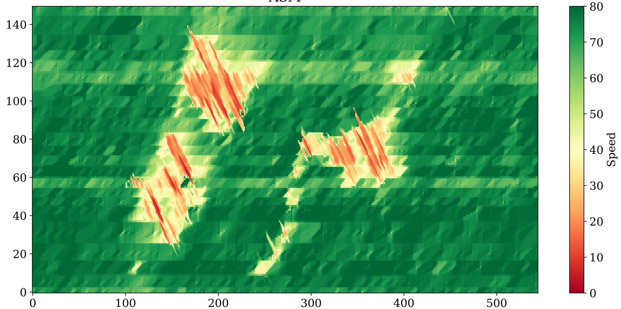
ASM
