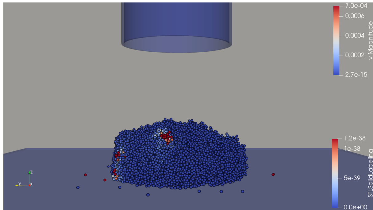
(d) 20k Conical Heap (ParaView)
