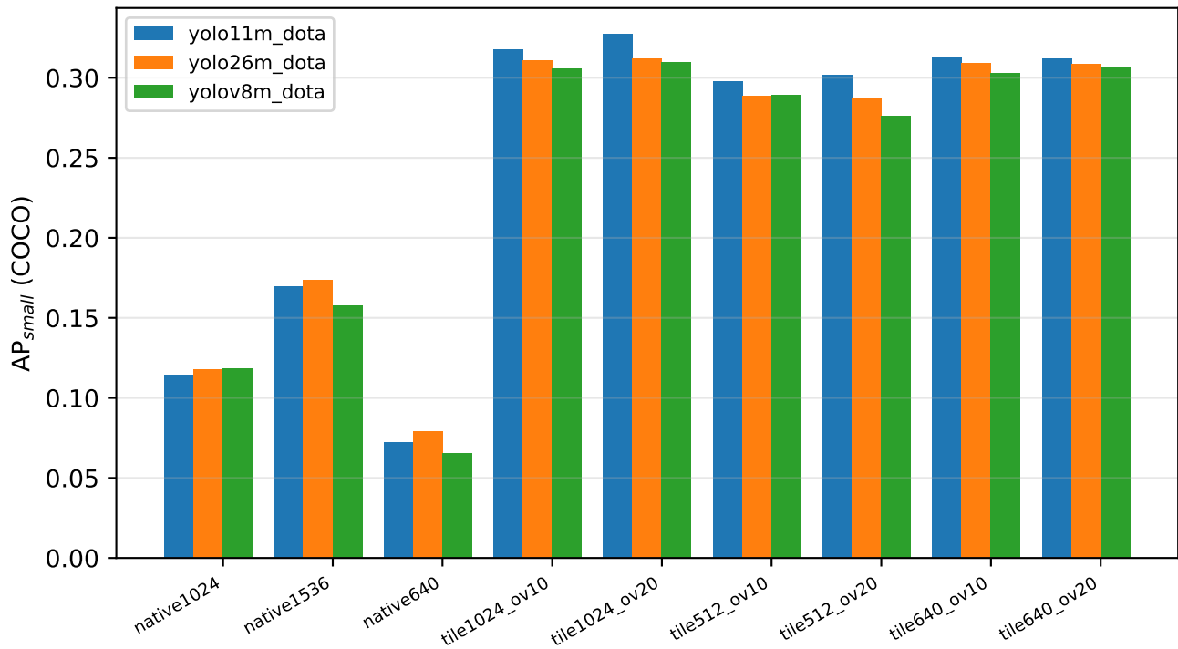
Small-object AP (DOTA)
