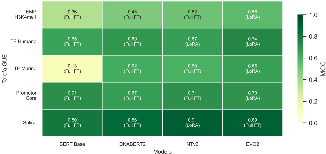
Melhor MCC por Modelo × Tarefa GUE (todas as estratégias)
