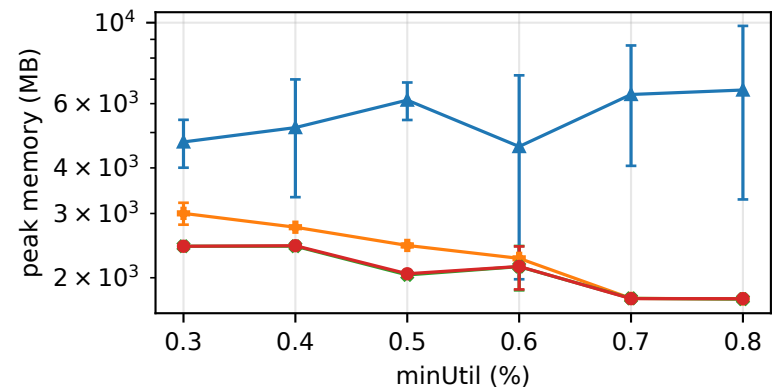
TAFENG
