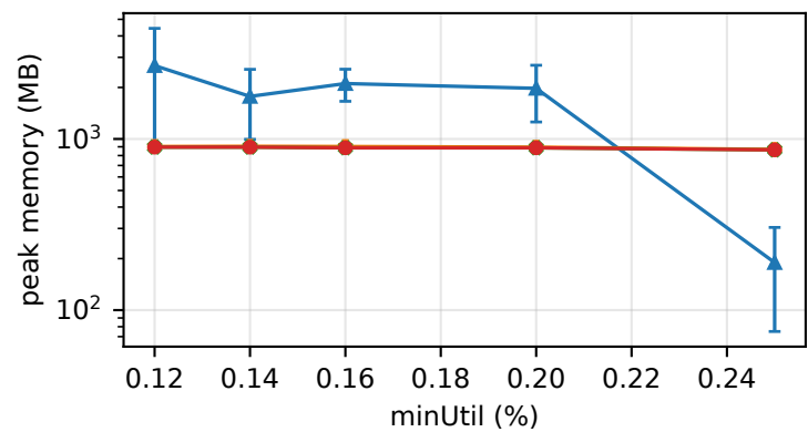
TAFENG
