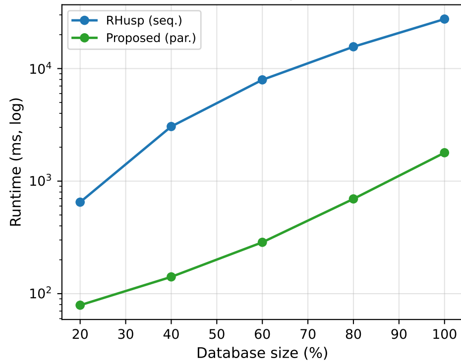
(a) Data scaling — SYN
