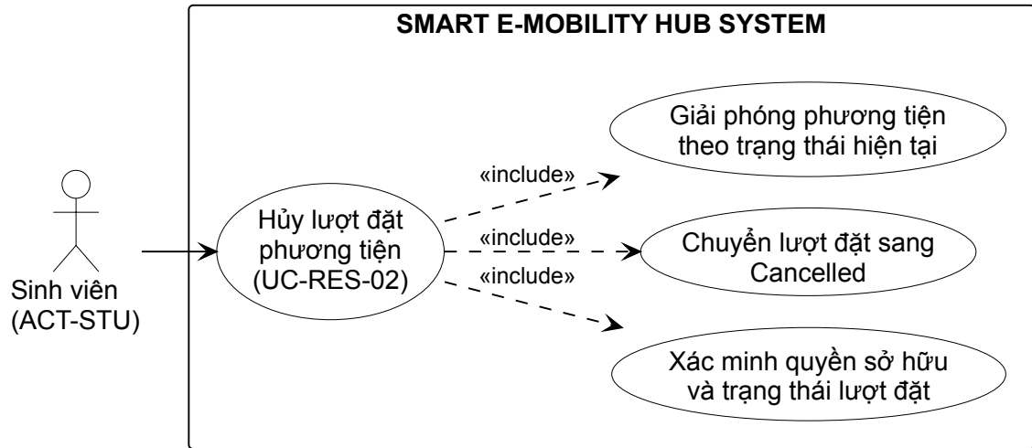
Hình 2: Sơ đồ Use Case UC-RES-02 – Hủy lượt đặt phương tiện
