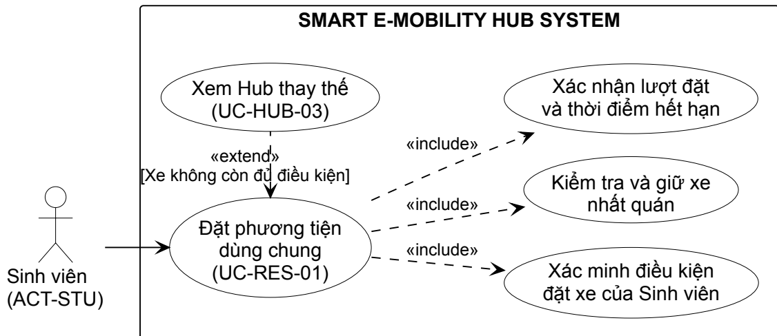
Hình 1: Sơ đồ Use Case UC-RES-01 – Đặt phương tiện dùng chung
