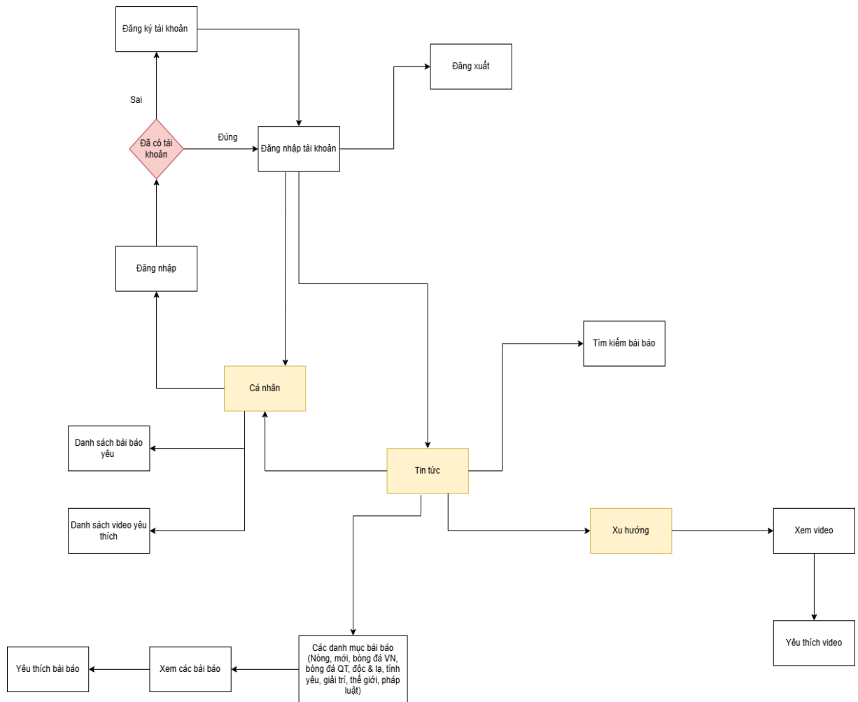
Hình 3.1.2. Điều hướng giữa các màn hình người dùng
