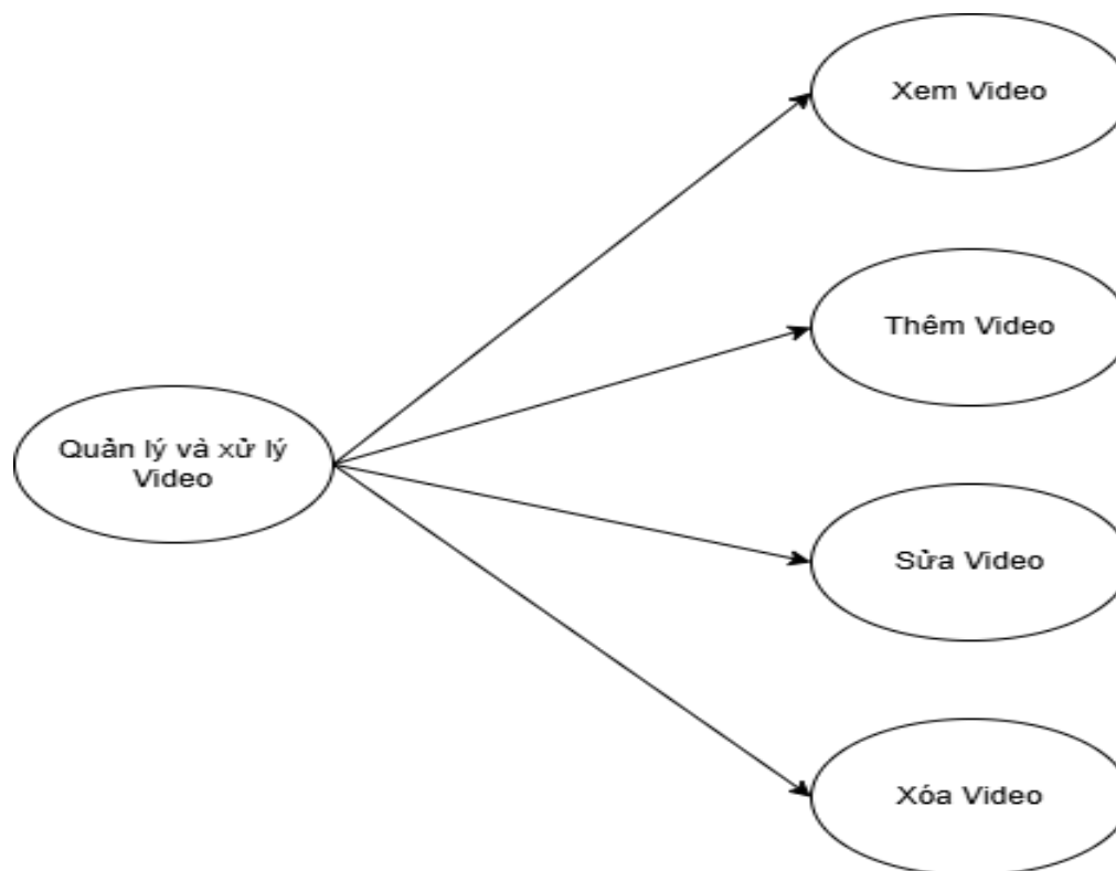
Hình 2.7. Use case quản lý và xử lý video
