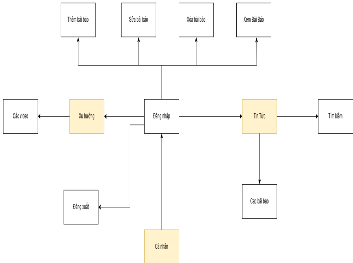
Hình 3.1. Điều hướng giữa các màn hình người quản trị
