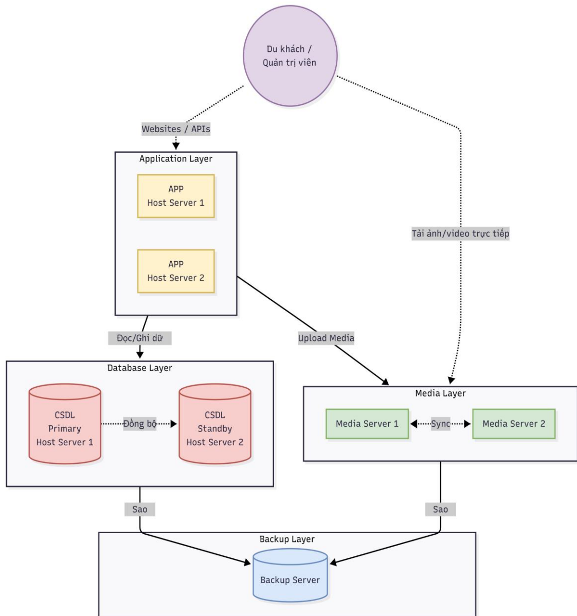
Hình: Mô hình vật lý hệ thống
