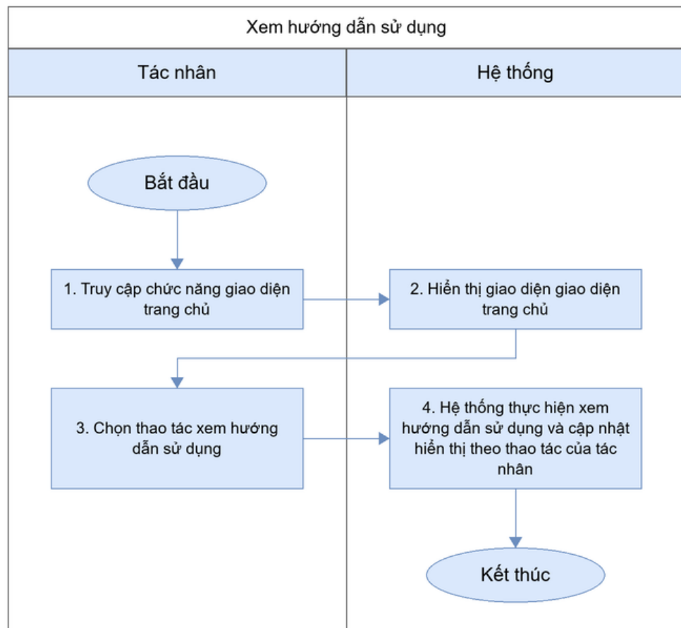
Mô tả dòng sự kiện chính (Basic flow)
