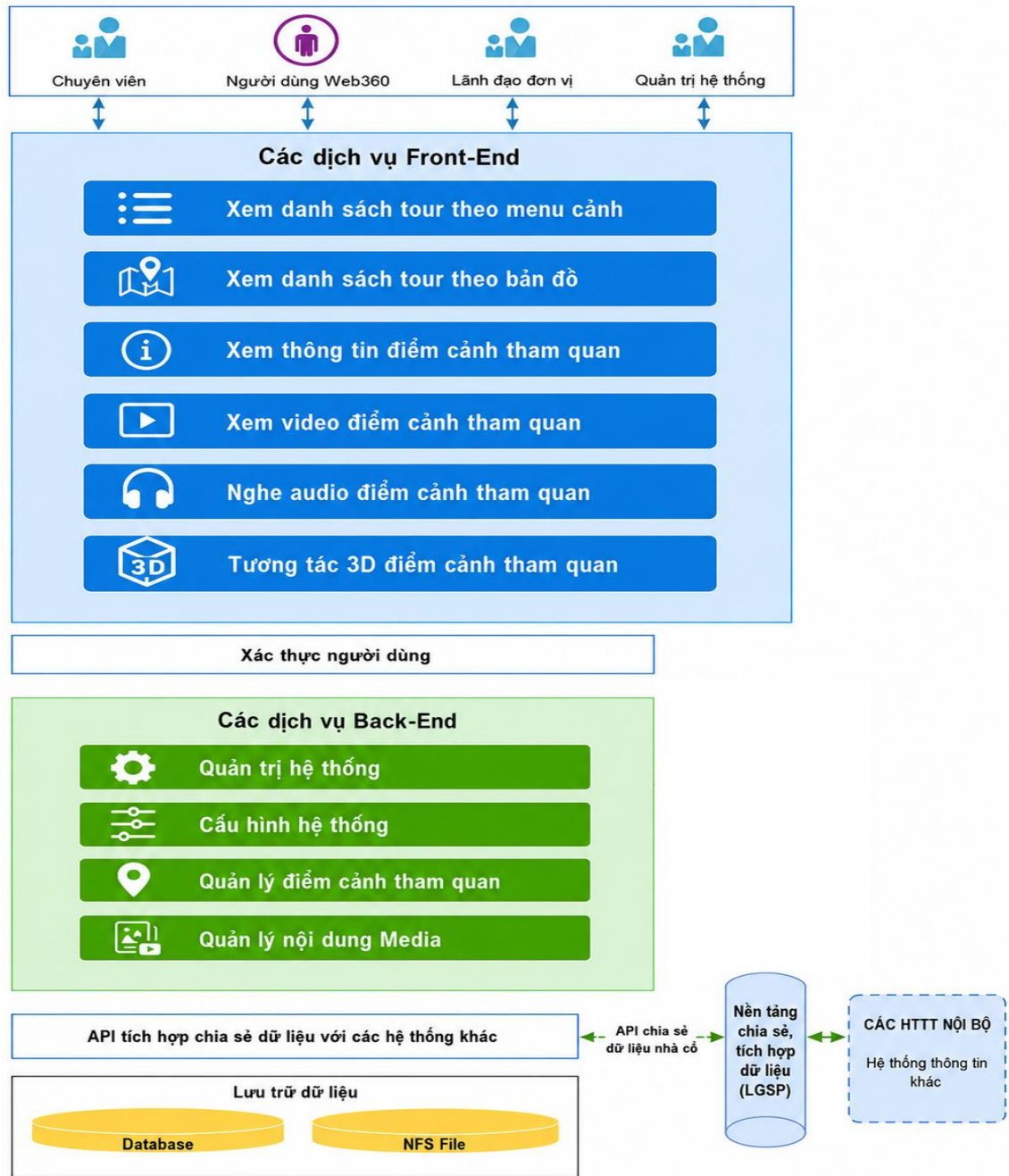
Hình: Mô hình logic hệ thống
