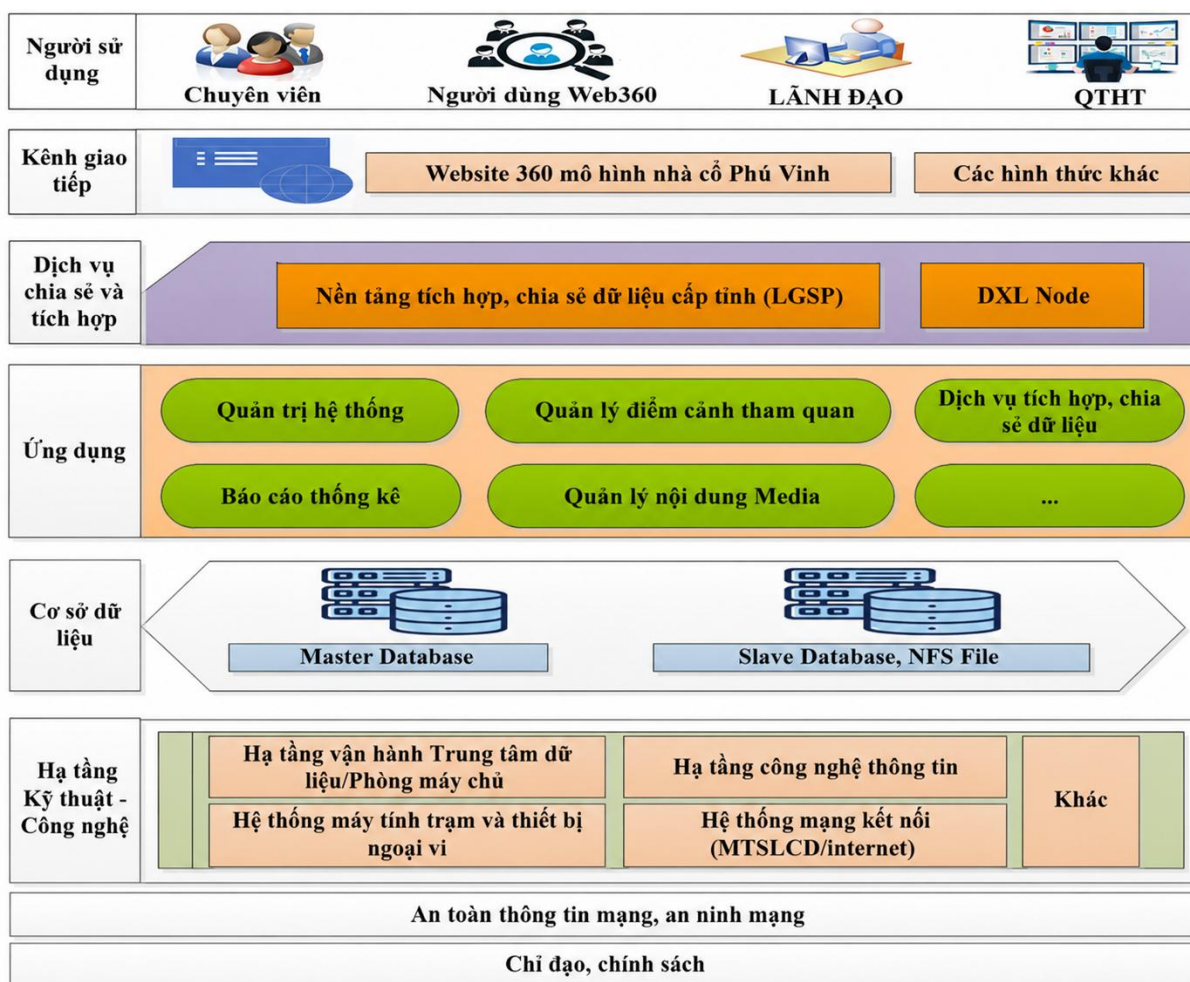
Hình: Mô hình tổng thể hệ thống
