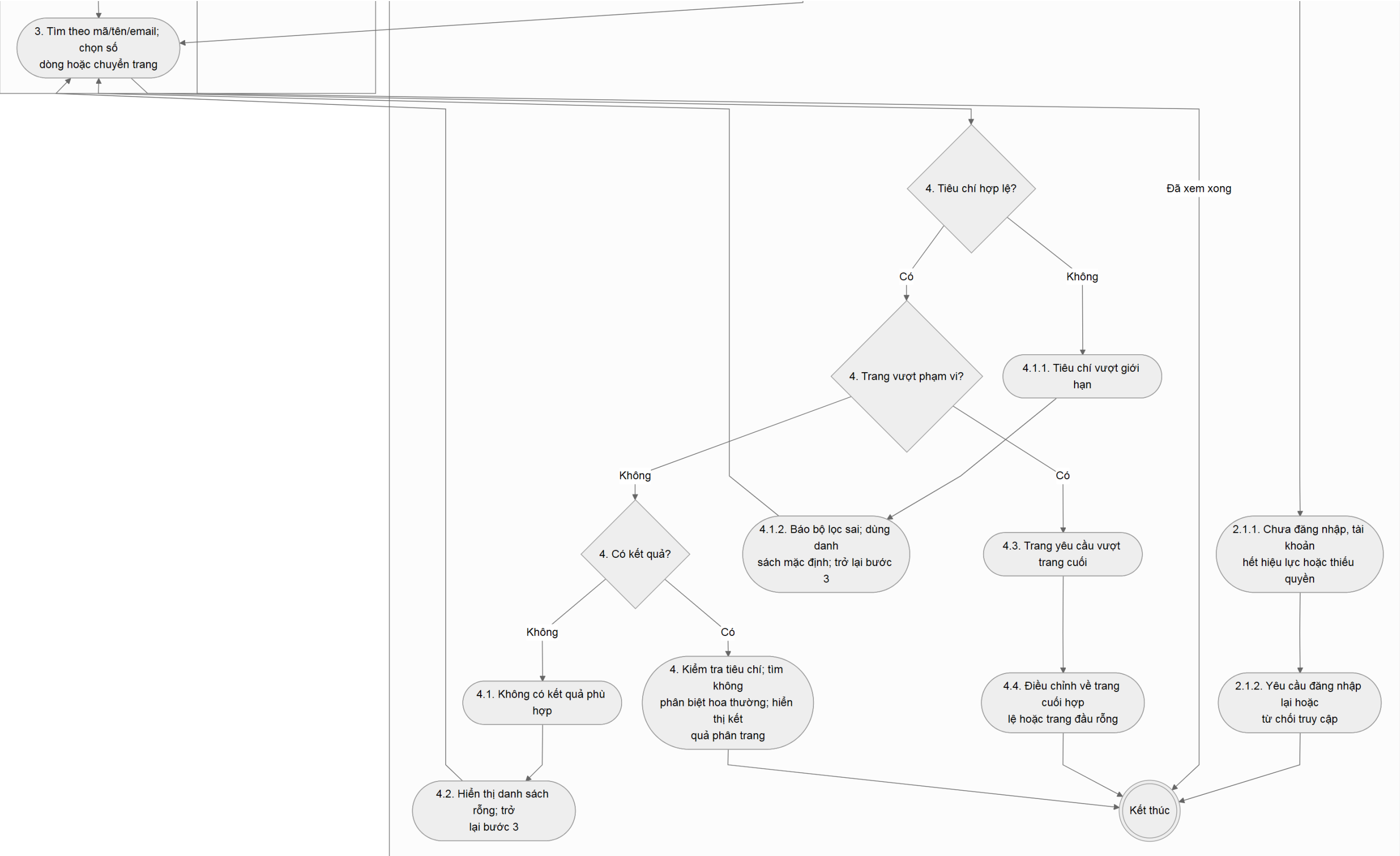
Hình activity-admin-view-users (2/2). Các phần liên nhau có vùng chồng lấp.
