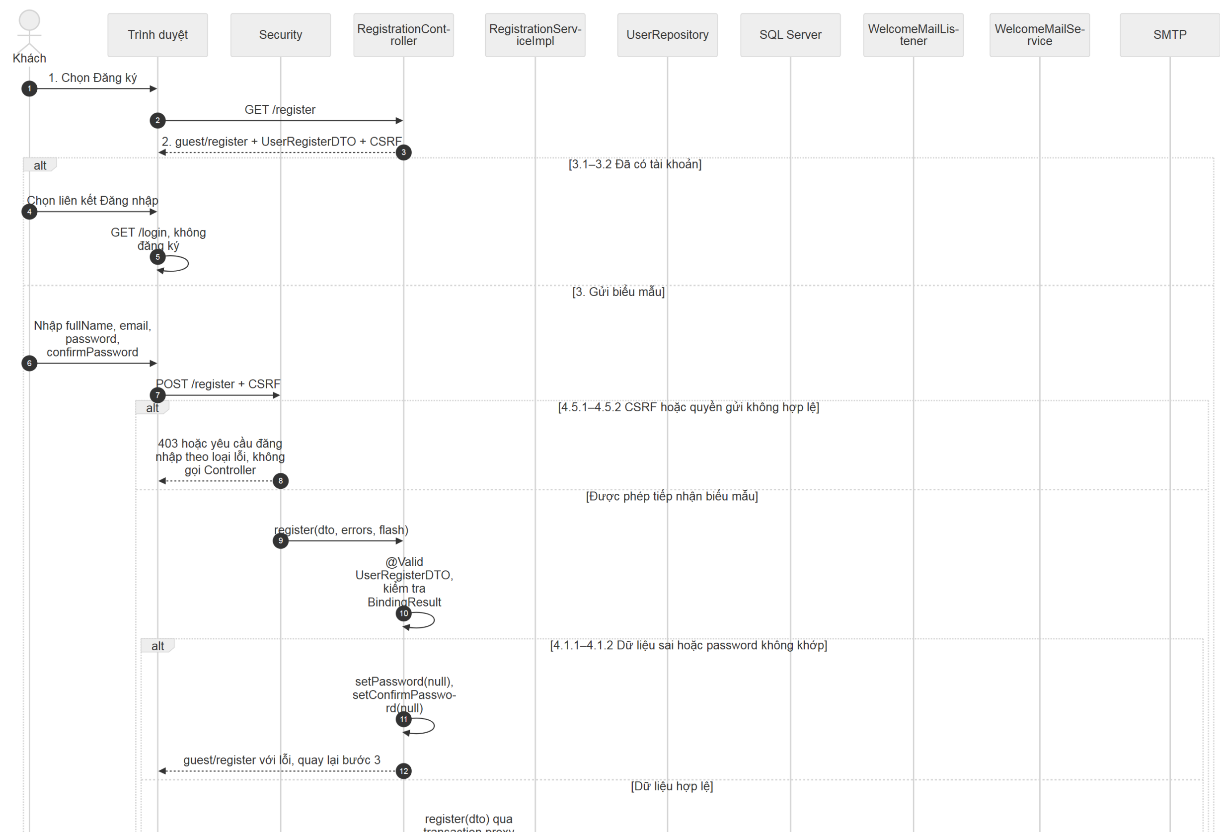
Hình sequence-auth-register (1/4). Các phần liên nhau có vùng chồng lấp.
