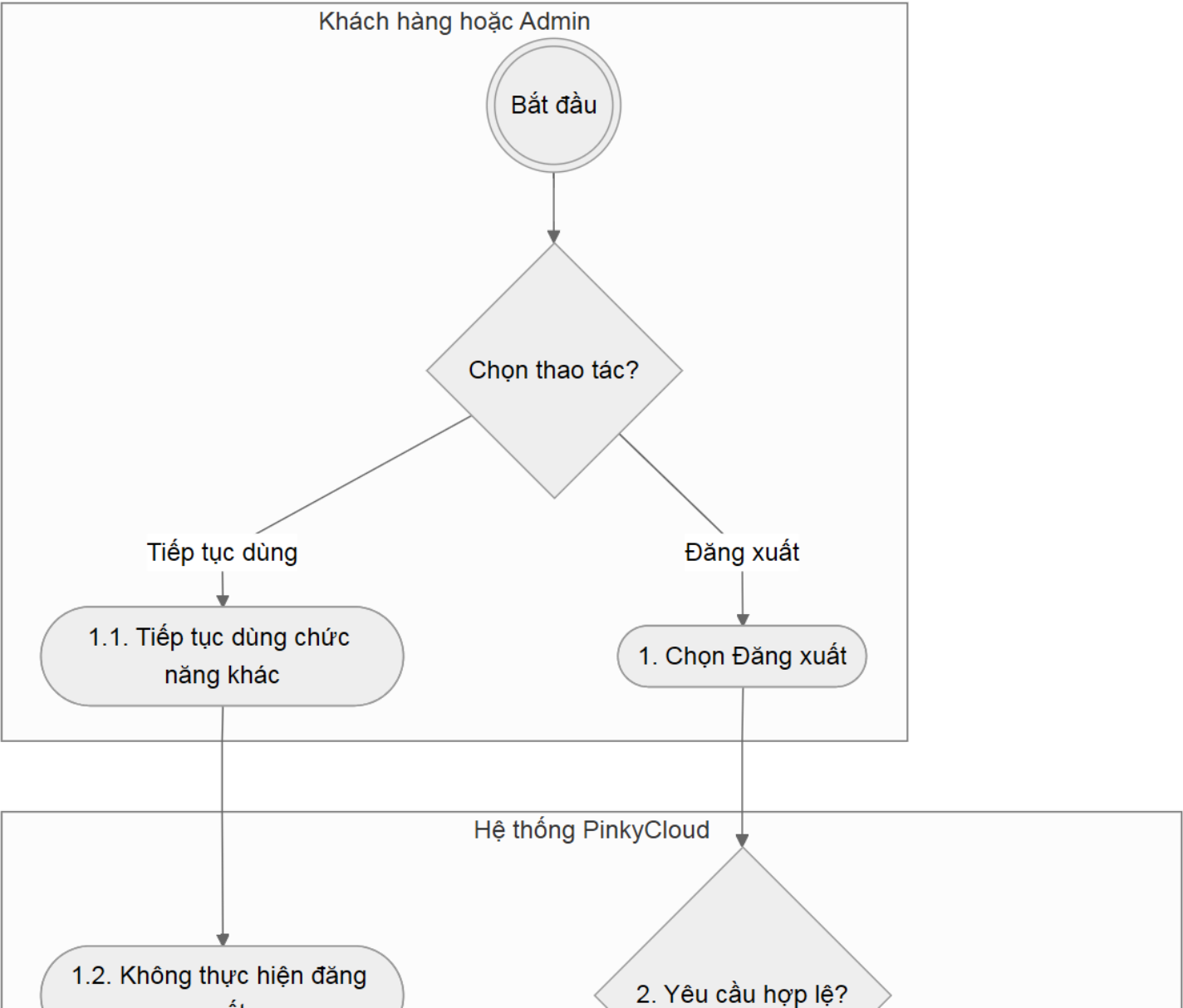
Hình activity-auth-logout (1/2). Các phần liên nhau có vùng chồng lấp.
