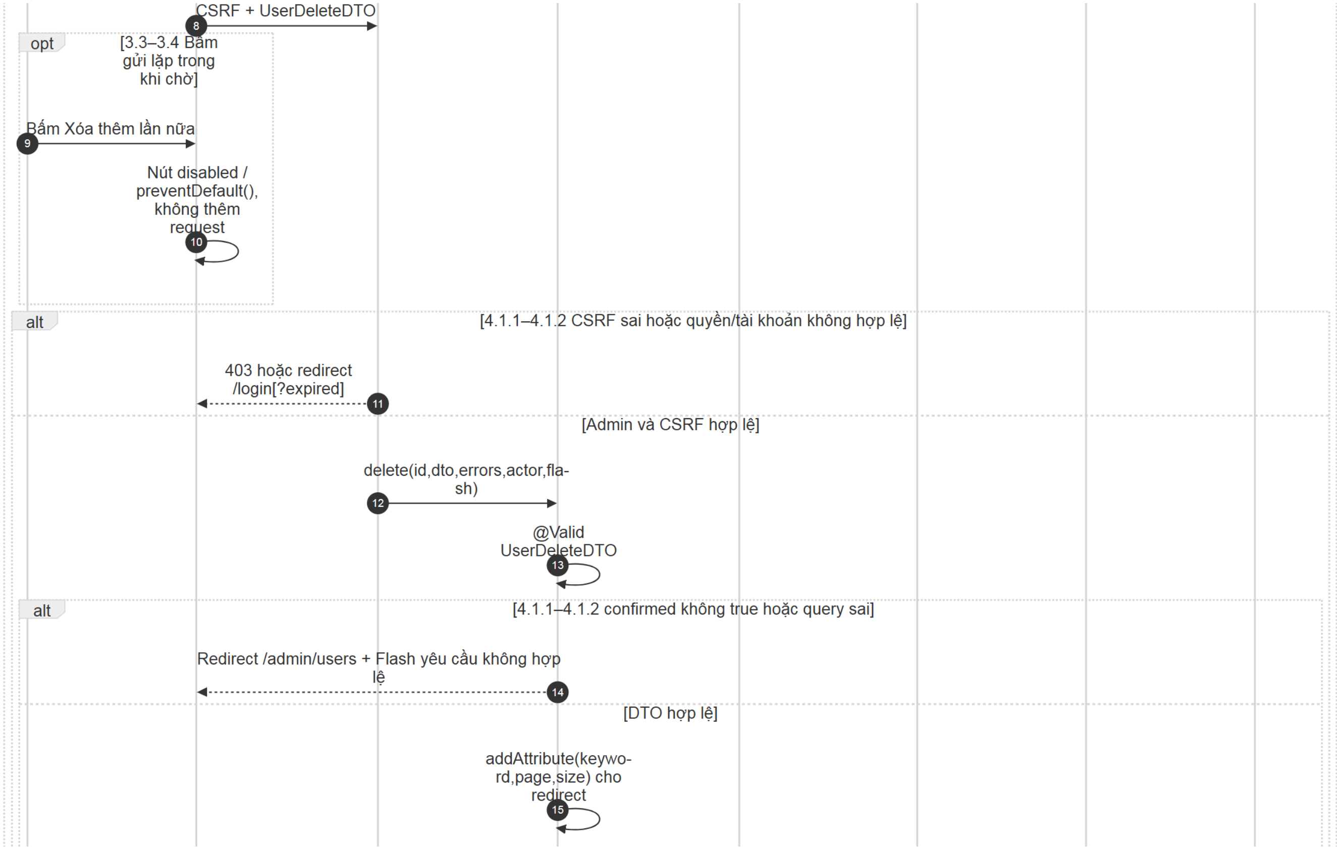
Hình sequence-admin-delete-user (2/6). Các phần liên nhau có vùng chồng lấp.
