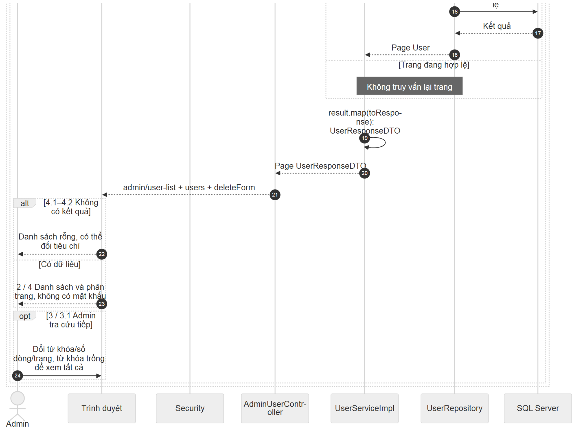
Hình sequence-admin-view-users (3/3). Các phần liên nhau có vùng chồng lấp.
