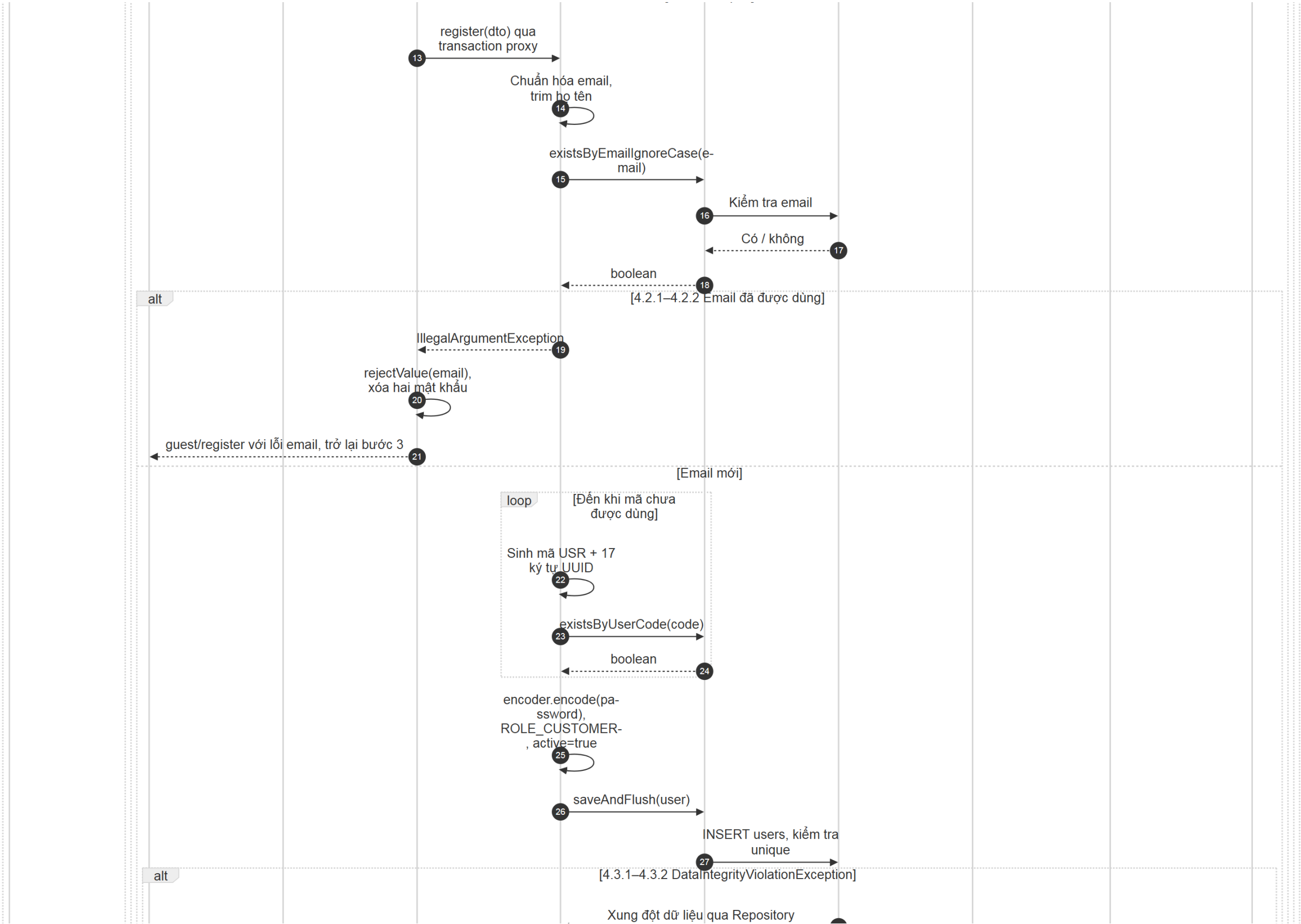
Hình sequence-auth-register (2/4). Các phần liên nhau có vùng chồng lặp.
