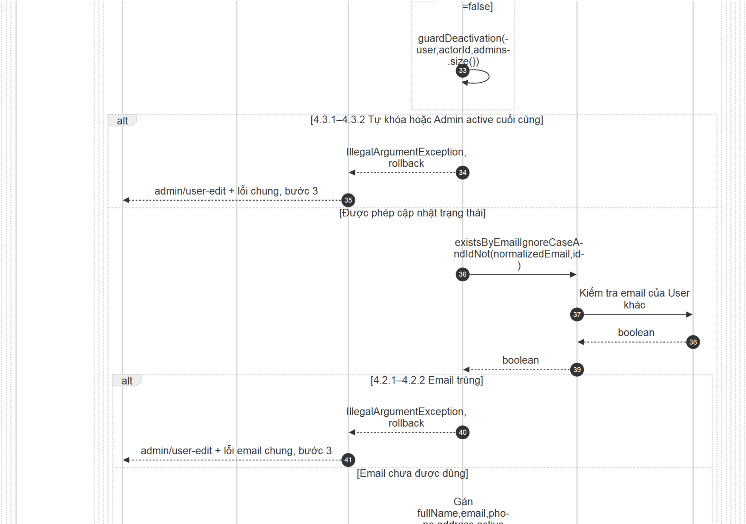
Hình sequence-admin-update-user (4/5). Các phần liên nhau có vùng chồng lấp.
