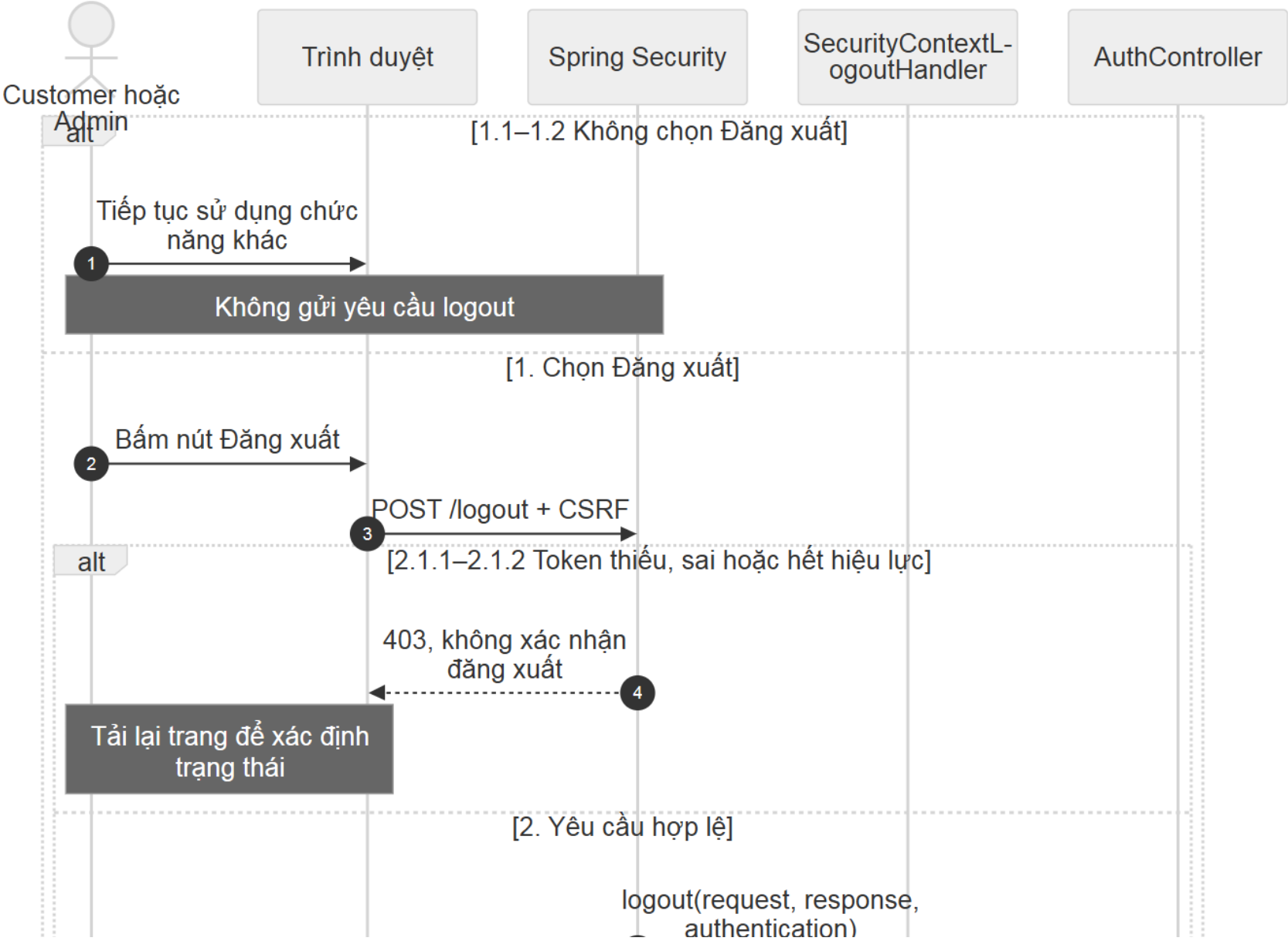
Hình sequence-auth-logout (1/2). Các phần liên nhau có vùng chồng lấp.
