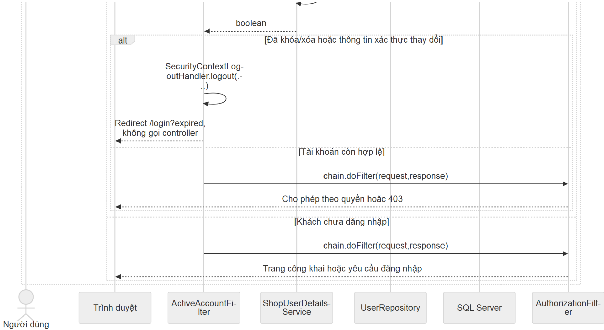
Hình sequence-auth-current-account (2/2). Các phần liên nhau có vùng chồng lấp.
