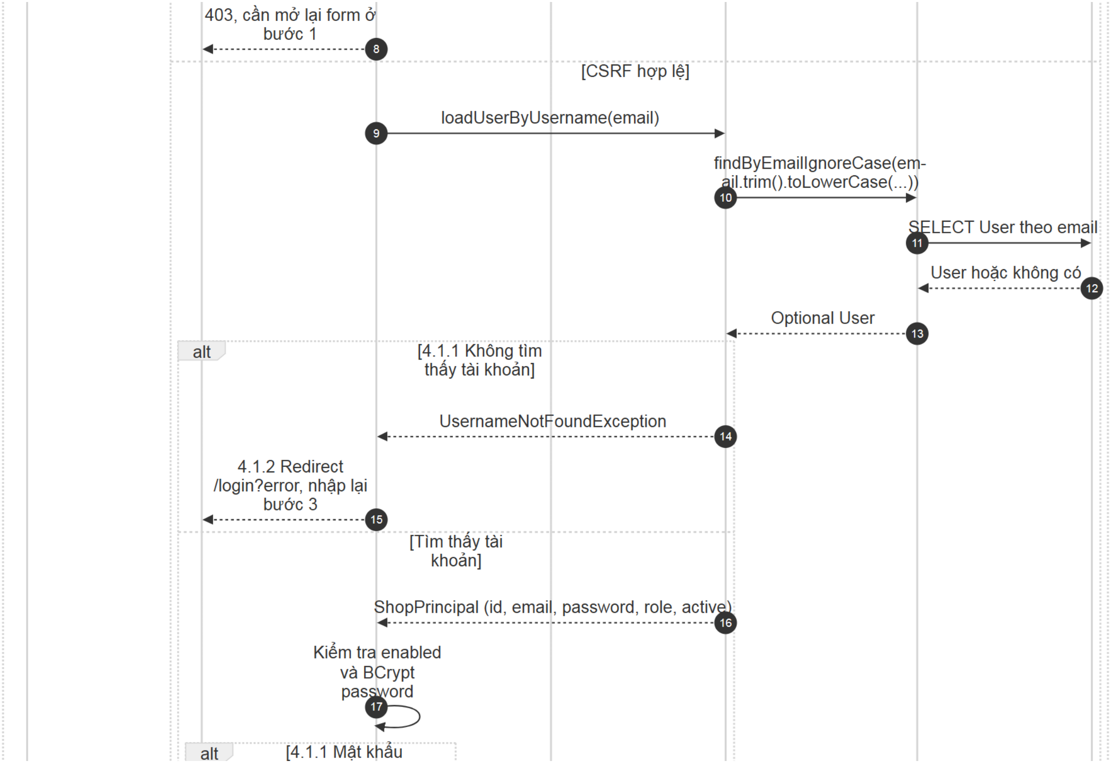
Hình sequence-auth-login (2/3). Các phần liên nhau có vùng chồng lấp.
