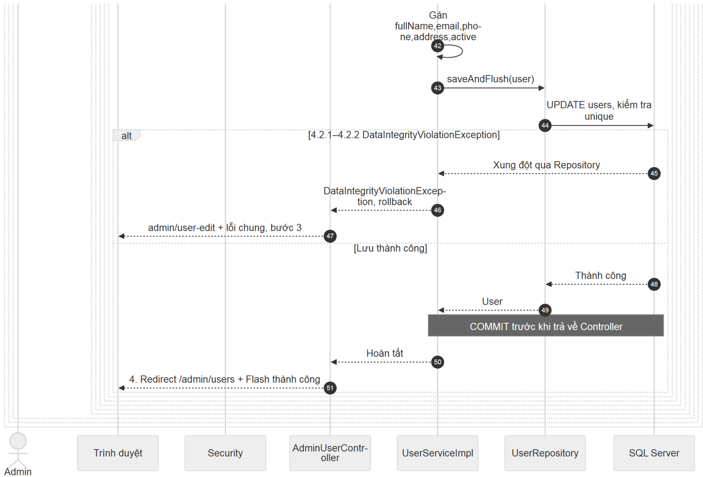
Hình sequence-admin-update-user (5/5). Các phần liền nhau có vùng chồng lấp.
