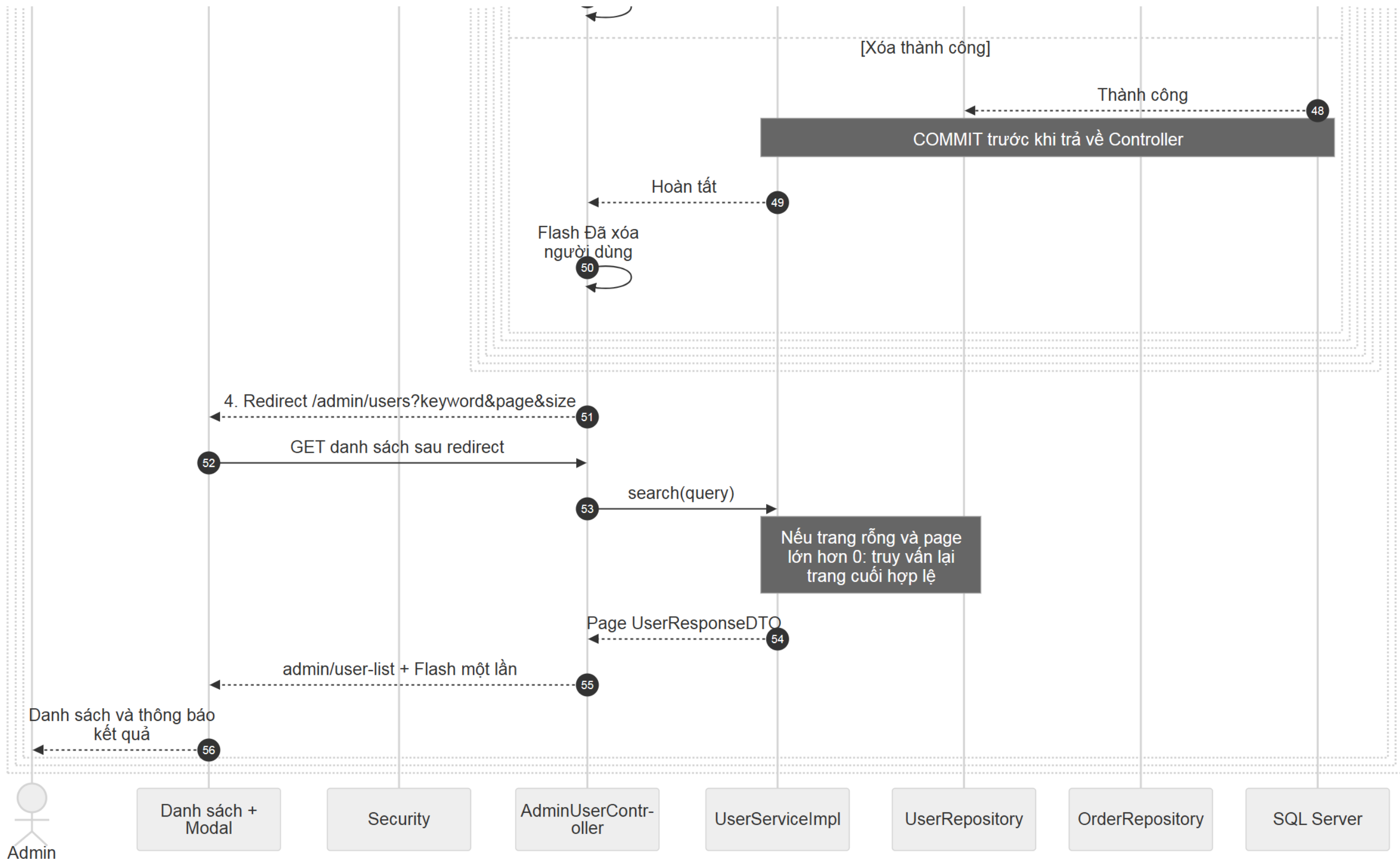
Hình sequence-admin-delete-user (6/6). Các phần liên nhau có vùng chồng lấp.
