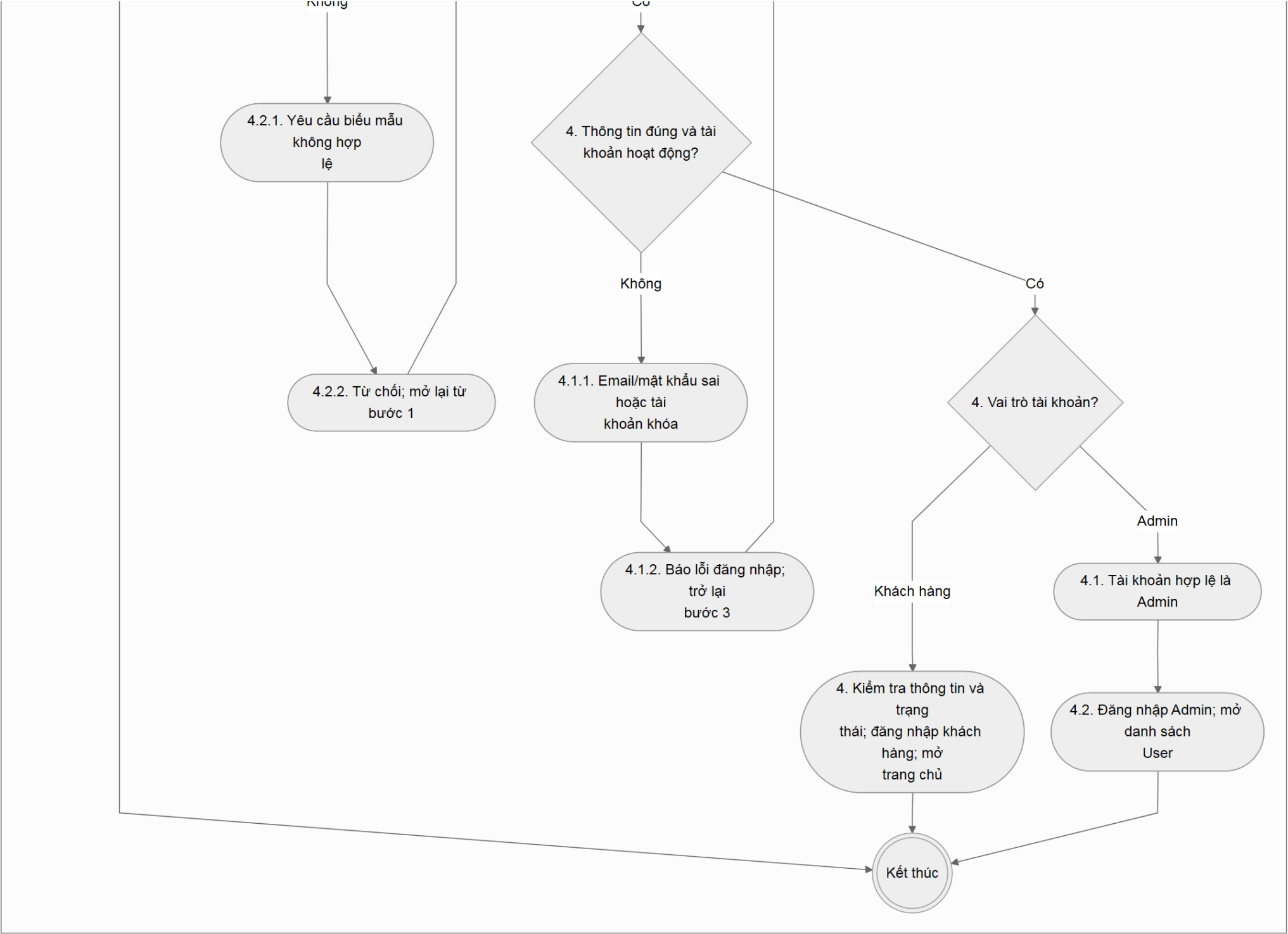
Hình activity-auth-login (2/2). Các phần liên nhau có vùng chồng lấp.
