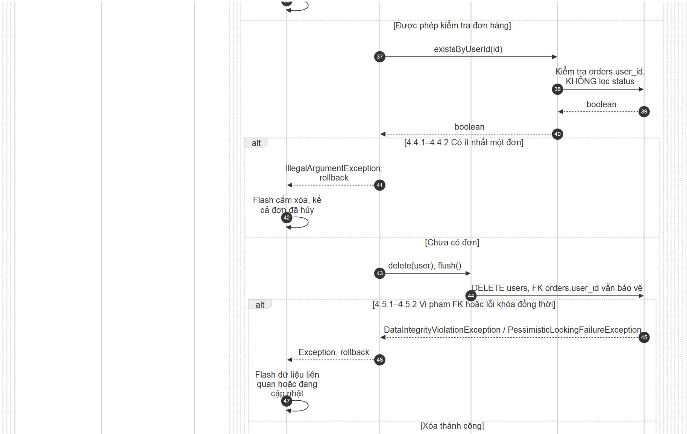
Hình sequence-admin-delete-user (5/6). Các phần liên nhau có vùng chồng lấp.
