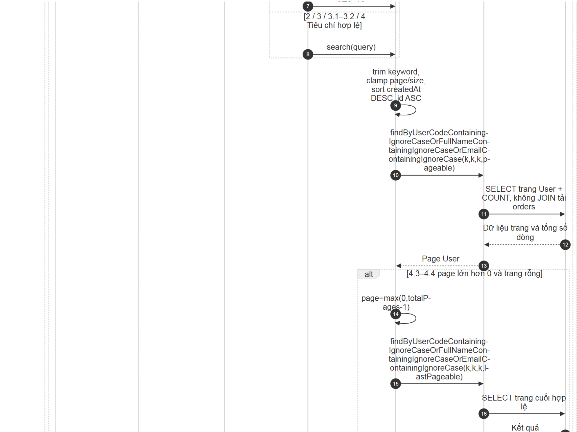
Hình sequence-admin-view-users (2/3). Các phần liên nhau có vùng chồng lấp.
