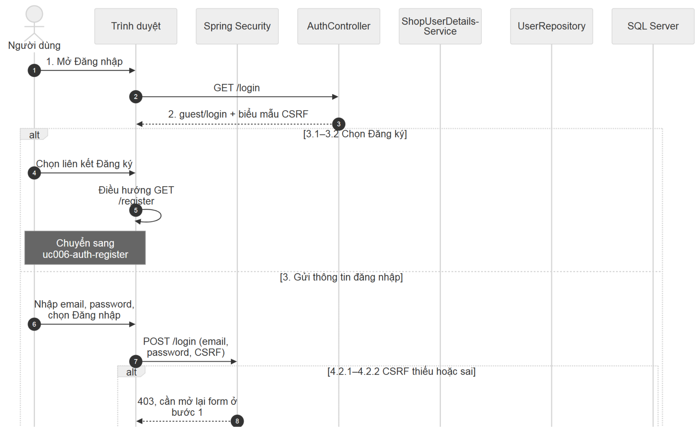
Hình sequence-auth-login (1/3). Các phần liên nhau có vùng chồng lấp.
