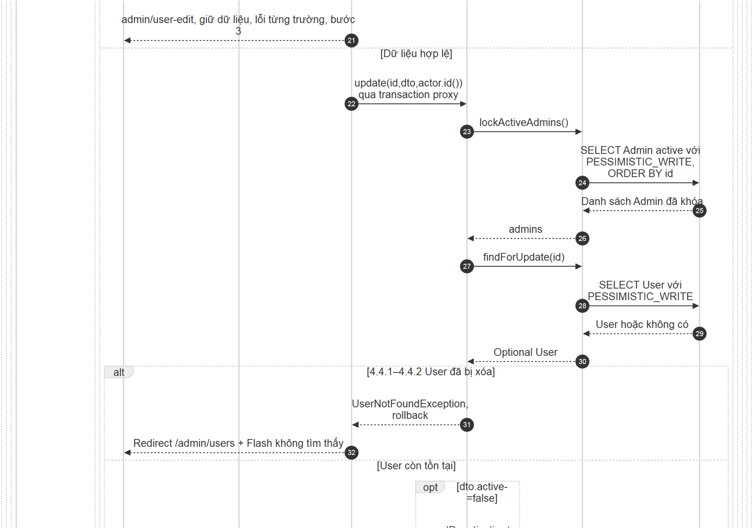
Hình sequence-admin-update-user (3/5). Các phần liên nhau có vùng chồng lấp.
