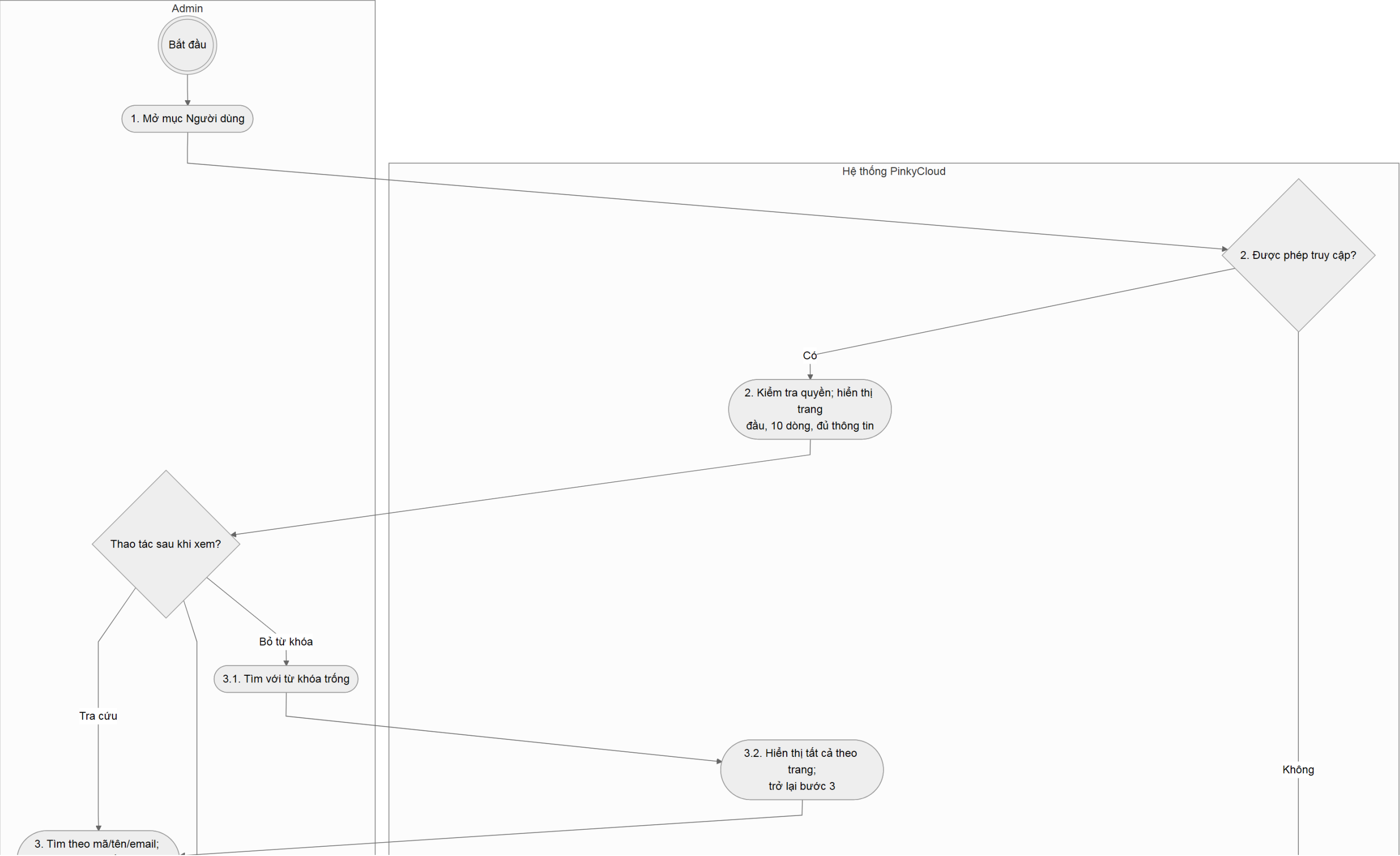
Hình activity-admin-view-users (1/2). Các phần liên nhau có vùng chồng lấp.
