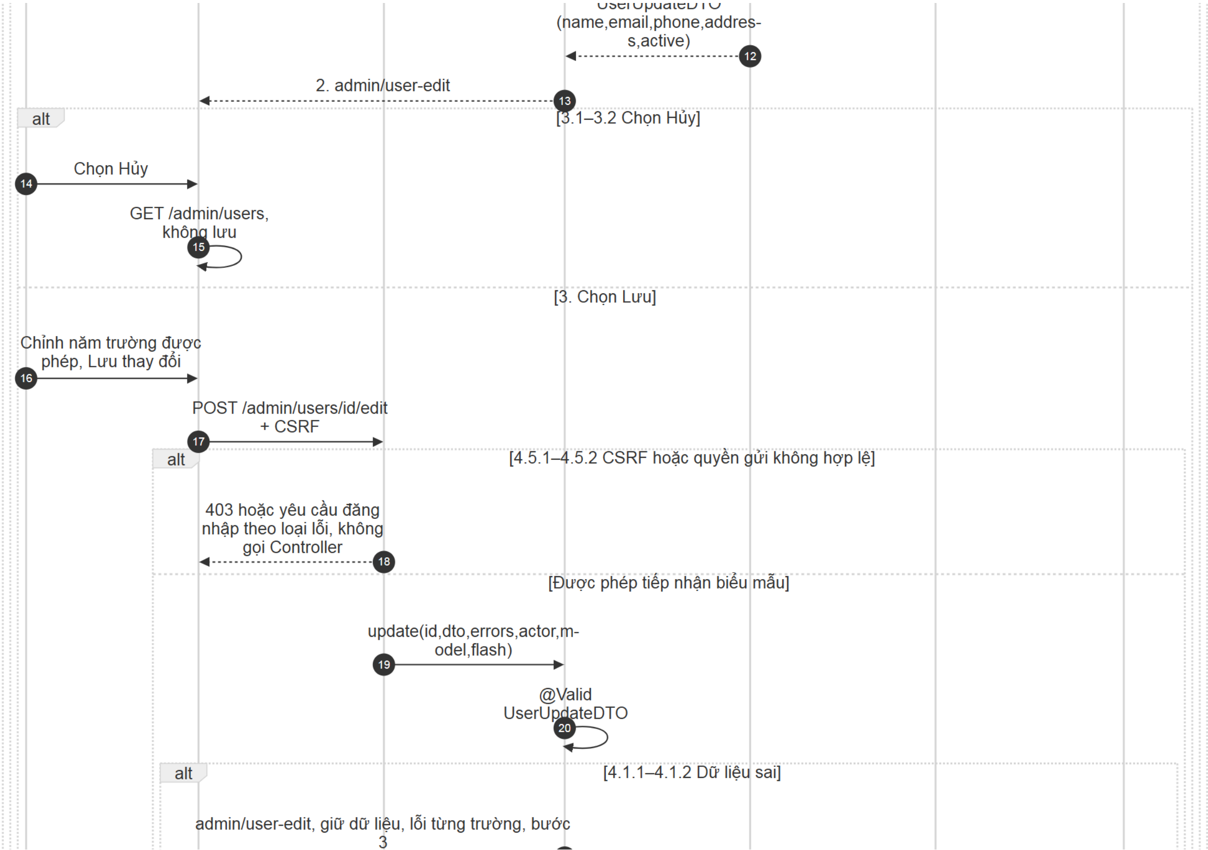
Hình sequence-admin-update-user (2/5). Các phần liên nhau có vùng chồng lấp.
