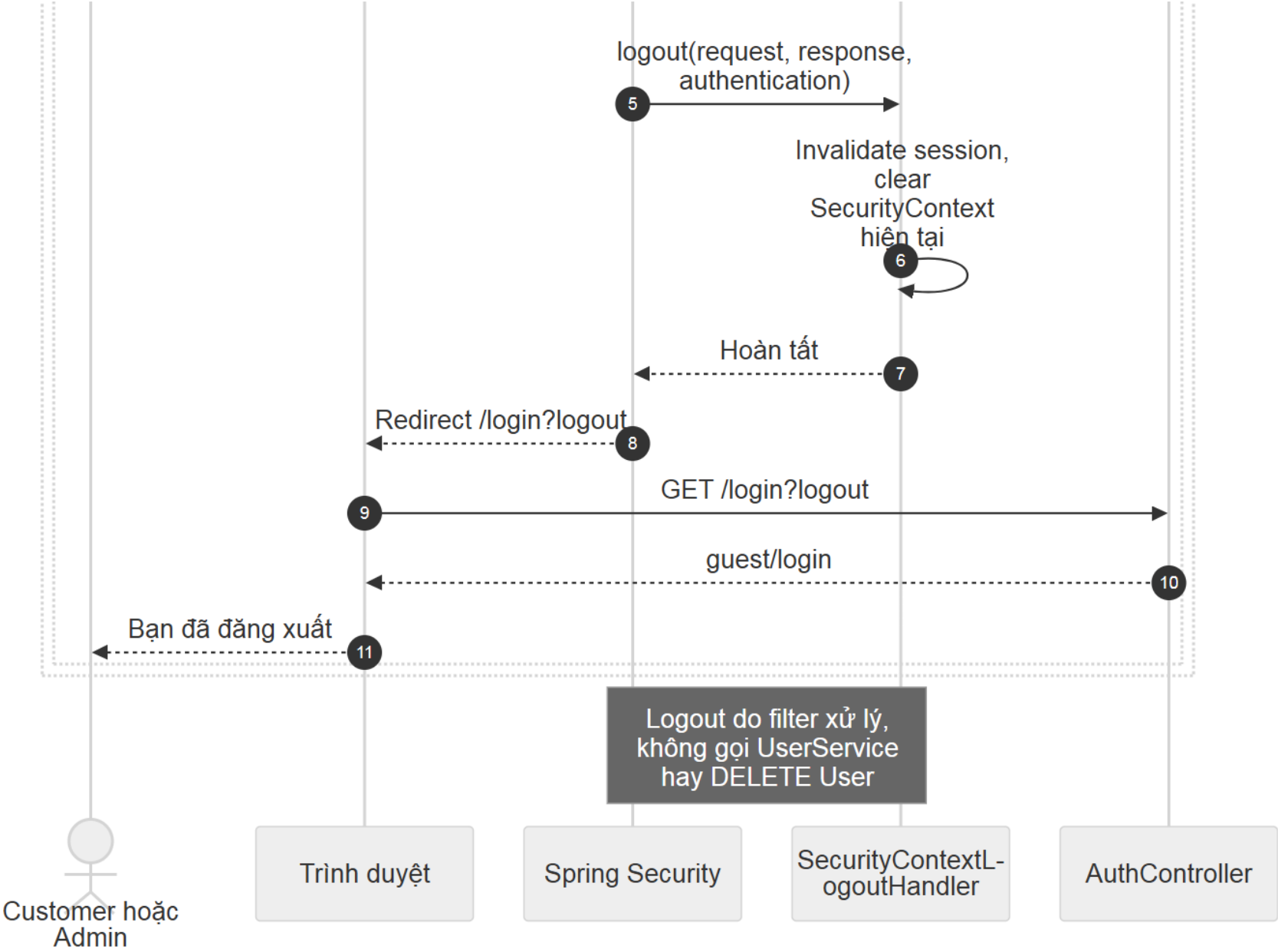
Hình sequence-auth-logout (2/2). Các phần liên nhau có vùng chồng lấp.
