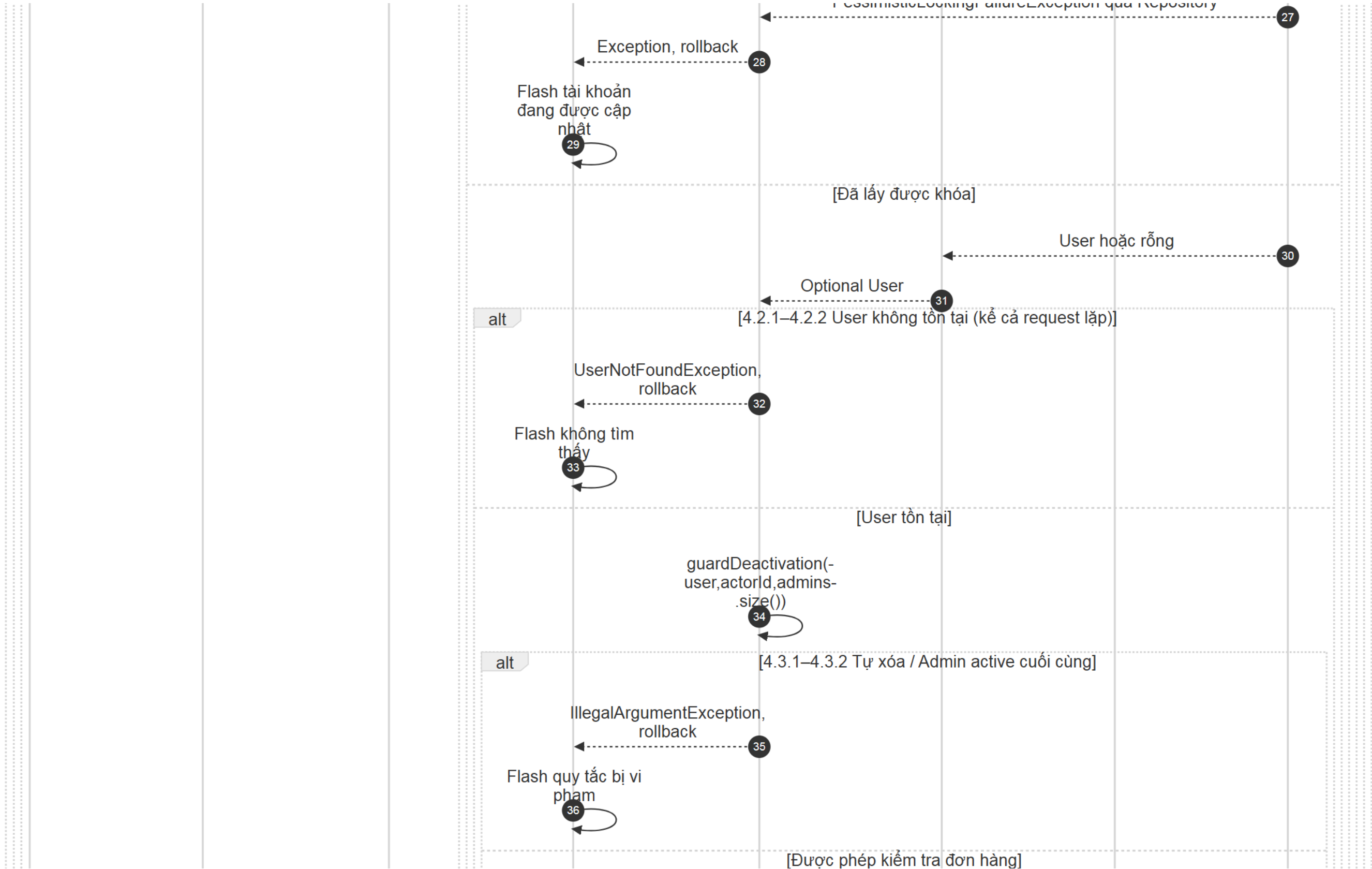
Hình sequence-admin-delete-user (4/6). Các phần liên nhau có vùng chồng lấp.
