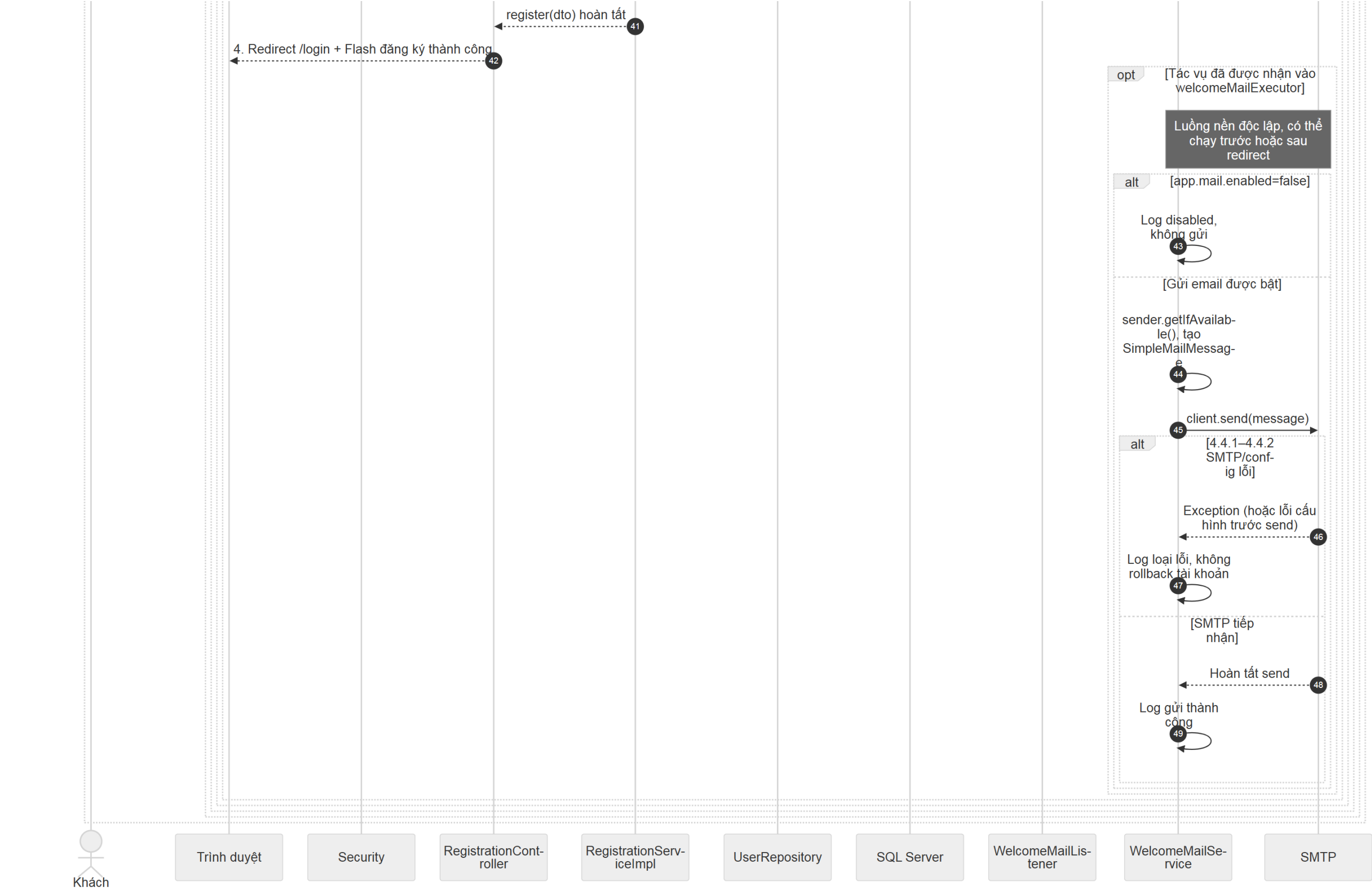
Hình sequence-auth-register (4/4). Các phần liên nhau có vùng chồng lặp.
