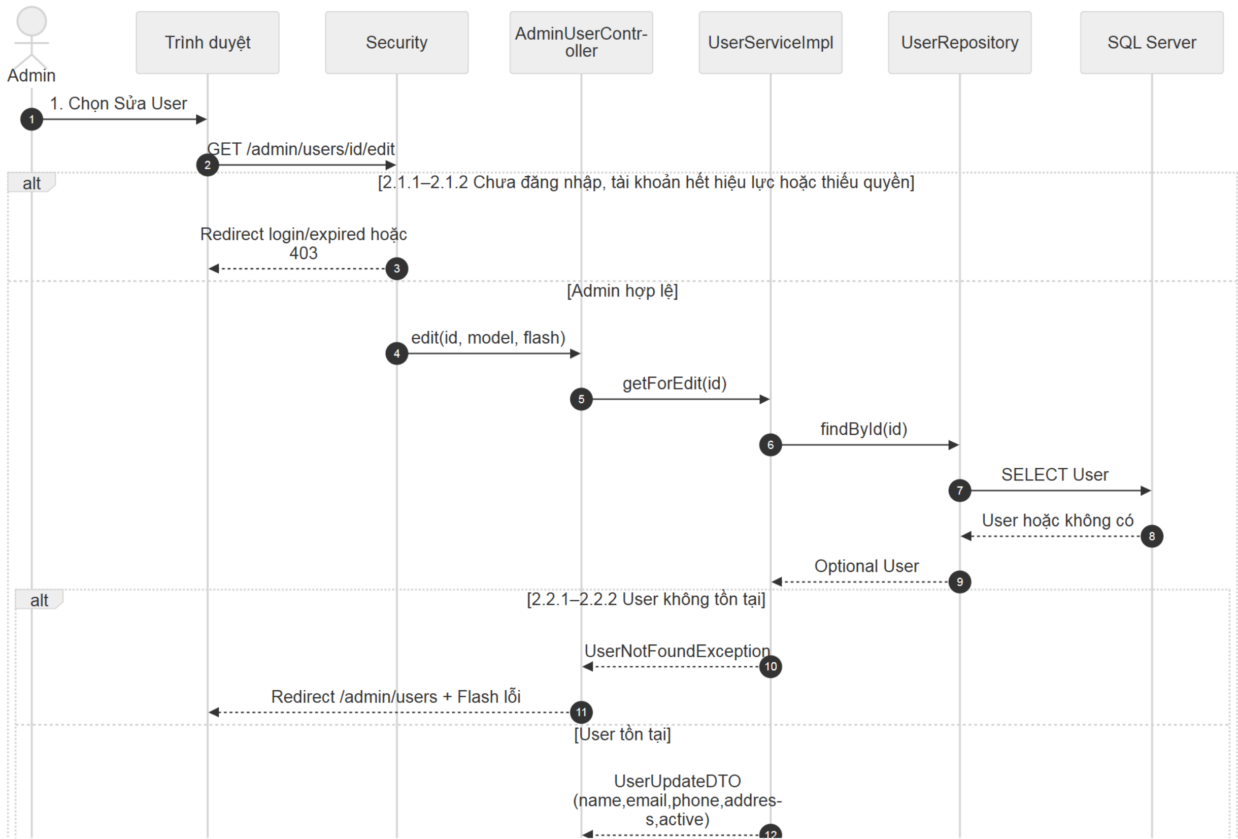
Hình sequence-admin-update-user (1/5). Các phần liên nhau có vùng chồng lấp.
