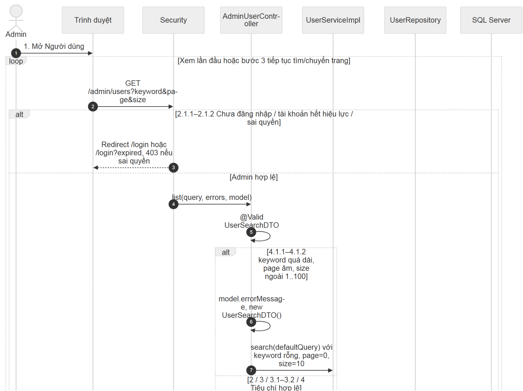
Hình sequence-admin-view-users (1/3). Các phần liên nhau có vùng chồng lấp.
