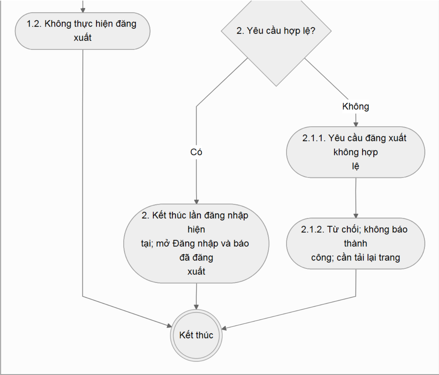
Hình activity-auth-logout (2/2). Các phần liên nhau có vùng chồng lấp.
