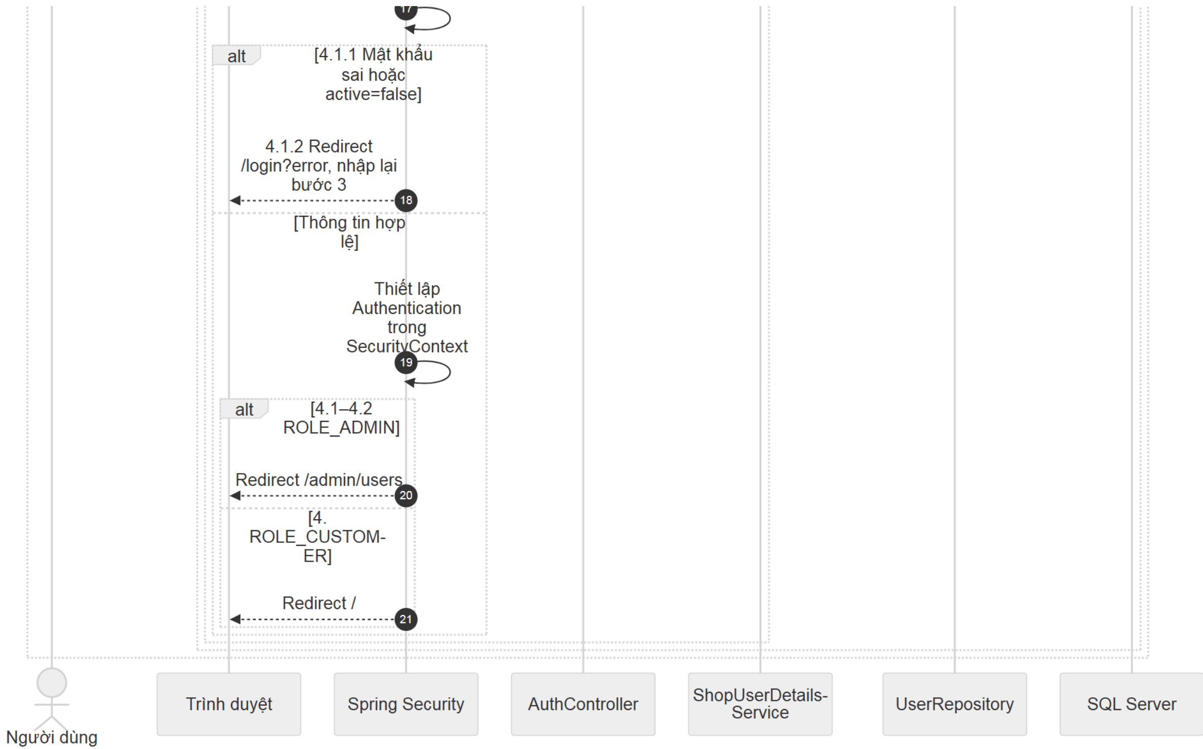
Hình sequence-auth-login (3/3). Các phần liên nhau có vùng chồng lấp.
