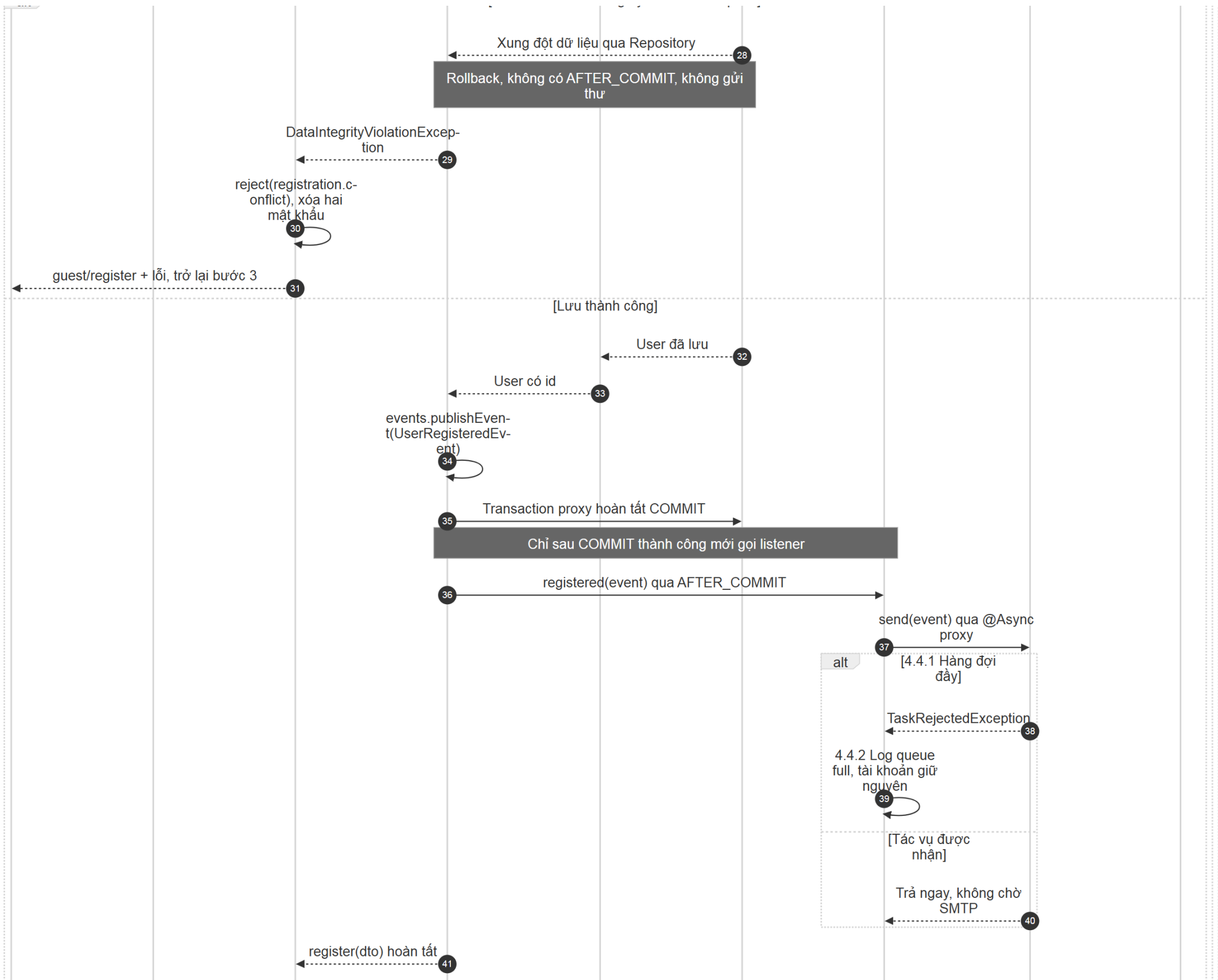
Hình sequence-auth-register (3/4). Các phần liền nhau có vùng chồng lặp.
