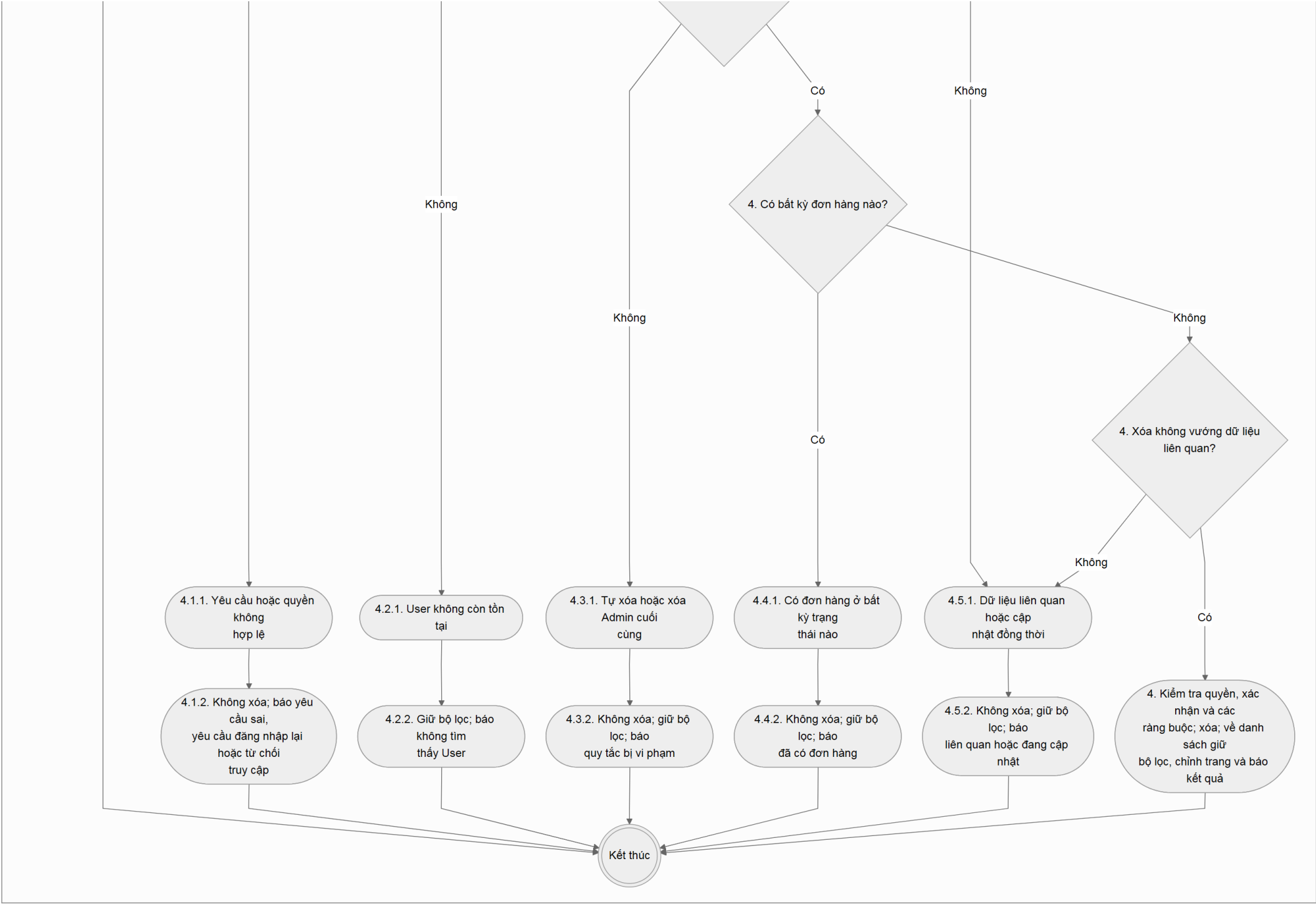
Hình activity-admin-delete-user (3/3). Các phần liên nhau có vùng chồng lấp.
