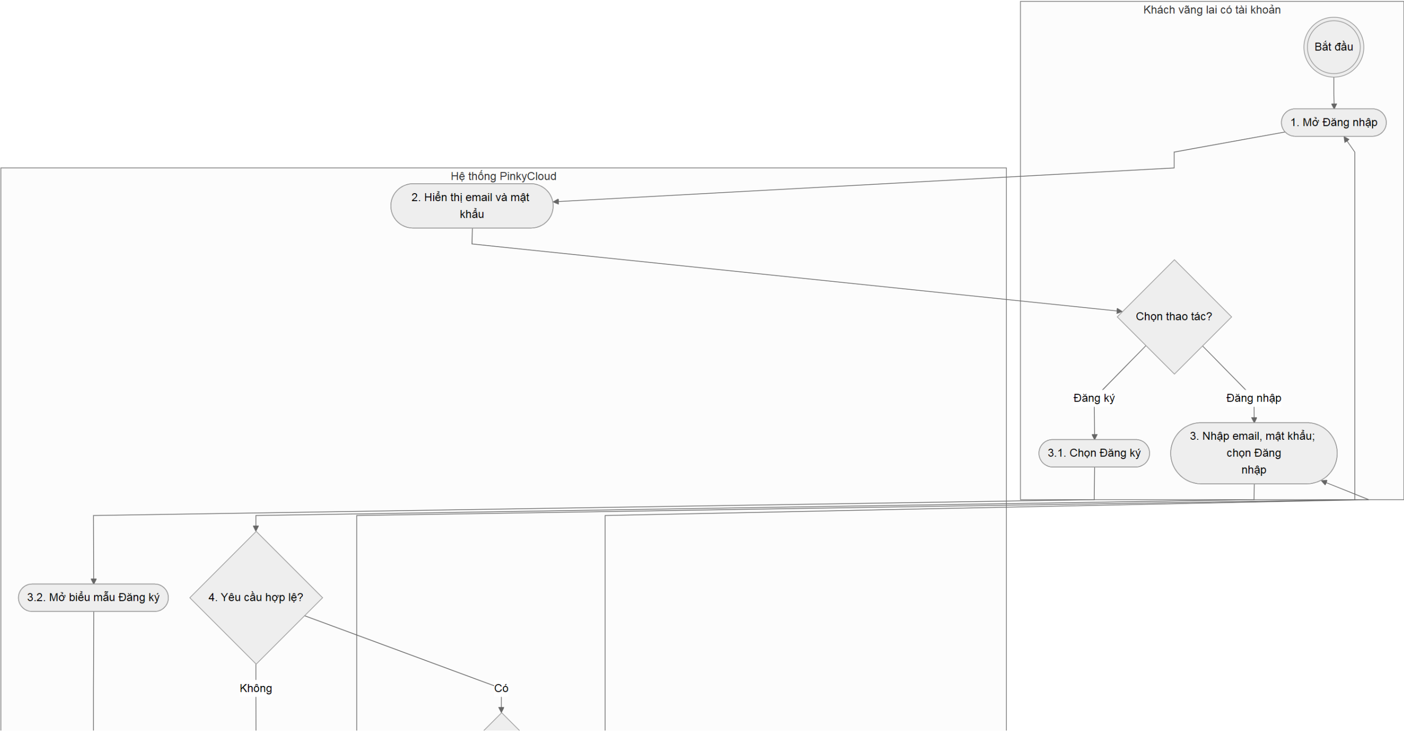
Hình activity-auth-login (1/2). Các phần liên nhau có vùng chồng lấp.
