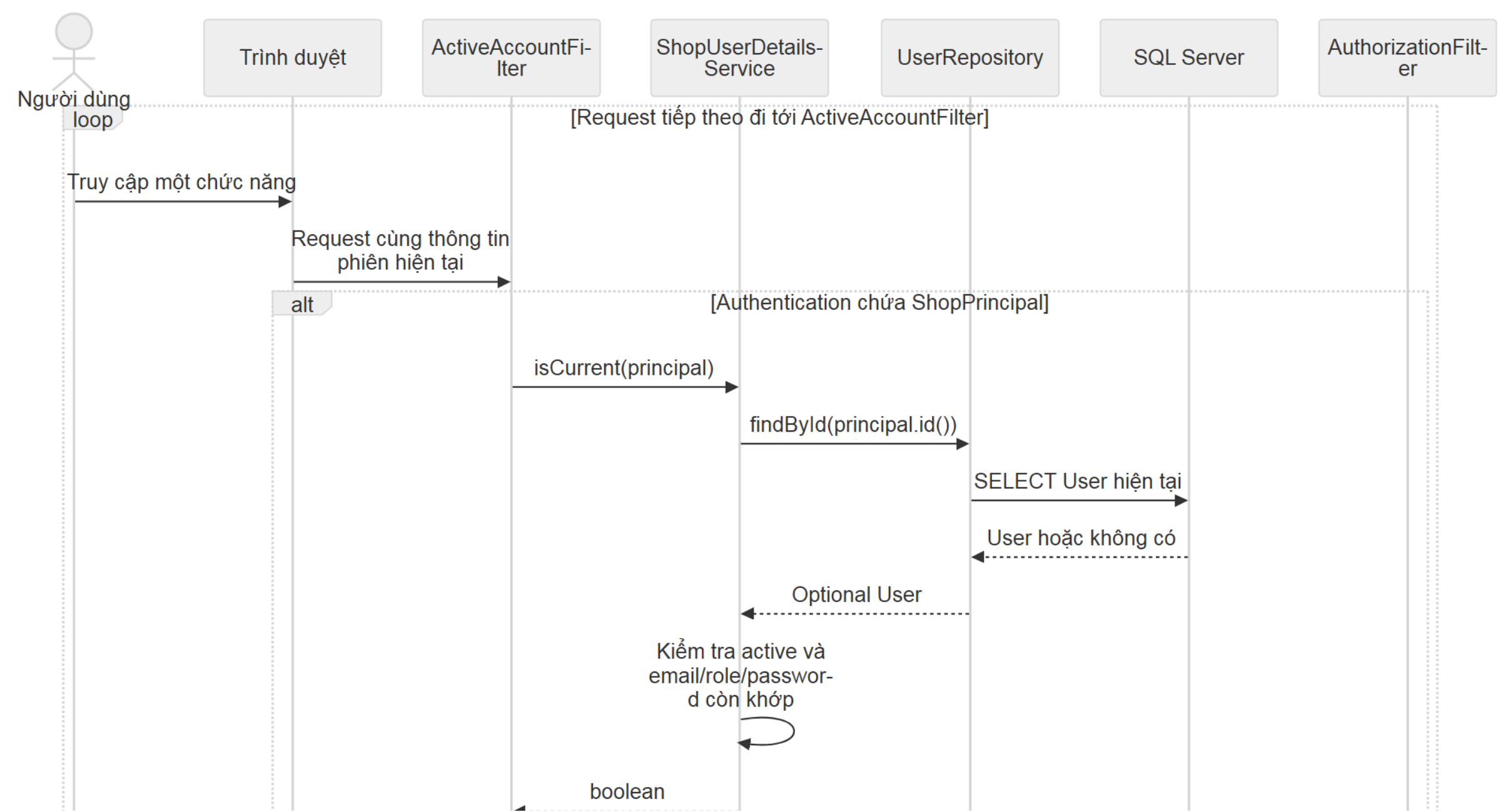
Hình sequence-auth-current-account (1/2). Các phần liên nhau có vùng chồng lấp.
