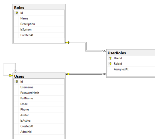
Hình 3.4 Mối quan hệ giữa User - Role
