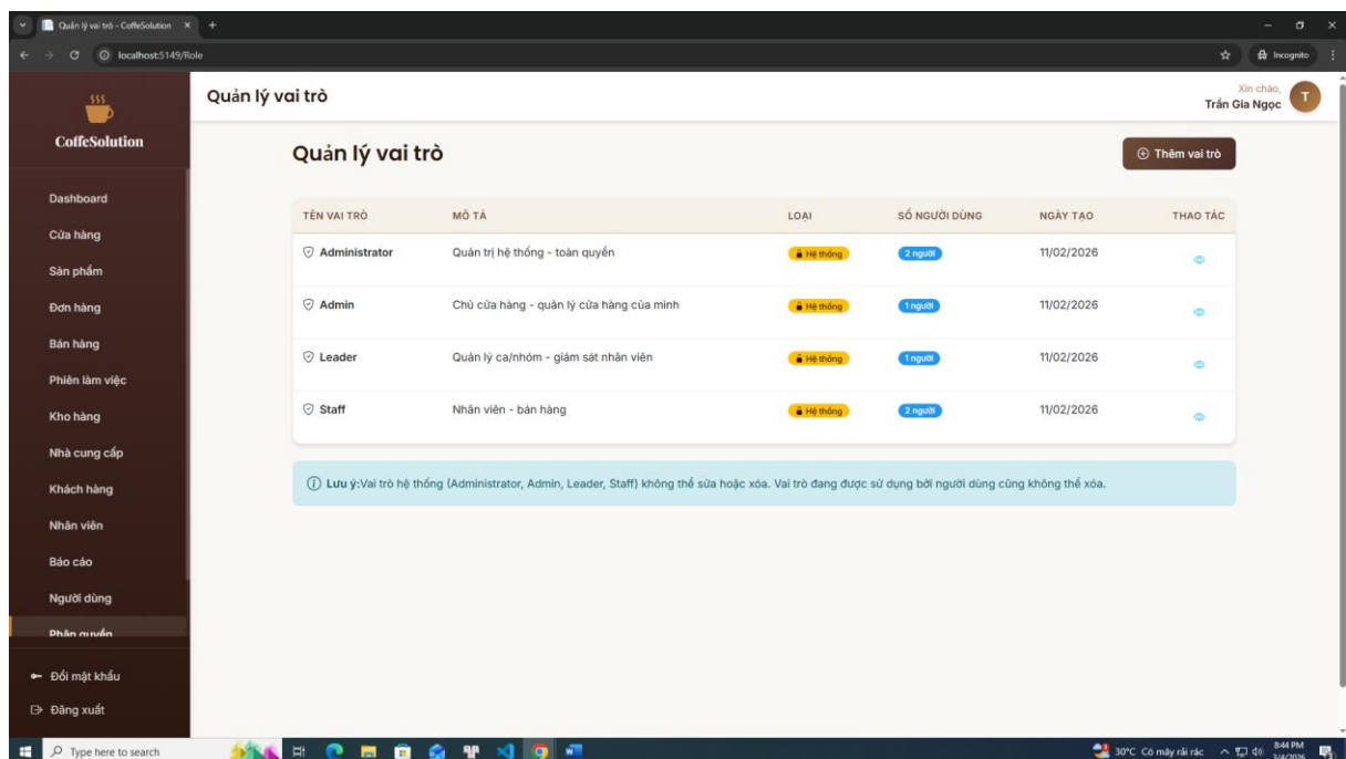
Hình 4.18 Giao diện quản lý vai trò
