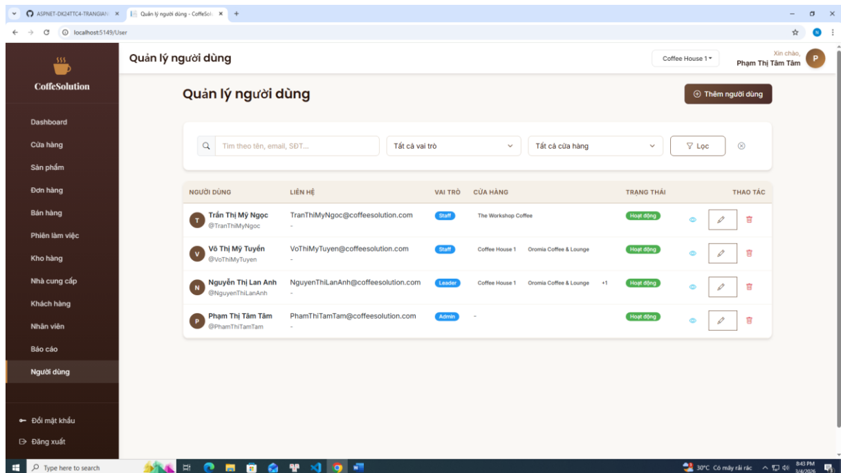
Hình 4.17 Giao diện quản lý người dùng
