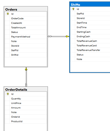
Hình 3.5 Mối quan hệ giữa Order - Shift
