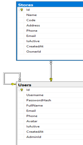
Hình 3.3 Mối quan hệ giữa User - Stores
