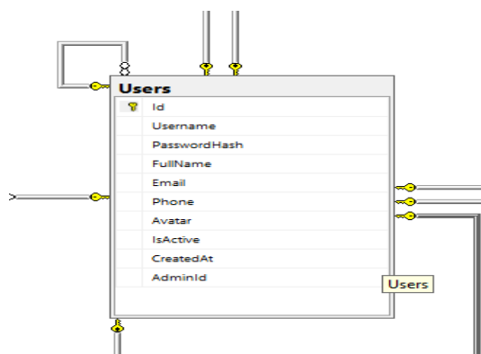
Hình 3.2 Mối quan hệ giữa User - Admin
