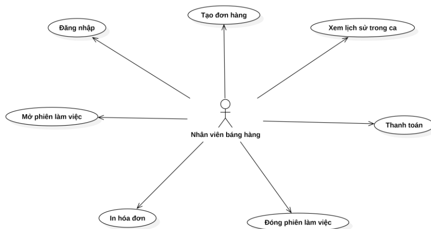
Hình 3.7 Sơ đồ use case nhân viên bán hàng
