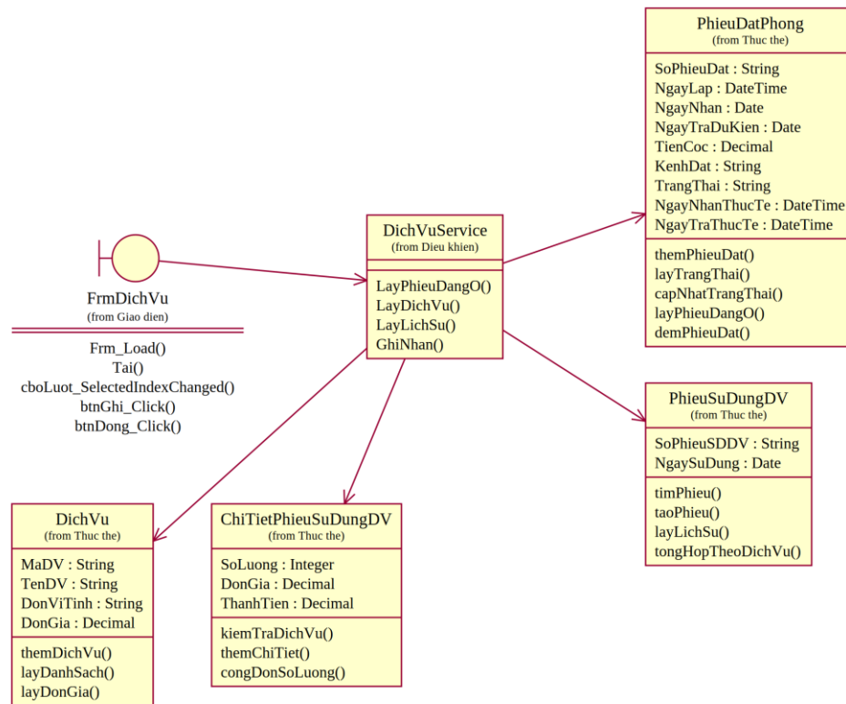
Hình P.19: Thiết kế lớp cho chức năng Ghi nhận dịch vụ
