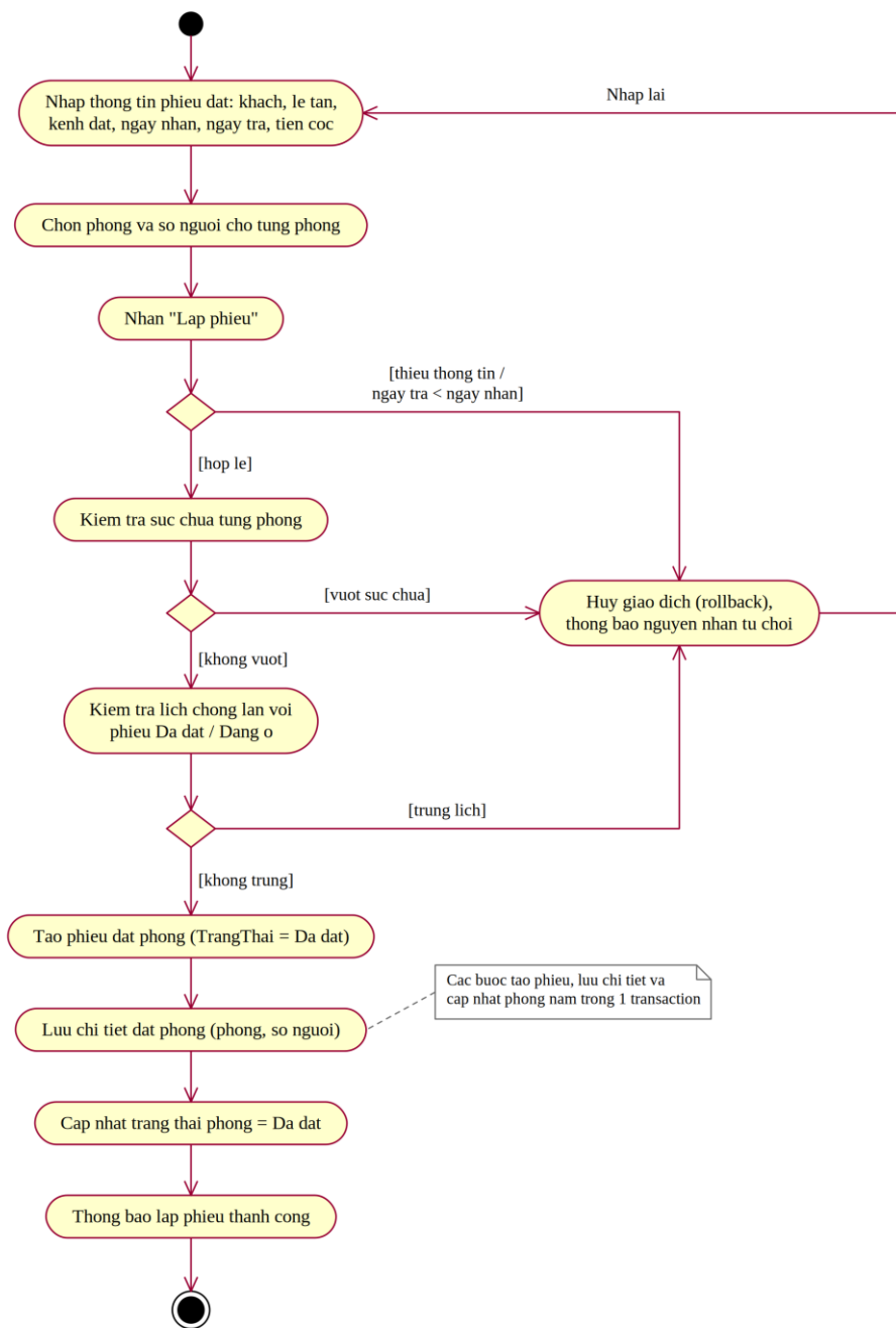
Hình P.22: Biểu đồ hoạt động của chức năng Đặt phòng
