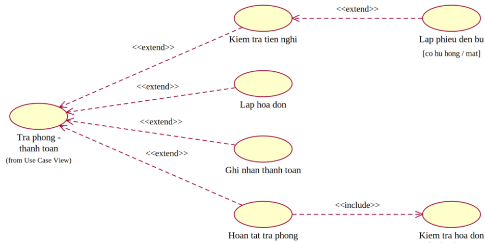
Hình P.4: Phân rã use case Trả phòng - thanh toán
