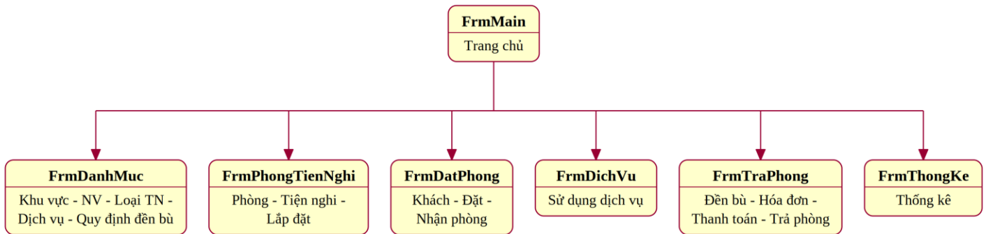
Hình 6. Sơ đồ điều hướng hệ thống Form. Tham khảo
