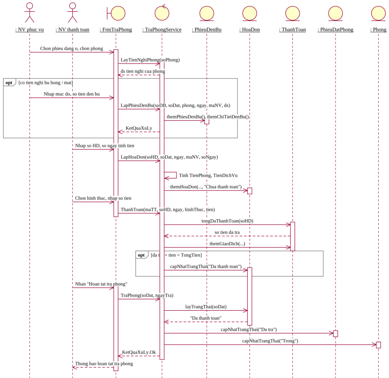
Hình P.13: Biểu đồ tuần tự cho chức năng Trả phòng - thanh toán
