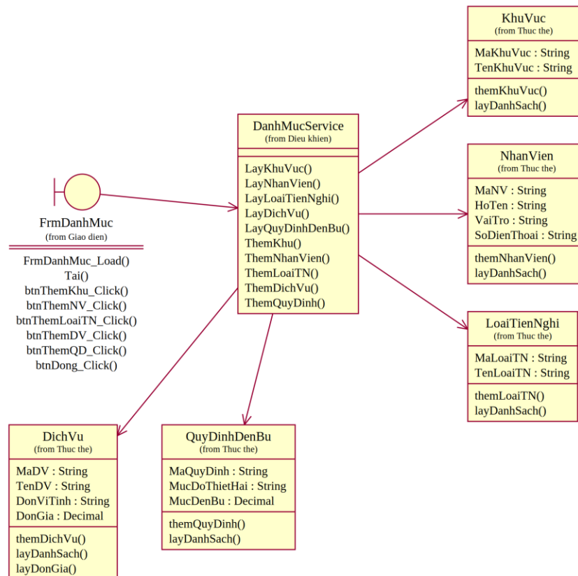
Hình P.16: Thiết kế lớp cho chức năng Quản lý danh mục
