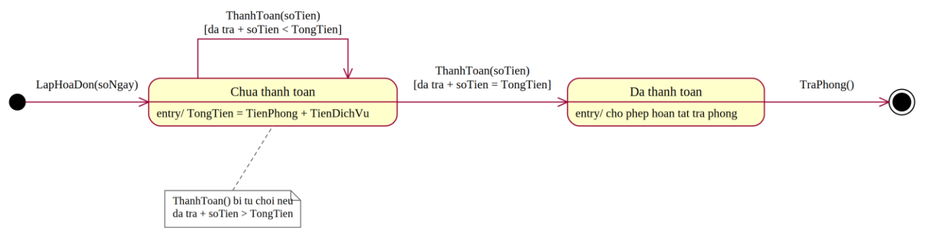
Hình P.8: Biểu đồ trạng thái lớp HoaDon
