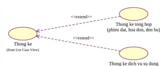
Hình P.5: Phân rã use case Thống kê
