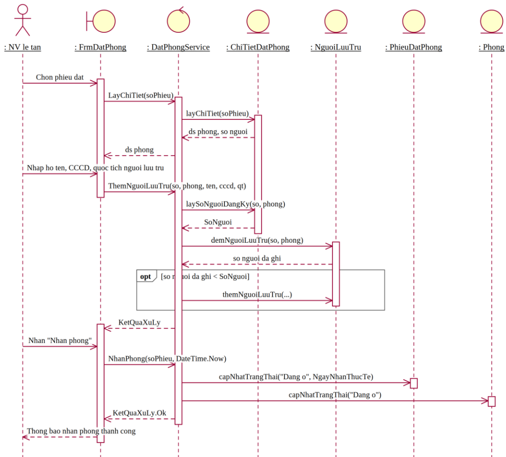
Hình P.10: Biểu đồ tuần tự cho chức năng Nhận phòng
