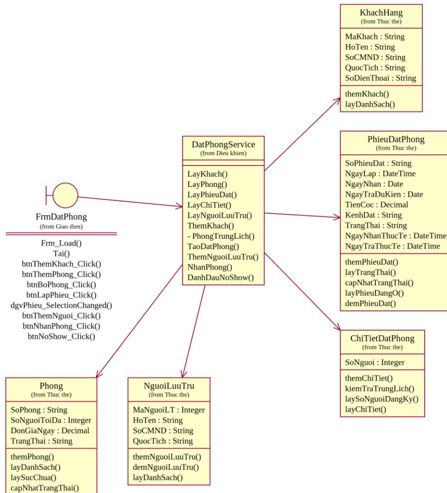
Hình P.18: Thiết kế lớp cho chức năng Đặt / nhận phòng
