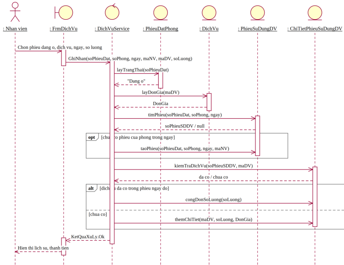
Hình P.12: Biểu đồ tuần tự cho chức năng Ghi nhận dịch vụ
