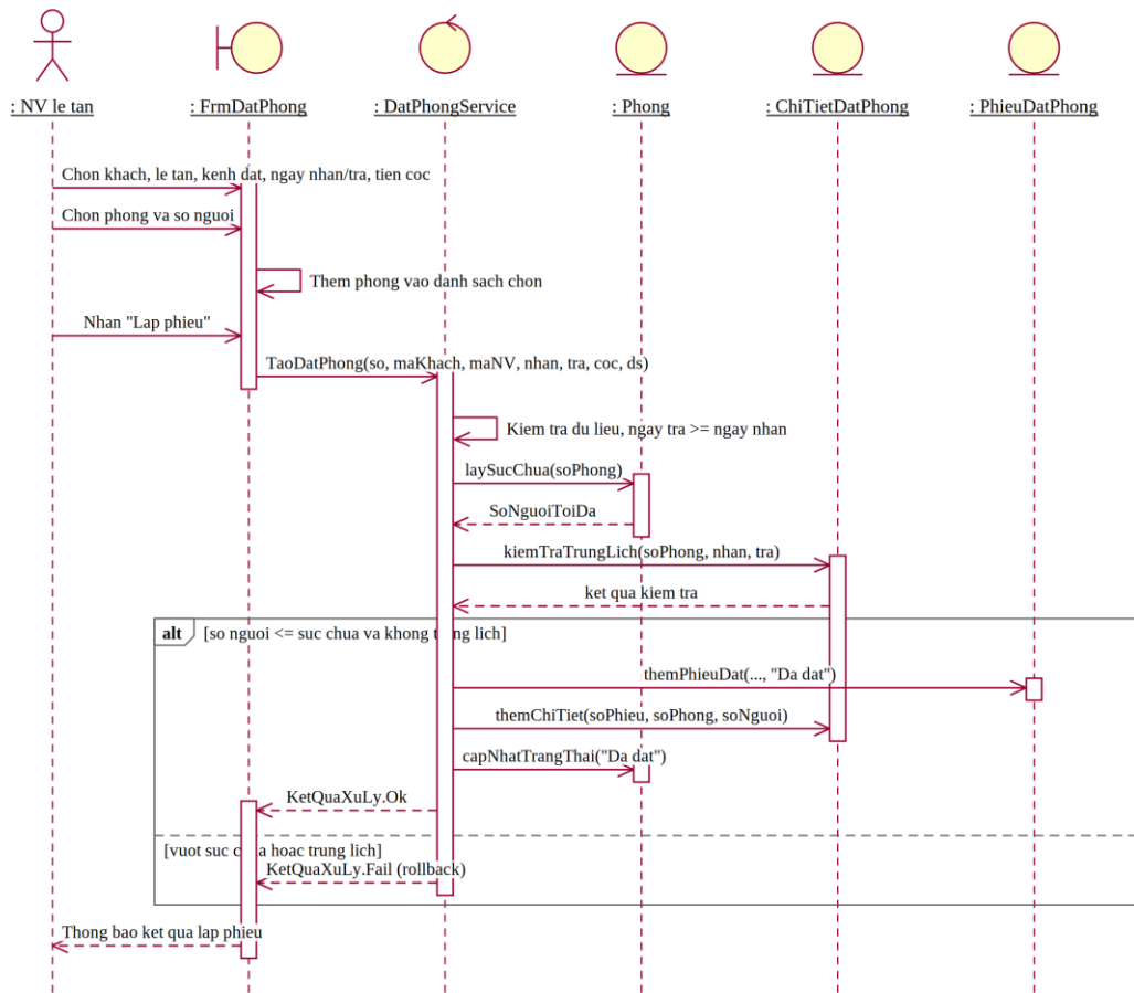
Hình P.9: Biểu đồ tuần tự cho chức năng Đặt phòng
