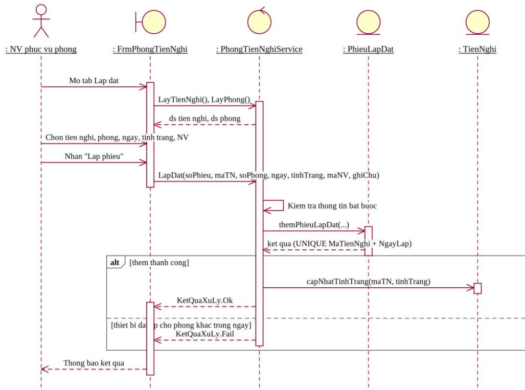
Hình P.11: Biểu đồ tuần tự cho chức năng Lập phiếu lắp đặt
