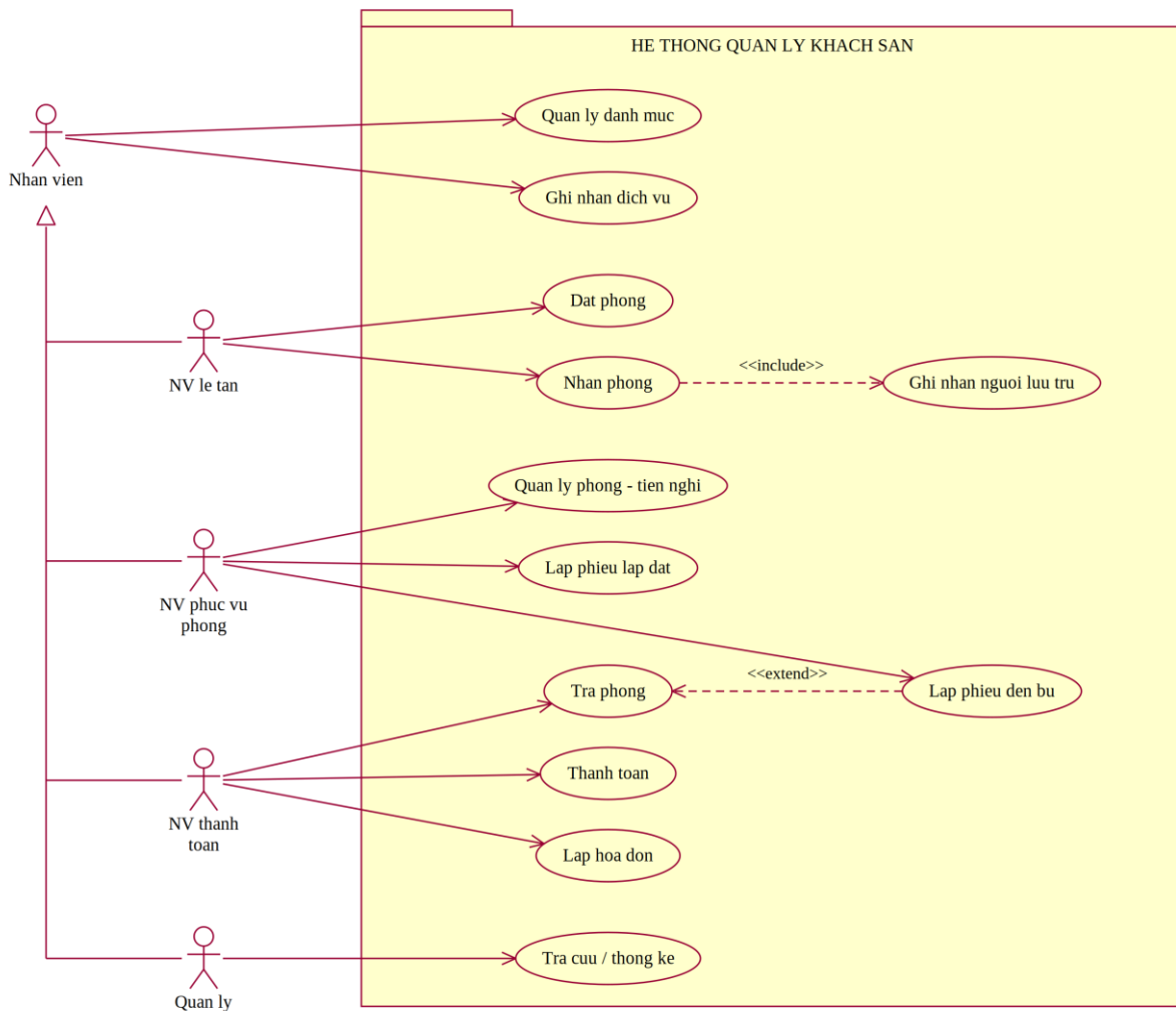
Hình P.1: Biểu đồ use case tổng quát của hệ thống
