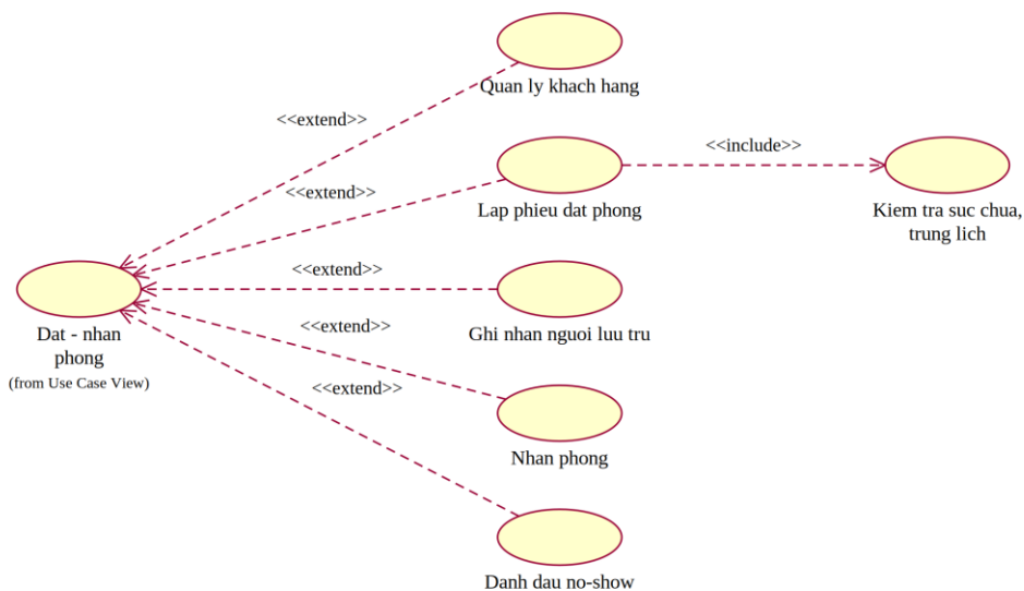
Hình P.3: Phân rã use case Đặt / nhận phòng
