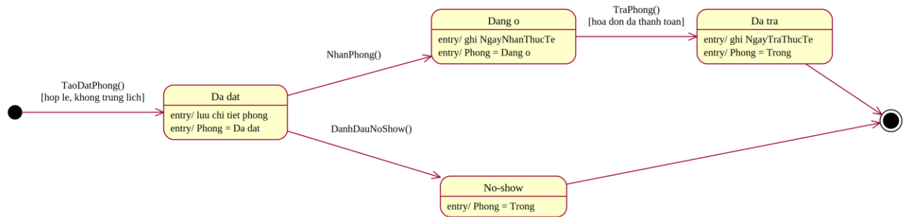
Hình P.7: Biểu đồ trạng thái lớp PhieuDatPhong
