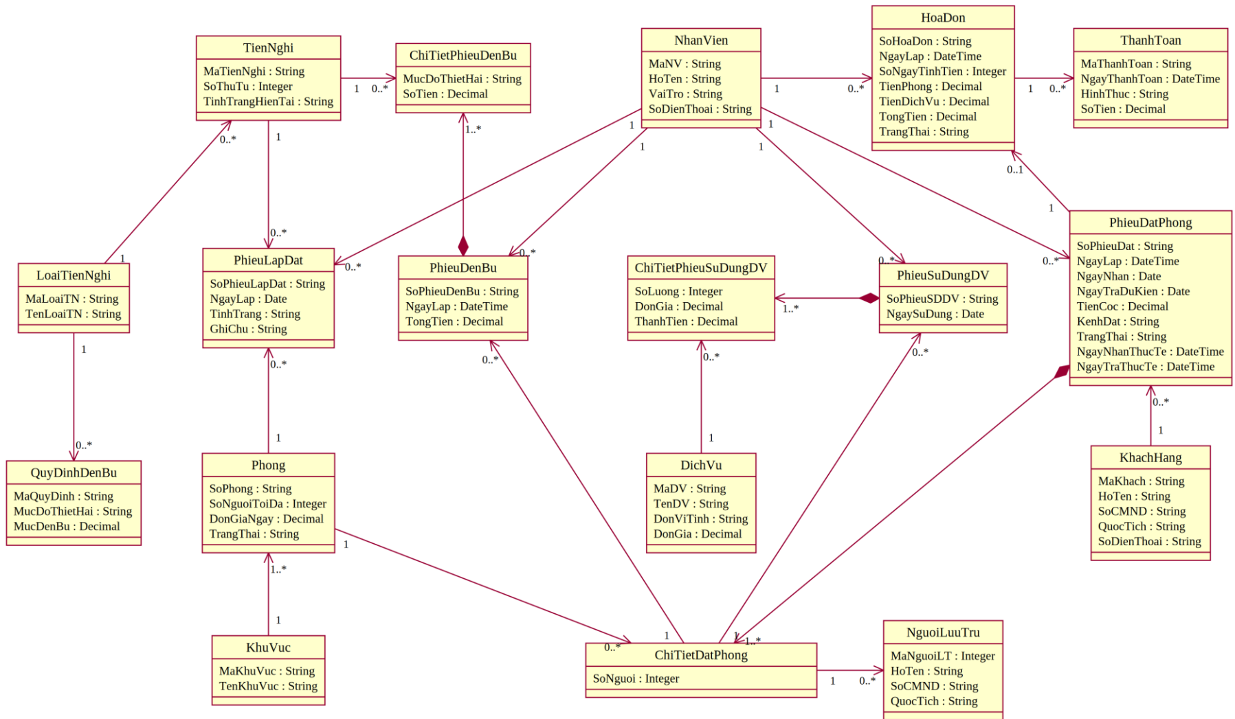
Hình P.6: Biểu đồ lớp phân tích của hệ thống
