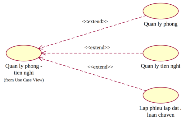
Hình P.2: Phân rã use case Quản lý phòng - tiện nghi
