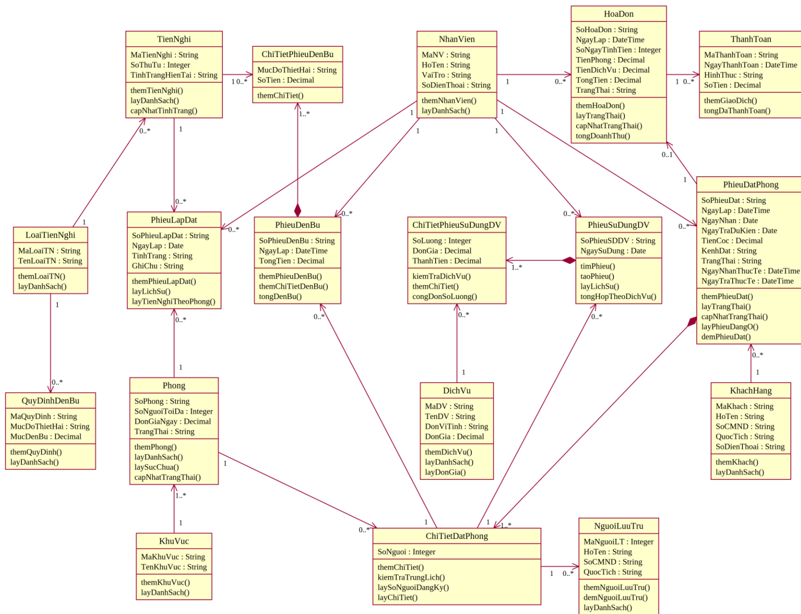
Hình P.15: Biểu đồ lớp thiết kế chi tiết của hệ thống
