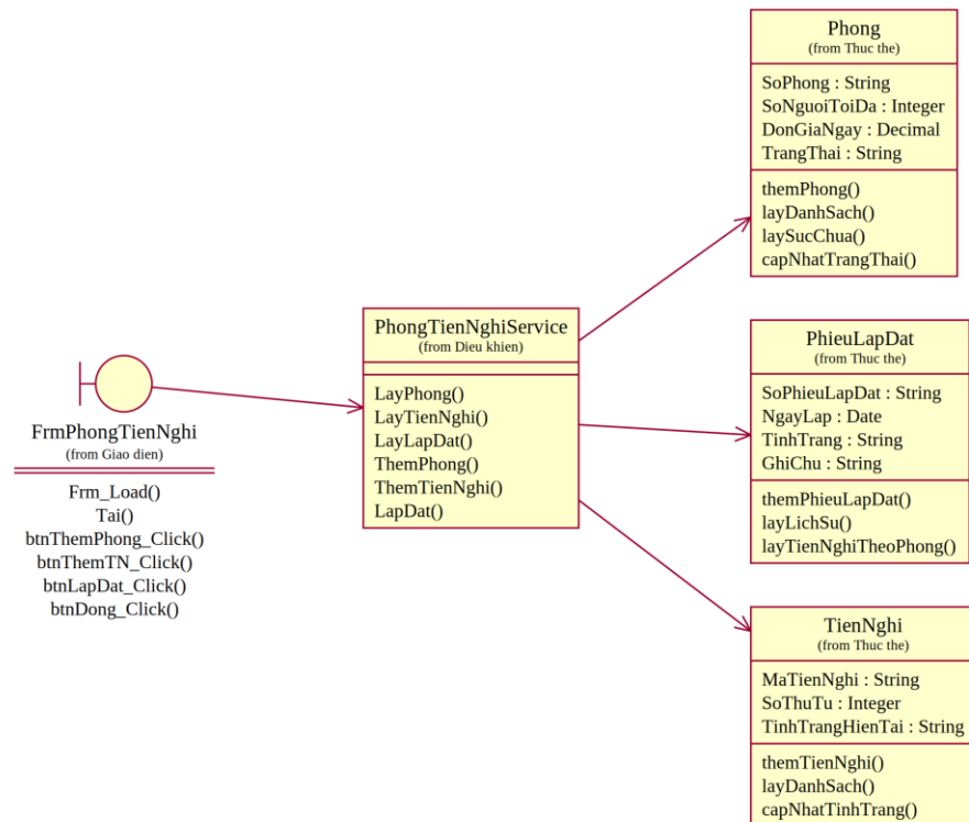
Hình P.17: Thiết kế lớp cho chức năng Quản lý phòng - tiện nghi
