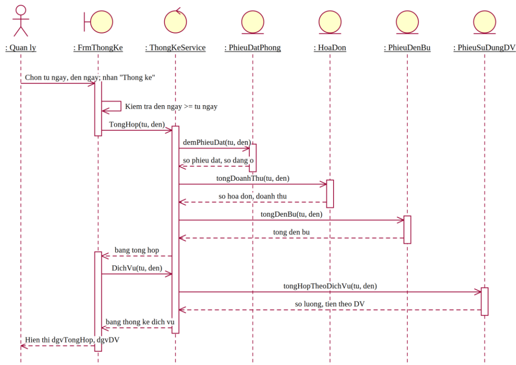
Hình P.14: Biểu đồ tuần tự cho chức năng Thống kê
