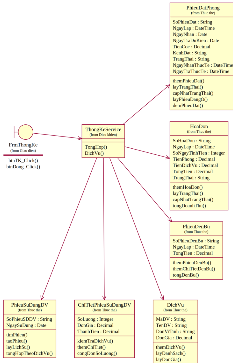
Hình P.21: Thiết kế lớp cho chức năng Thống kê
