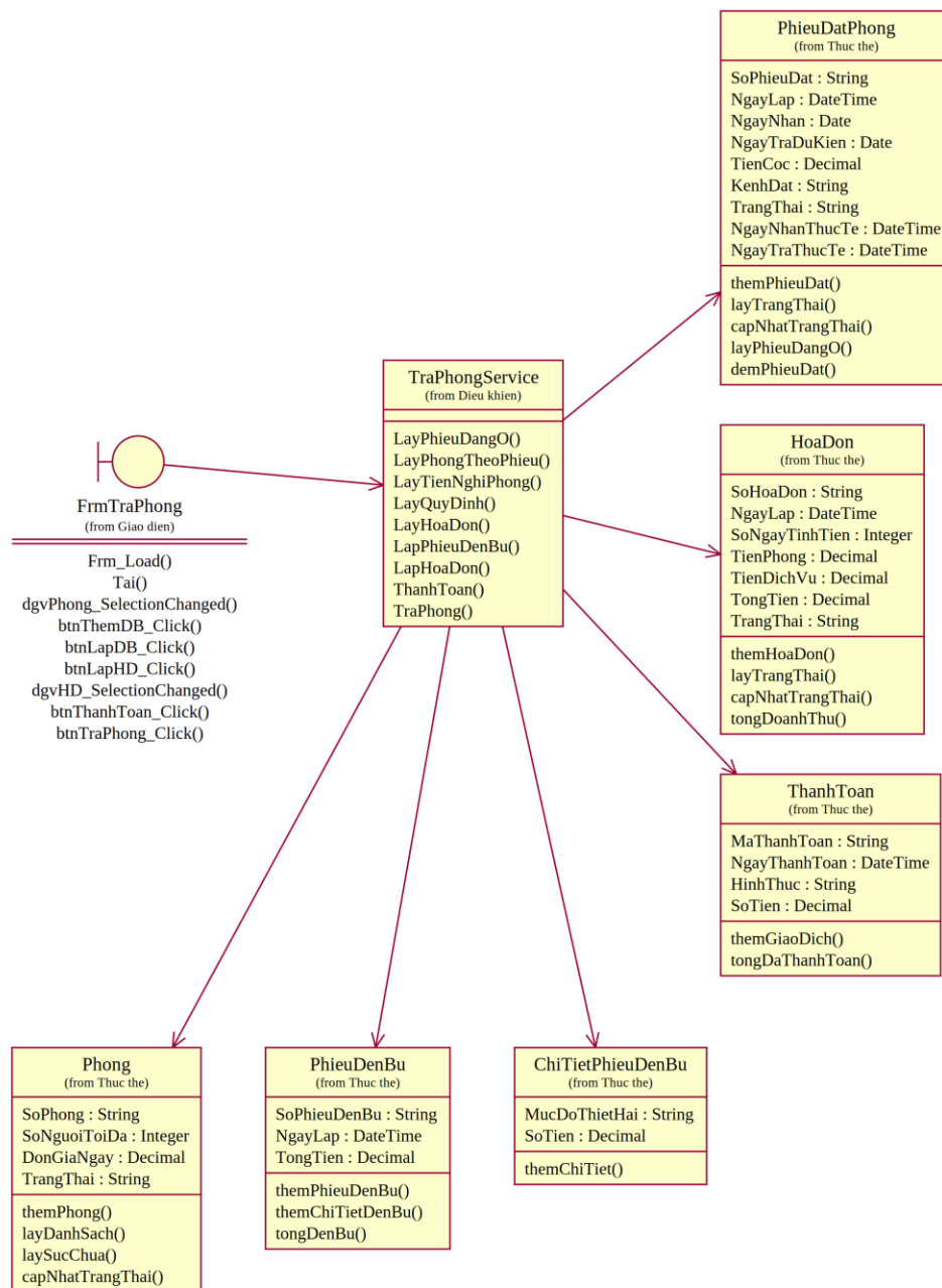
Hình P.20: Thiết kế lớp cho chức năng Trả phòng - thanh toán
