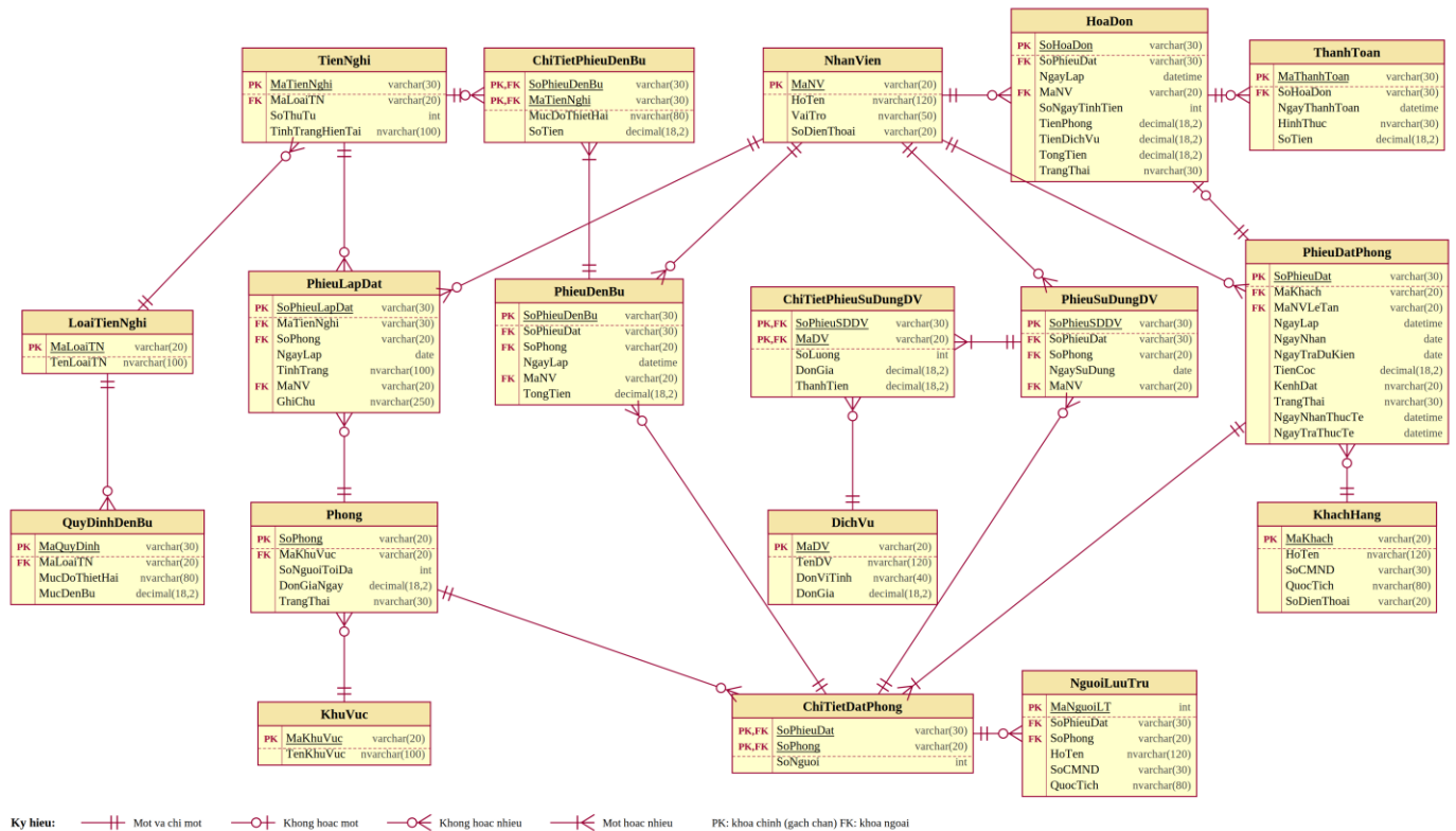
Hình 5. ERD triển khai SQL Server
