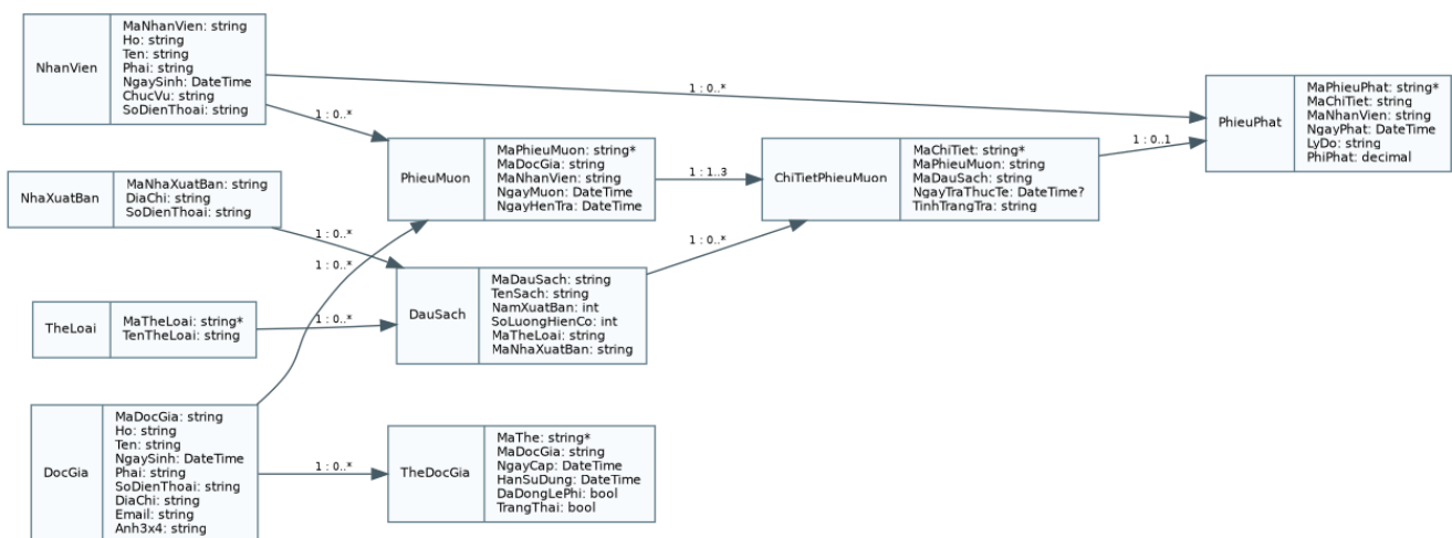
Hình 2. Class Diagram
