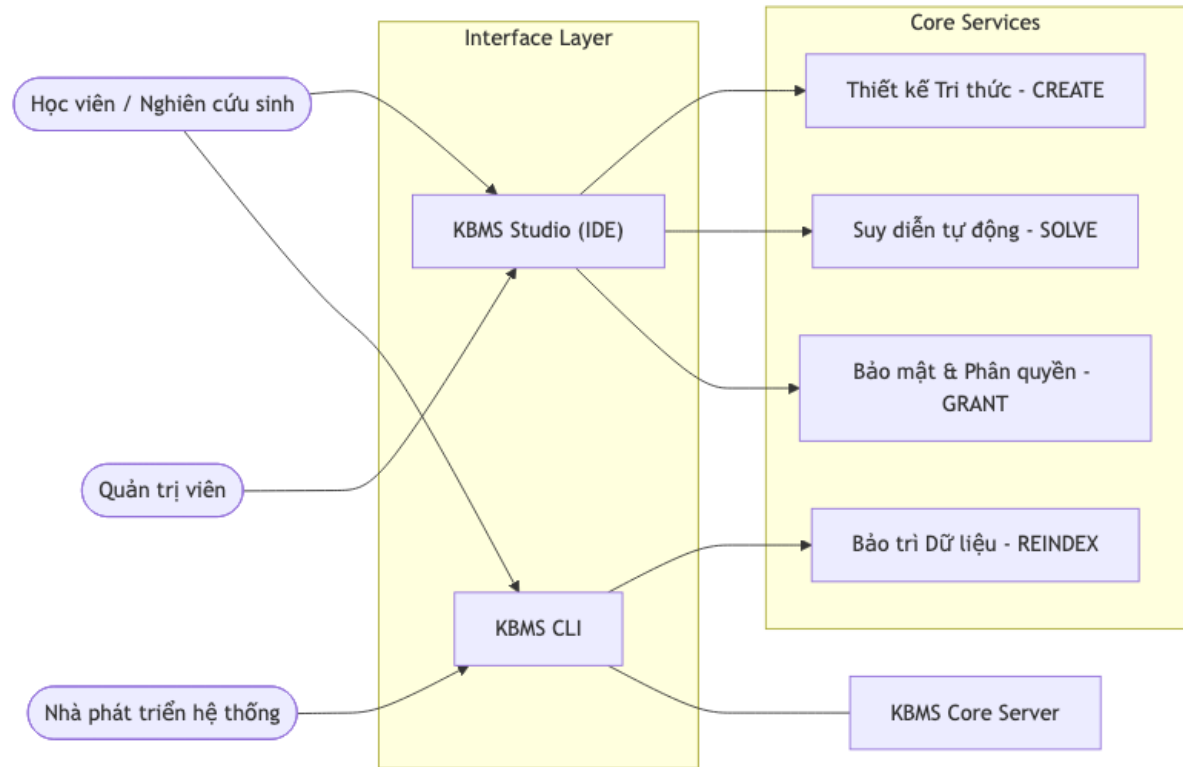
Hình 3.2: Sơ đồ Use Case tổng quát sự tương tác giữa người dùng và các dịch vụ lõi.
