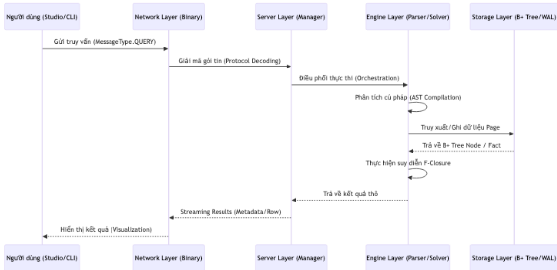
Hình 3.3: Sơ đồ Sequence mô tả quy trình xử lý yêu cầu phân tầng trong KBMS V3.
