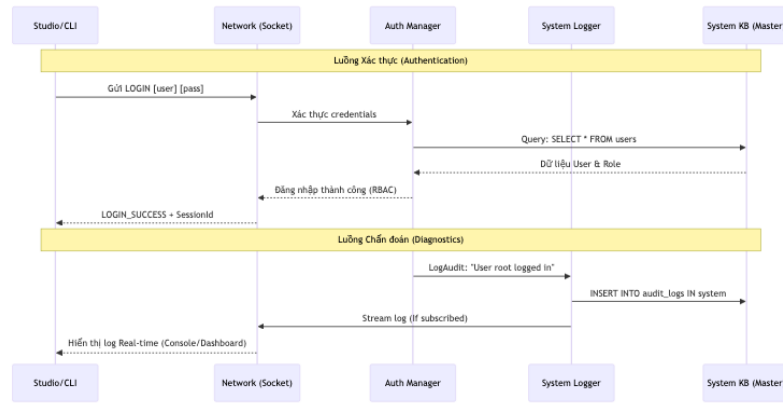
Hình 4.3: Sơ đồ luồng chẩn đoán và kiểm soát an ninh hệ thống.
