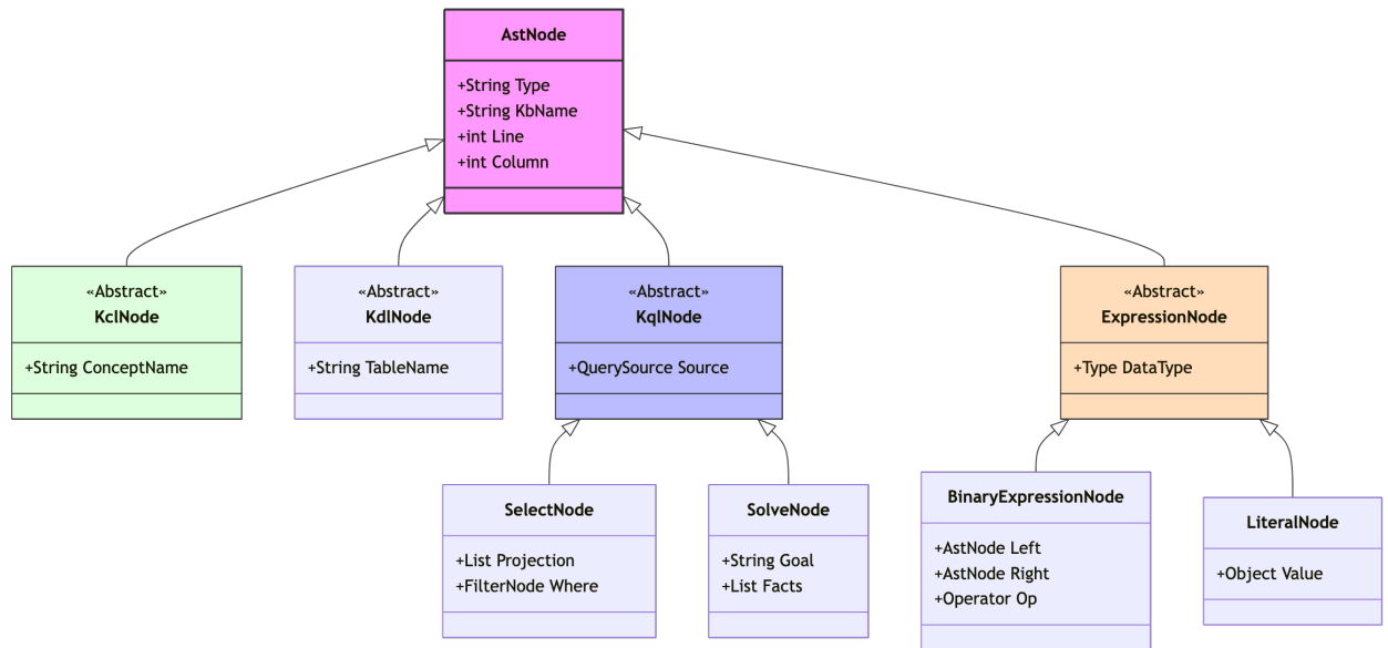
Hình 4.23: Sơ đồ phân cấp các đối tượng nốt AST phục vụ điều phối tri thức.
