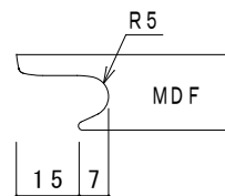
Ｊ取手加工図
