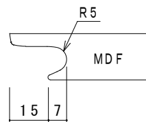
J取手加工図
