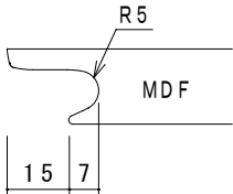
J取手加工図
