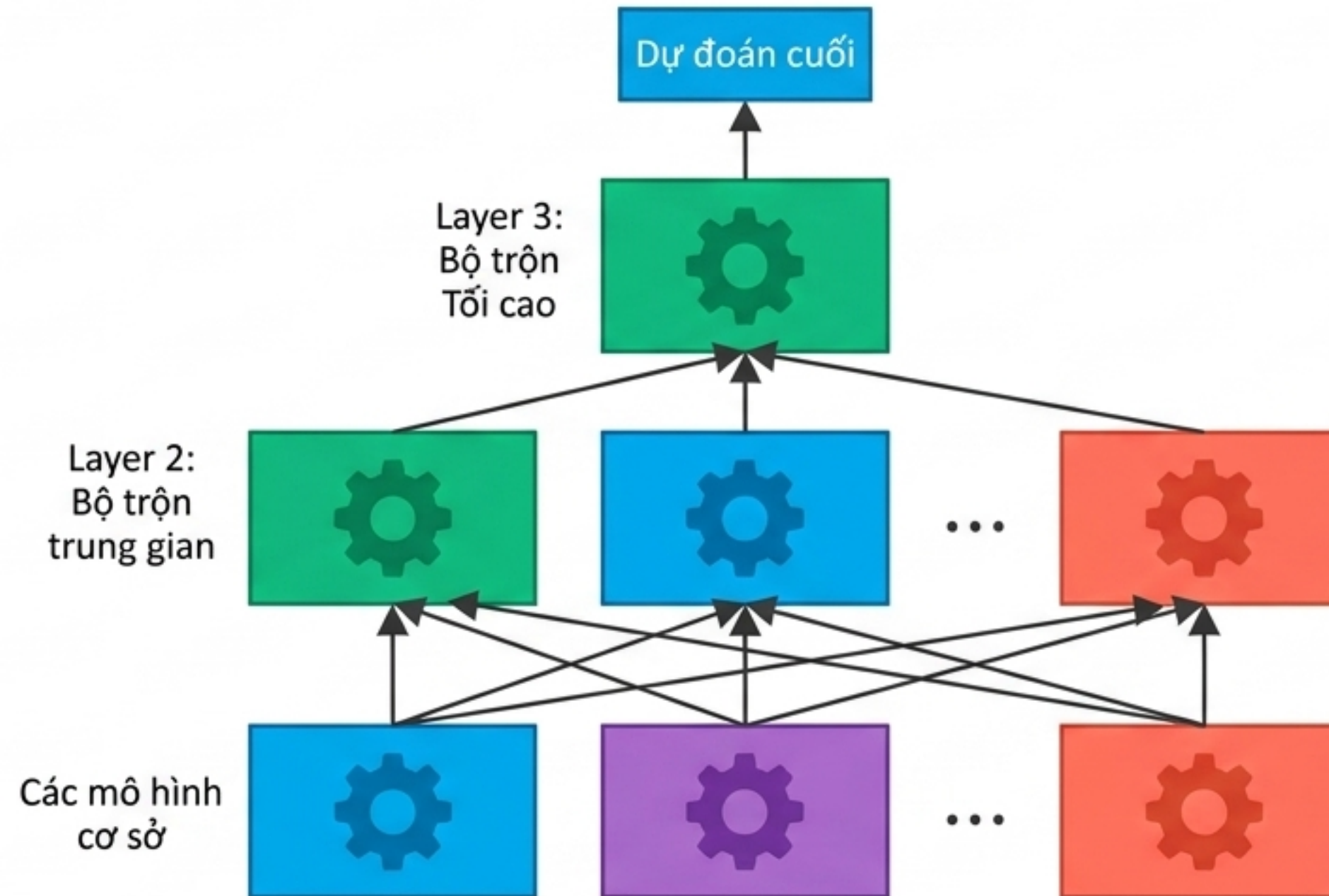
Hình 7-13. Mạng Stacking đa tầng (Multi-layer Stacking Ensemble)
