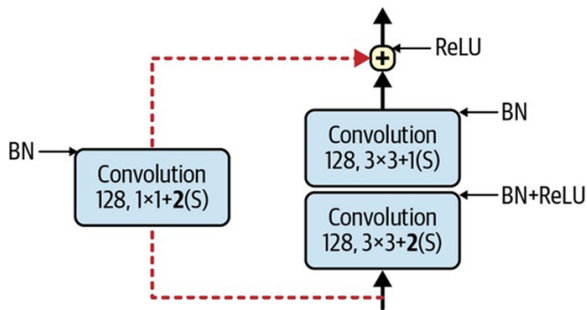
Hình 14-19: Khối thay đổi kích thước
