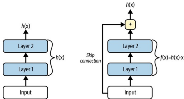
Hình 14-16: Khối Residual Learning cơ bản
