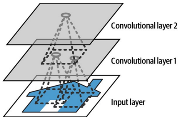
Hình 14-2: Kết nối cục bộ giữa 2 lớp CNN
