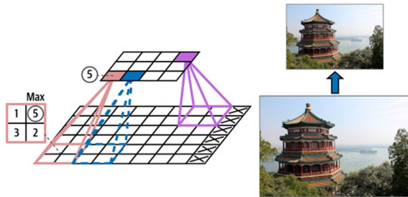
Hình 14-9: Lớp gộp cực đại (Max Pooling Layer)
