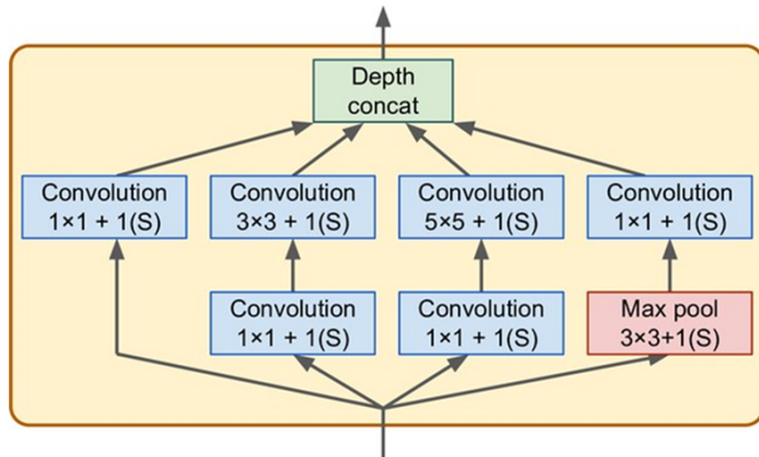
Hình 14-14: Kiến trúc một mô-đun Inception
