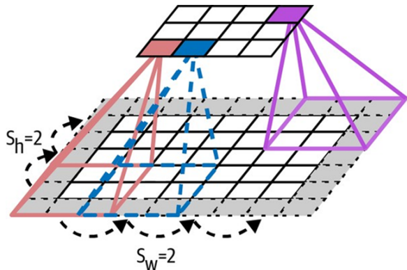
Hình 14-4: Lớp tích chập với bước nhảy \text{Stride}=2
