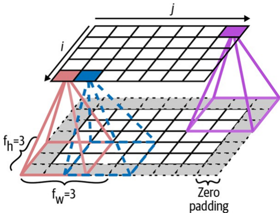
14-3: Kết nối với Padding
