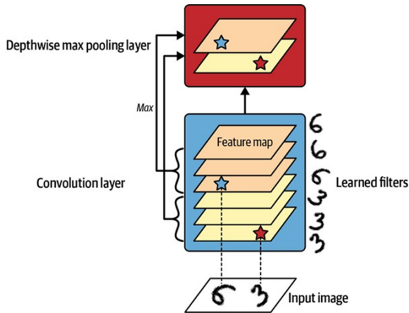
Hình 14-11: Tính bất biến nhờ Max Pooling
