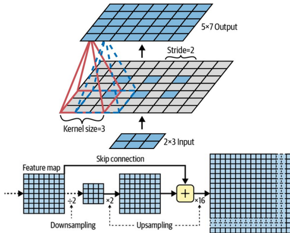
Hình 14-28, 14-29: Phép tích chập ngược (Up-sampling)
