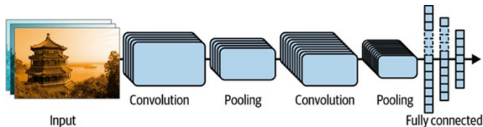
Hình 14-12: Mạng Nơ-ron Tích chập điển hình
