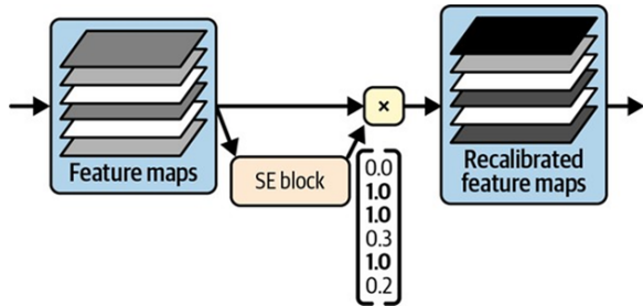
Hình 14-22: Khối SE (Squeeze-and-Excitation)
