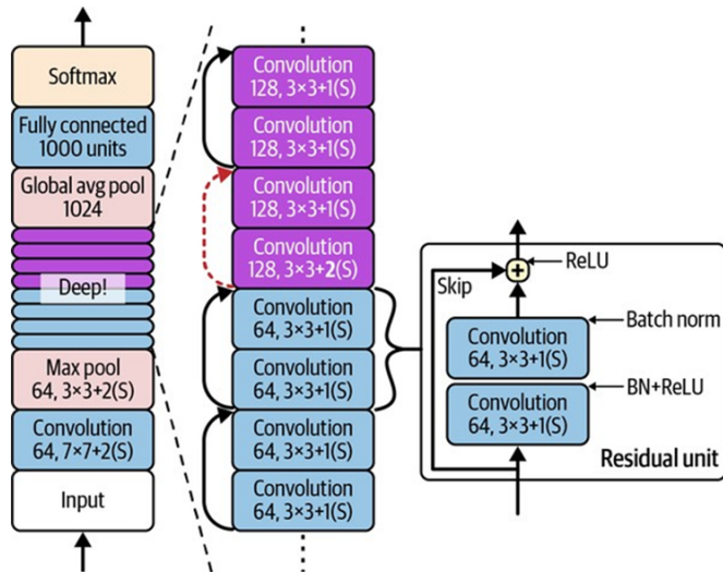
14-18: Kiến trúc tổng thể ResNet
