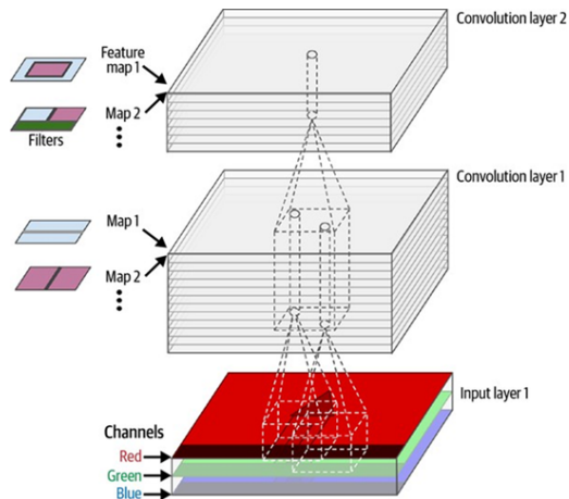
Hình 14-6: Đầu vào đa kênh và Đầu ra đa kênh
