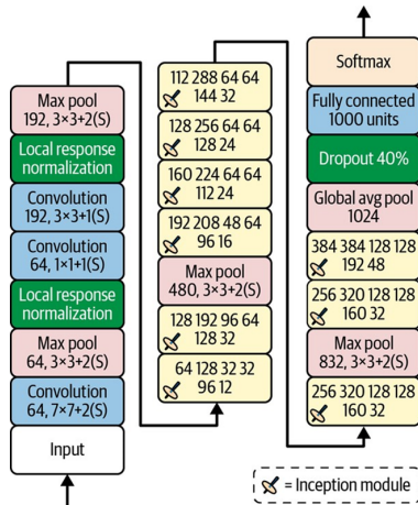
Hình 14-15: Toàn cảnh Kiến trúc GoogLeNet sâu thẳm
