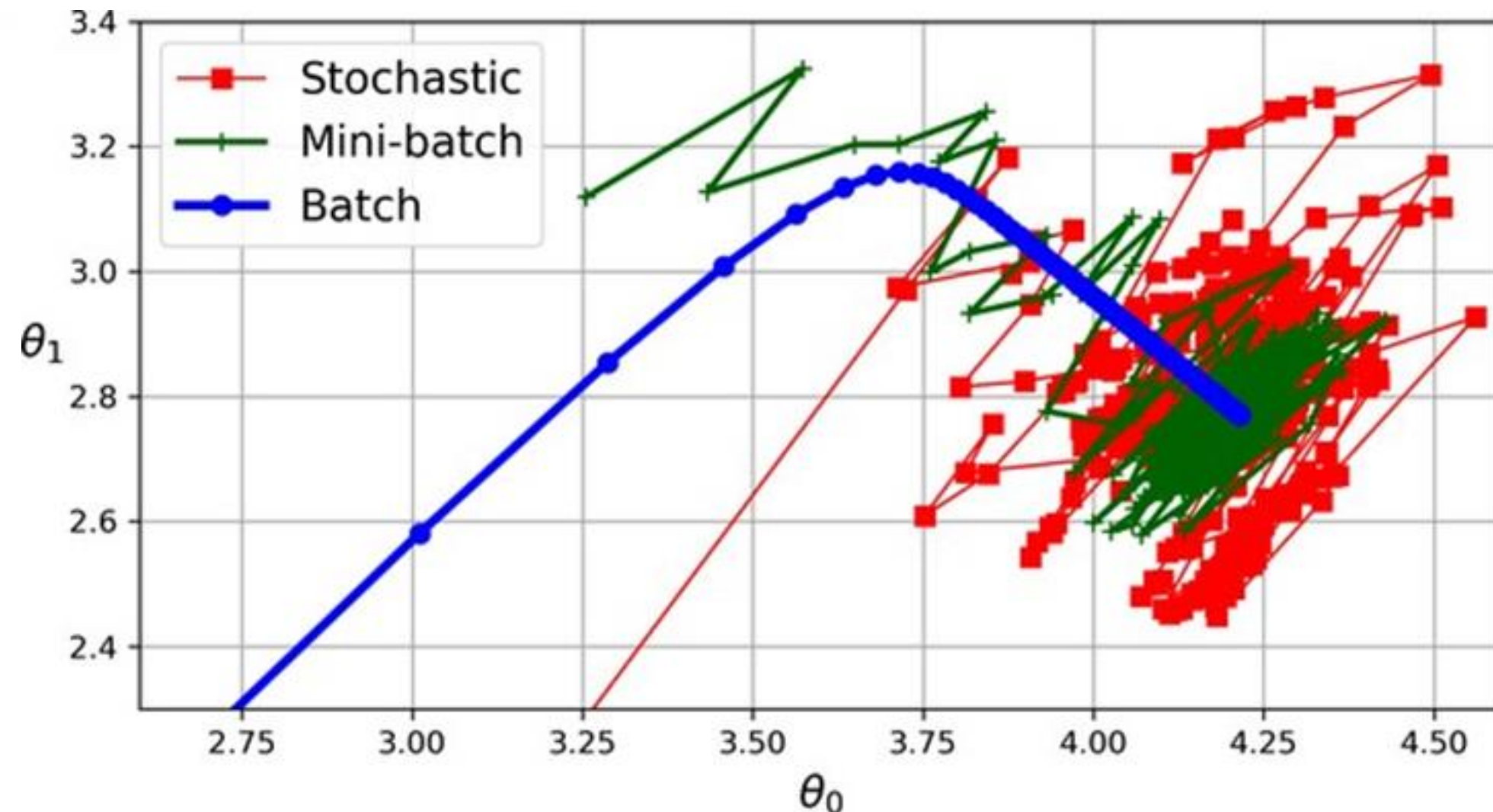
Hình 4-11. Đường đi của 3 thuật toán GD
