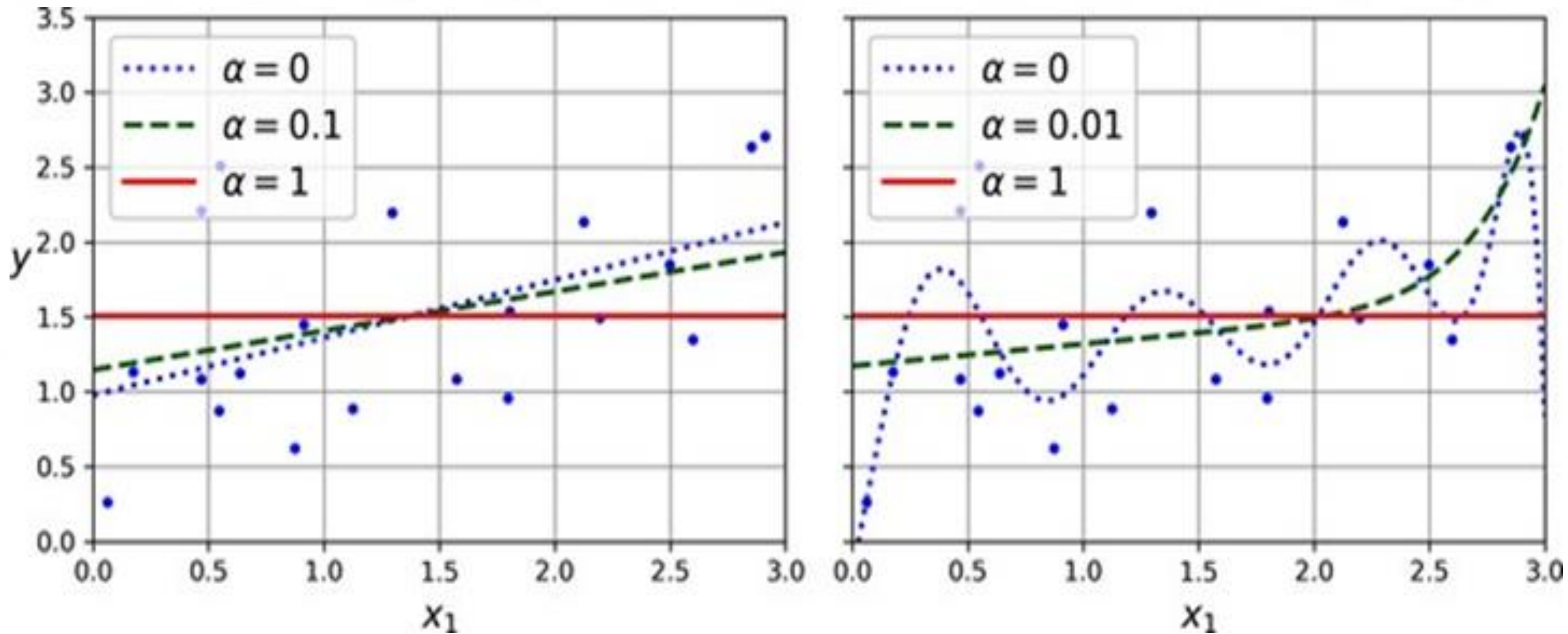
Hình 4-18. Hồi quy Lasso trên mô hình tuyến tính và đa thức
