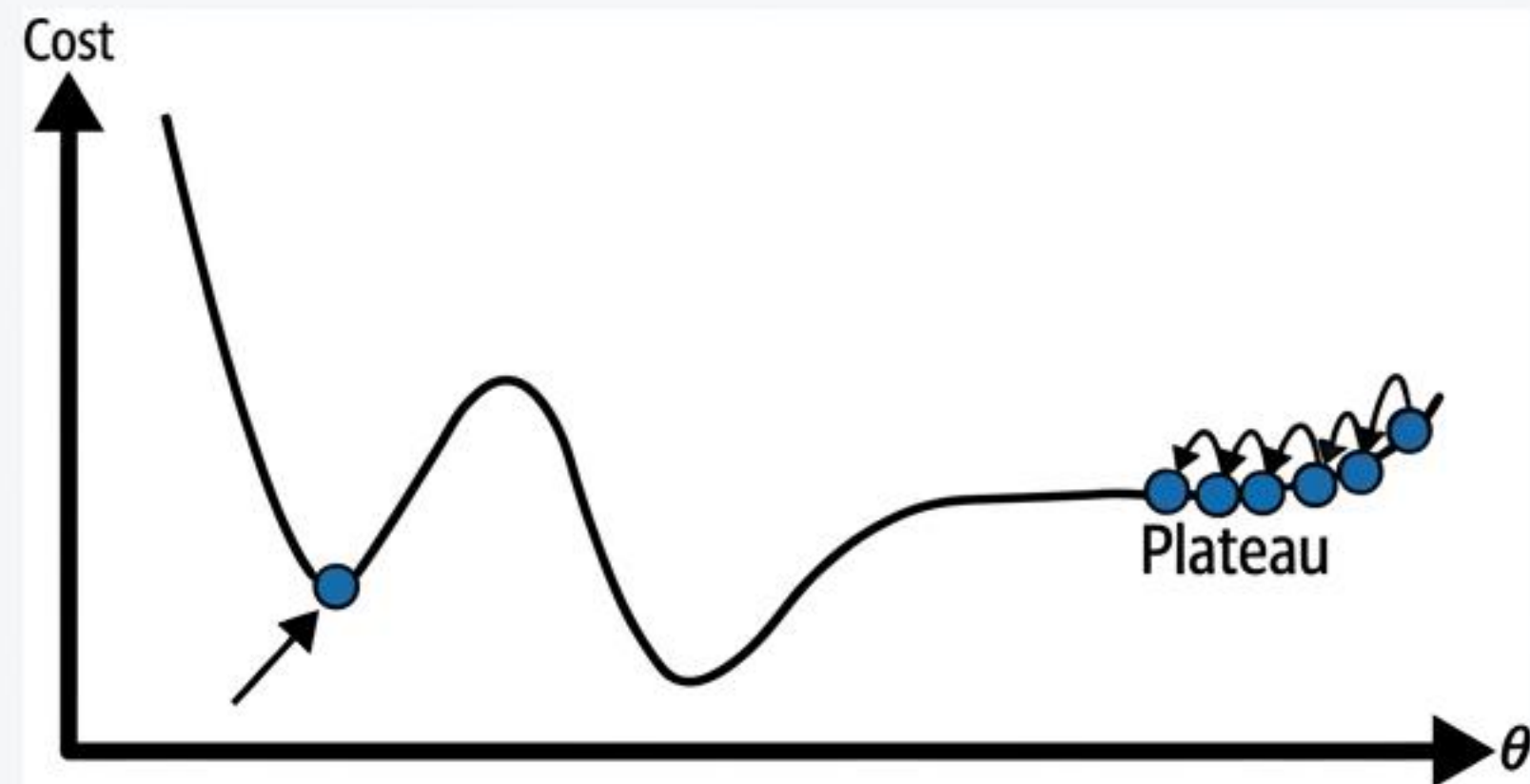
Hình 4-6. Cạm bẫy cực tiểu cục bộ
