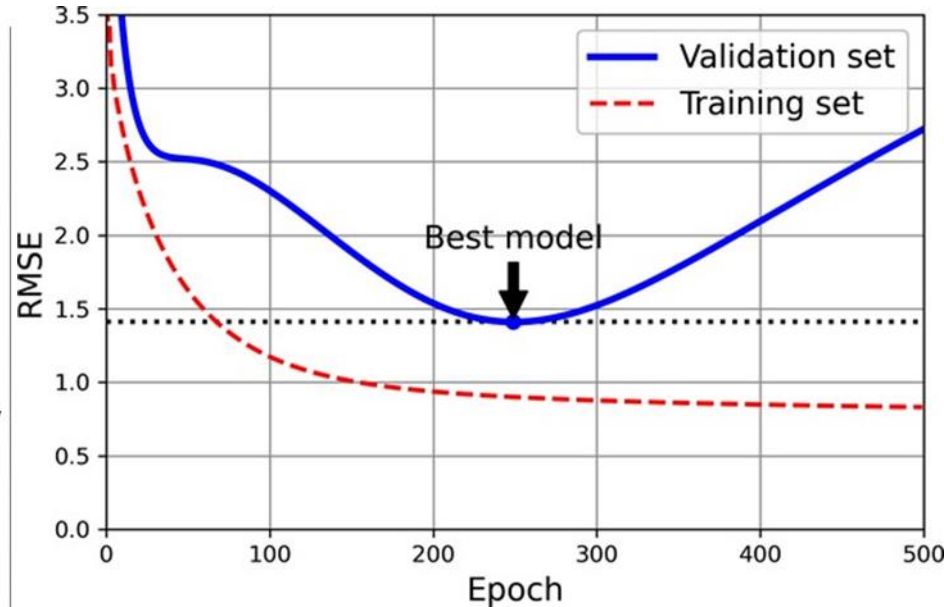
Hình 4-20. Early Stopping (Mũi tên chỉ thời điểm tốt nhất. Các bước sau chỉ làm mô hình tệ hơn...)
