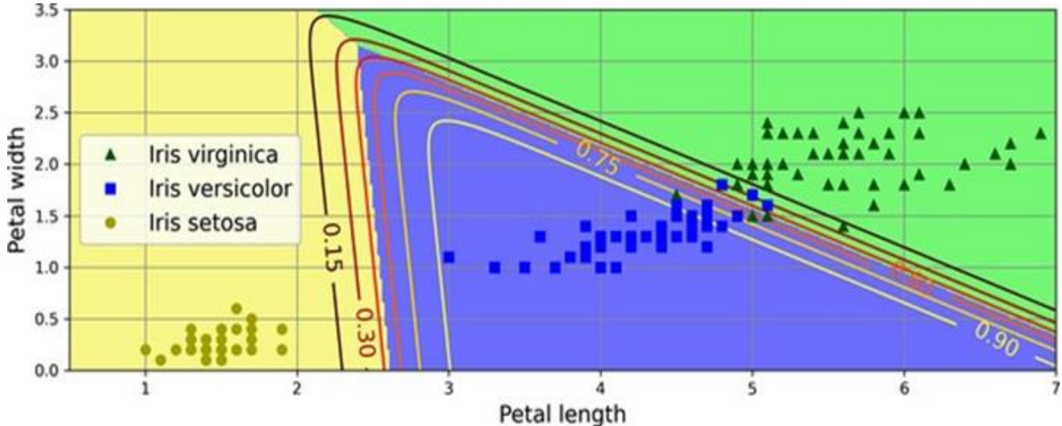
Hình 4-25. Ranh giới quyết định hồi quy Softmax (Mô phỏng).
