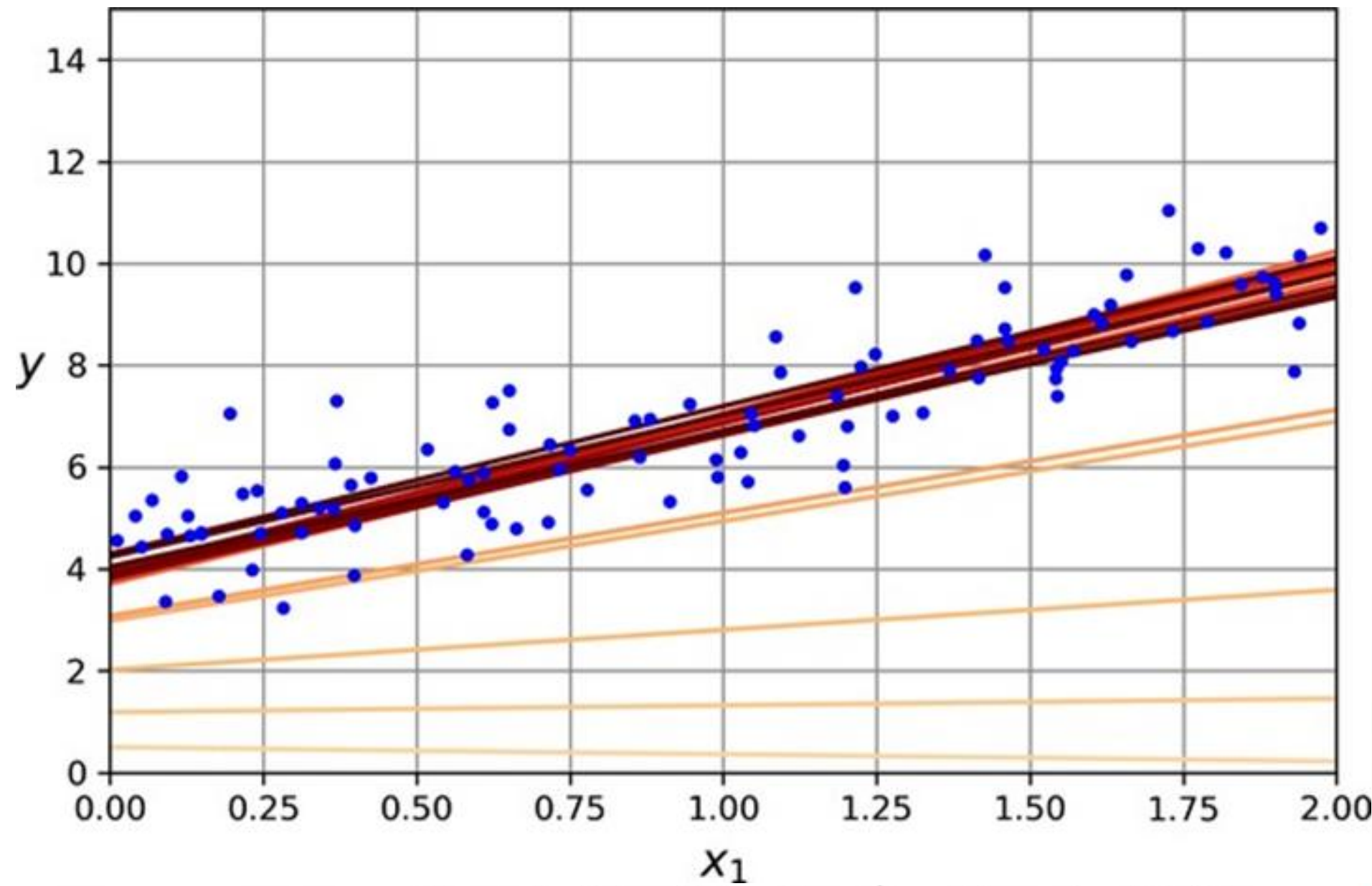
Hình 4-10. 20 bước đầu tiên của SGD
