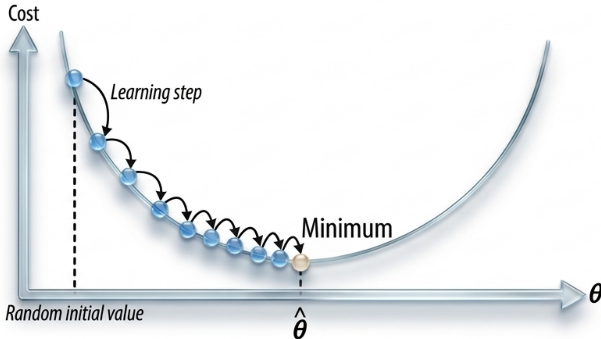
Hình 4-3. Gradient Descent
