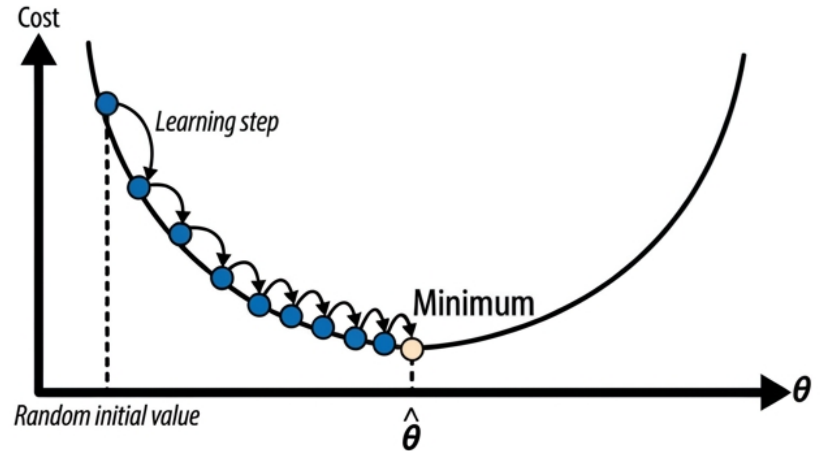
Hình 4-3. Gradient Descent
