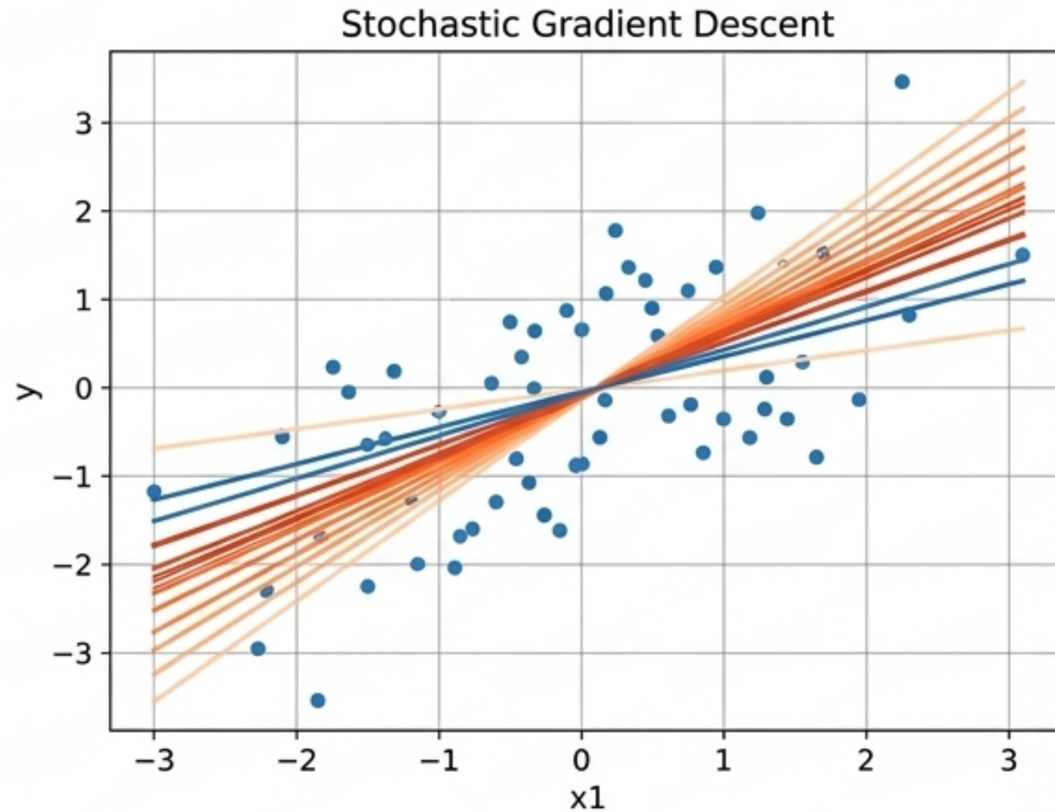
Hình 4-10. 20 bước đầu tiên của SGD
