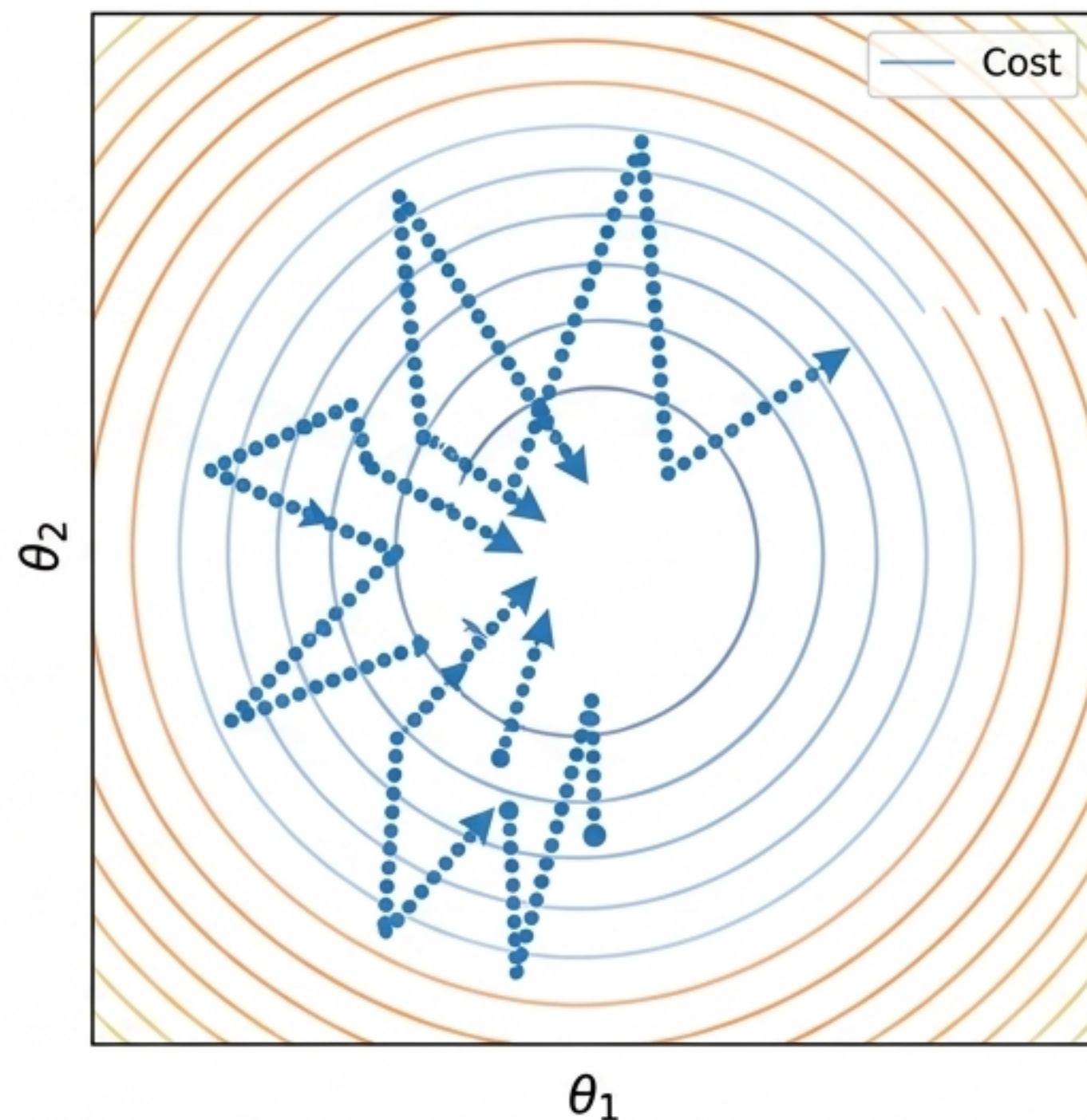
Hình 4-9. Đặc điểm bất thường của SGD
