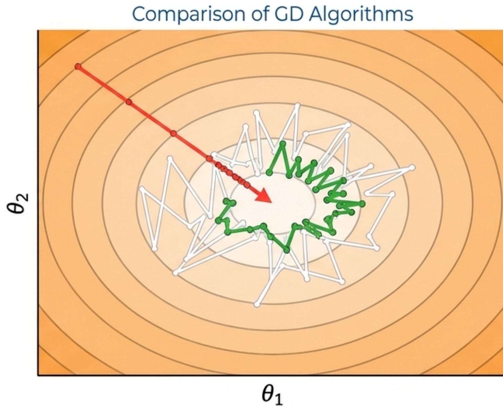
Hình 4-11. Đường đi của 3 thuật toán GD
