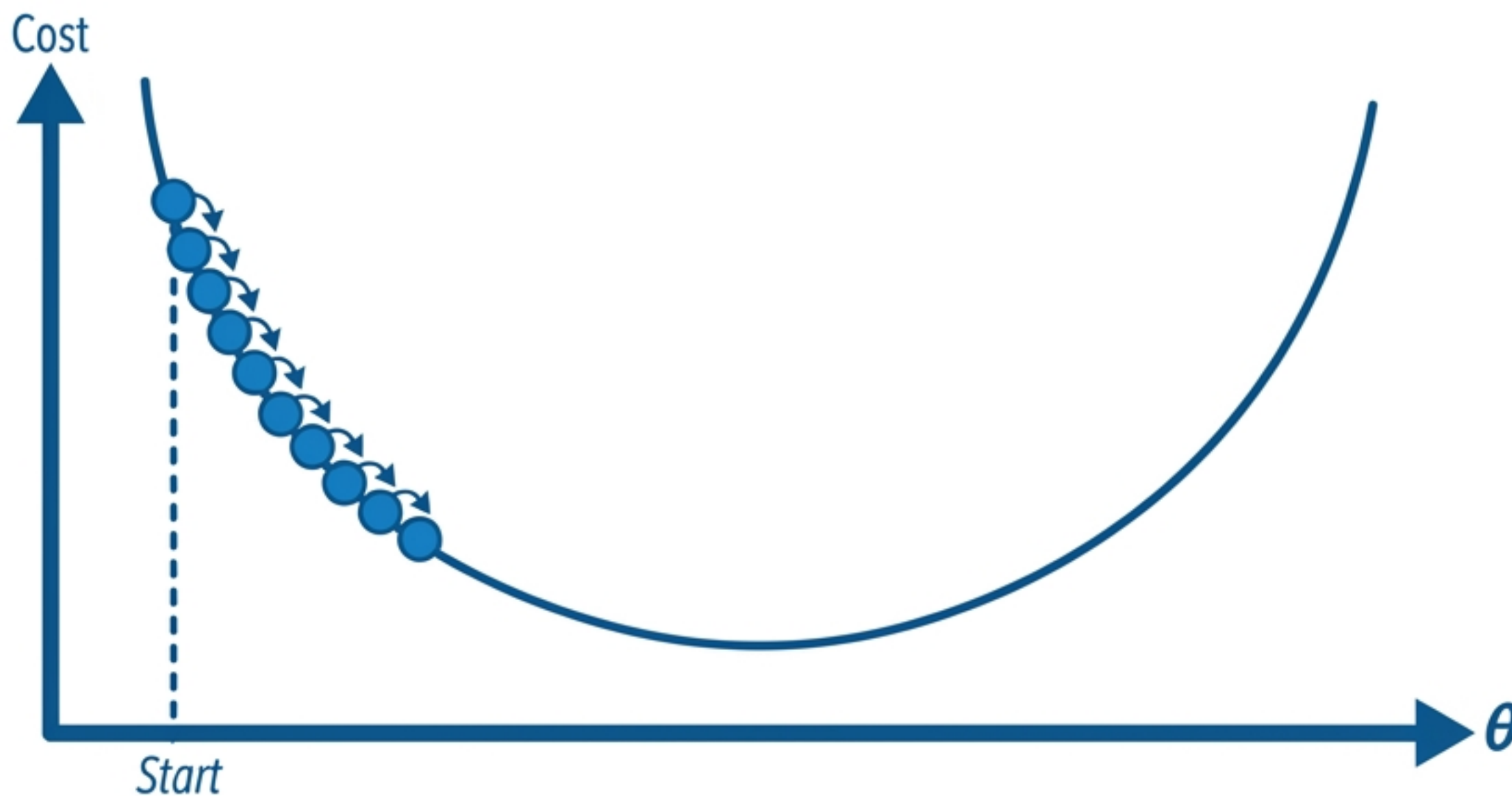
Hình 4-4. Tốc độ học quá nhỏ
