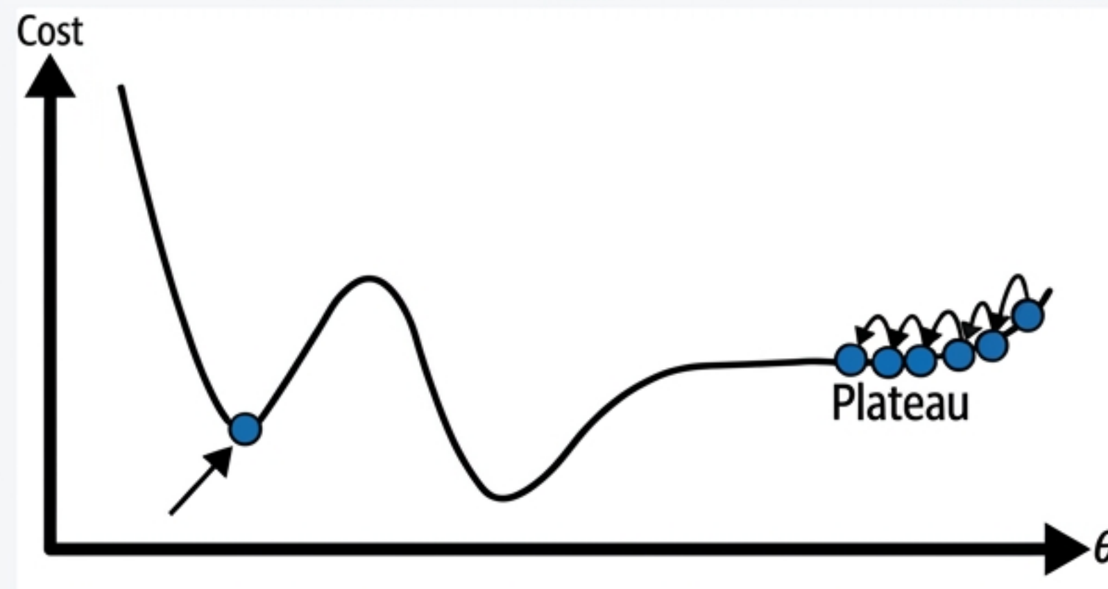
Hình 4-6. Cạm bẫy cực tiểu cục bộ
