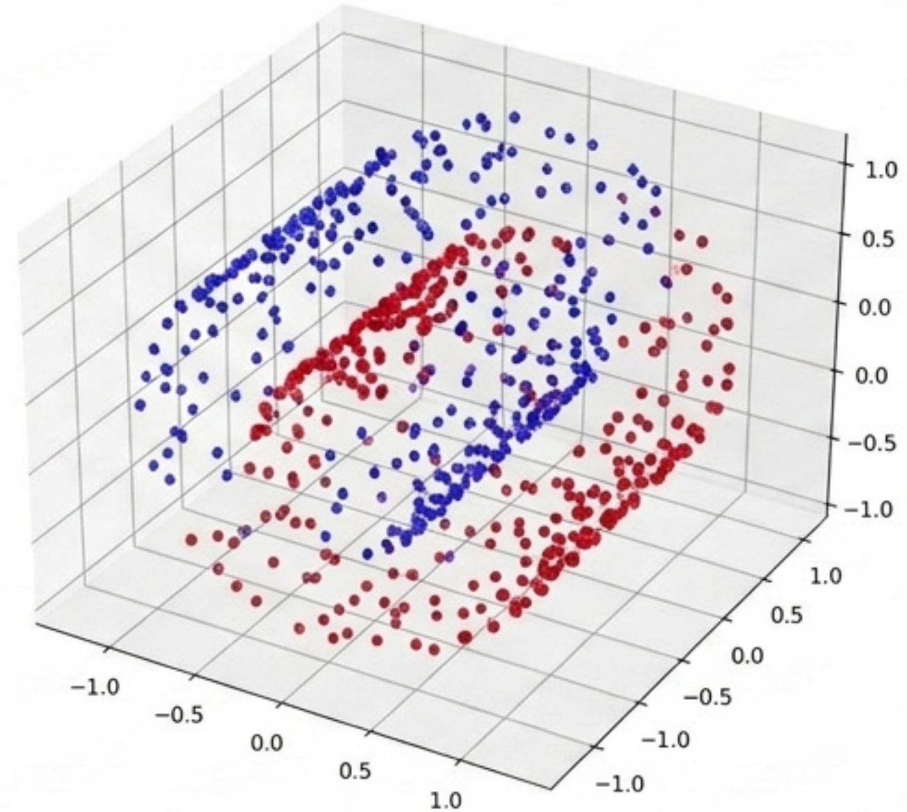
Tập dữ liệu Swiss roll
