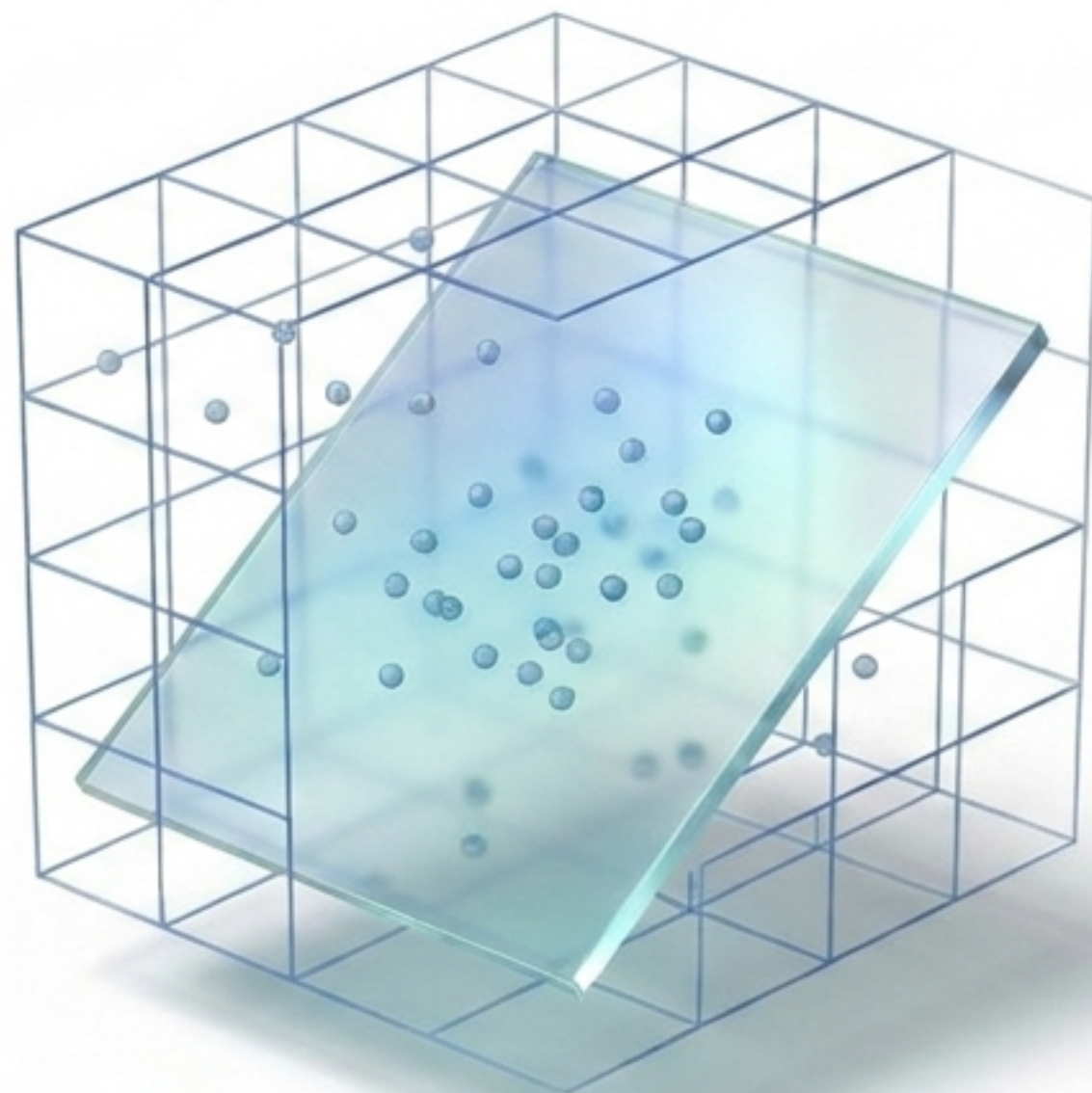
Tập dữ liệu 3D gần không gian con 2D Hình 8-2. Một tập dữ liệu 3D nằm gần một không gian con 2D (mặt phẳng)
