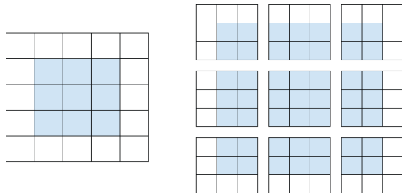
Hình 8.4: Trích xuất các patches 3 \times 3
