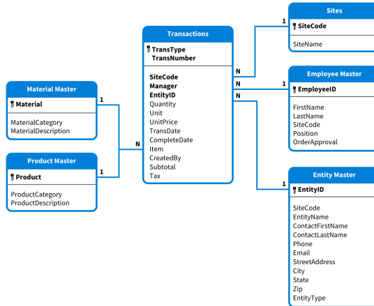
Entity-Relationship Diagram (ERD)
