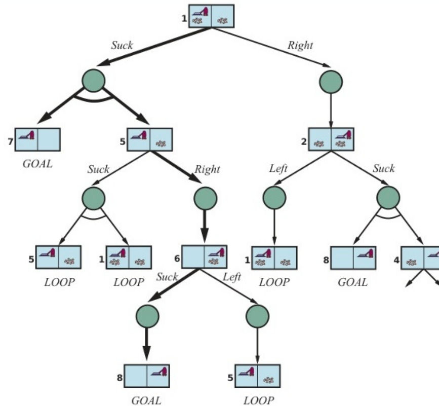
Figure 4: Mô hình cây AND-OR xử lý hệ quả không tắt định trong bài toán hút bụi.
