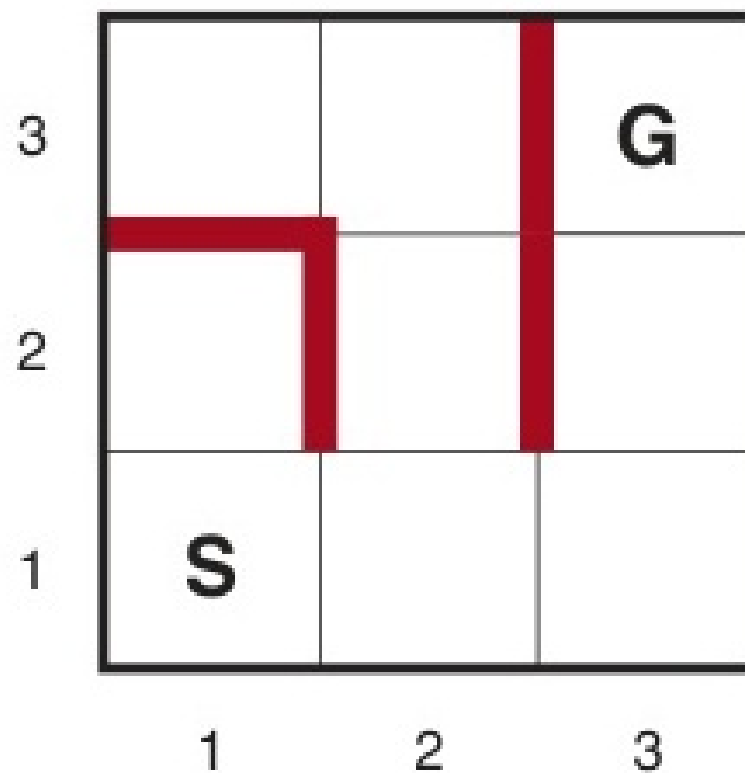
Figure 6: Robot bị kẹt (dead end) vĩnh viễn do không biết trước cấu trúc hành lang.
