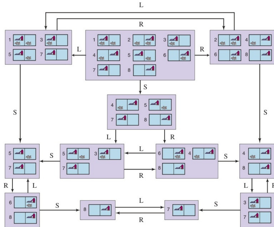
Figure 5: Sự chuyển đổi tập hợp Belief states của robot hút bụi khi không có cảm biến.
