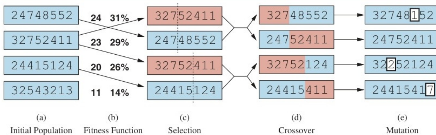
Figure 3: Tiến hóa (Đánh giá, Lựa chọn, Lai ghép, Đột biến) trong bài toán 8-Queens.
