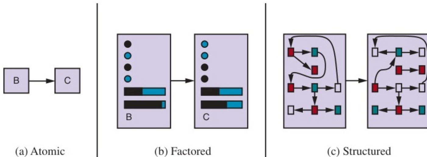
Figure 16: Ba cách biểu diễn trạng thái: Nguyên tử, Phân tách, Có cấu trúc.
