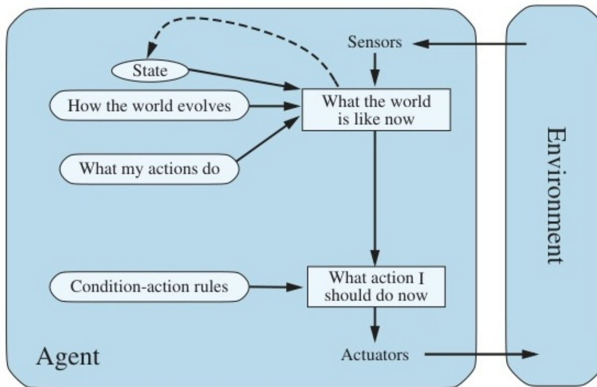
Figure 11: Mô hình Tác nhân phản xạ dựa trên mô hình (Model-based reflex agent).
