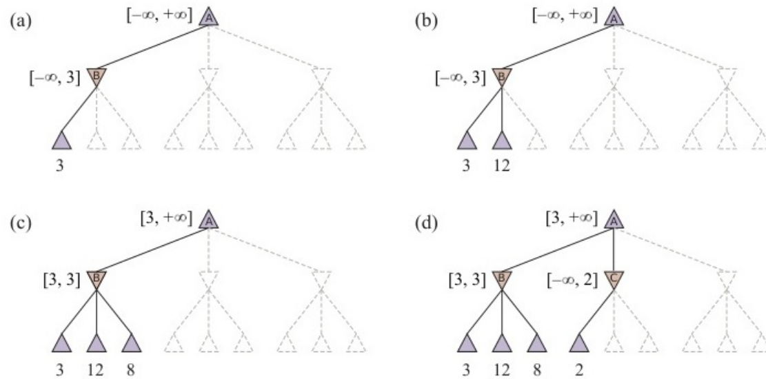
Figure 5: Mô phỏng cắt tỉa: Nhánh thứ 3 bị bỏ qua vì MIN chắc chắn sẽ ép giá trị xuống \leq 2 , trong khi MAX đã có nhánh khác đảm bảo giá trị lớn hơn là 3.
