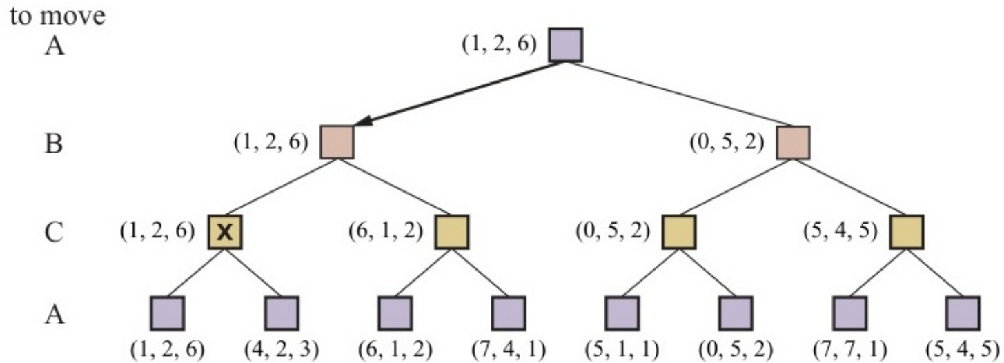
Figure 4: Ba ply đầu tiên của một cây trò chơi với ba người chơi (A, B, C).
