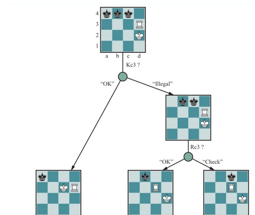
Figure 16: Tìm kiếm chiến lược trong điều kiện khuyết thiếu thông tin (VD: Tàn cuộc cờ vua mù - Kriegspiel).
