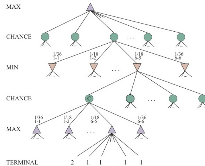
Figure 14: Mô phỏng cây trò chơi Expectiminimax với các nút tròn xúc xắc xen ngang.
