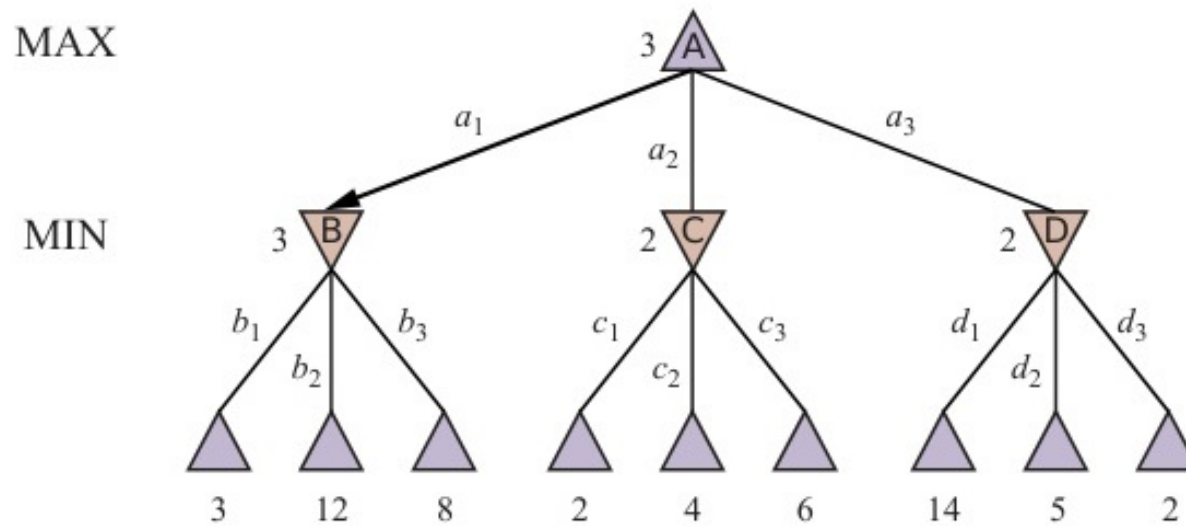
Figure 3: Hoạt động của Minimax: Gốc (MAX) sẽ chọn nước đi dẫn tới giá trị 3 (Cao nhất trong các lựa chọn ép buộc của MIN).
