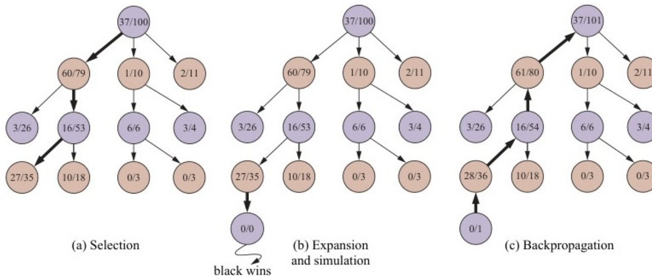
Figure 11: Quá trình chọn một nước đi bằng MCTS sử dụng số liệu lựa chọn UCT.
