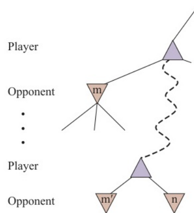
Figure 6: Trường hợp tổng quát cho việc cắt tỉa alpha-beta trên cây trò chơi.
