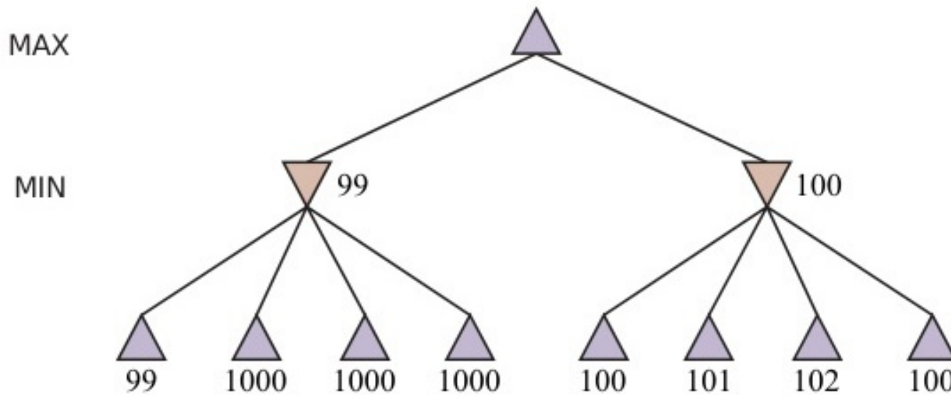
Figure 9: Một cây trò chơi hai ply mà heuristic minimax có thể mắc lỗi trong việc ra quyết định do đánh giá không chính xác ở độ sâu cạn.
