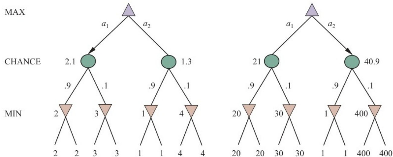
Figure 15: Một phép biến đổi bảo toàn thứ tự trên các giá trị lá có thể làm thay đổi nước đi tốt nhất.
