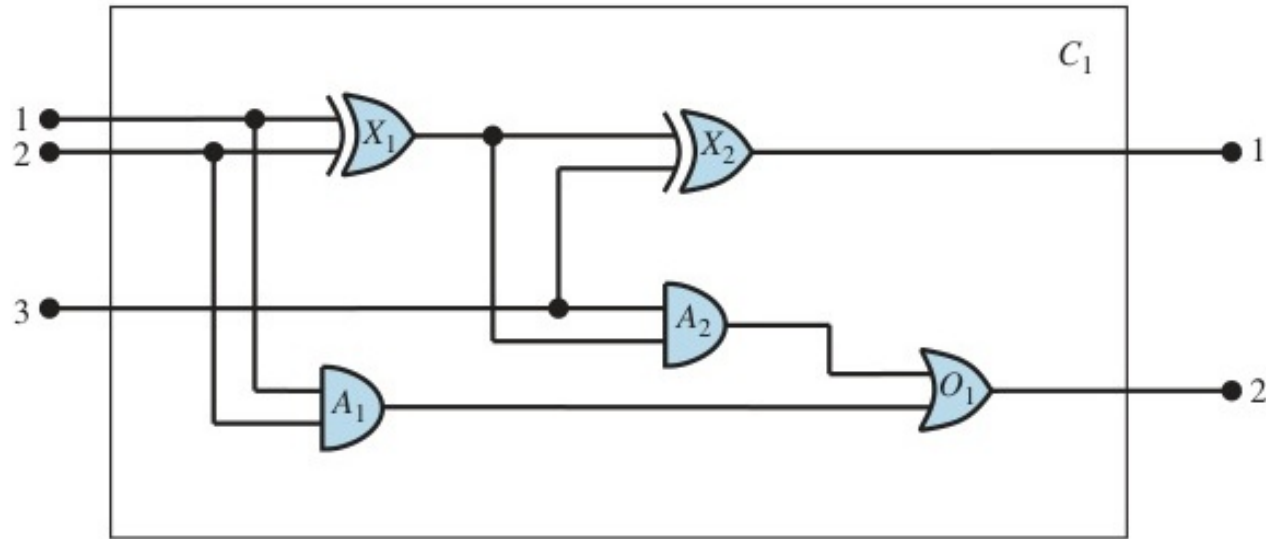
Figure 6: Một mạch kỹ thuật số (bộ cộng đầy đủ 1-bit), có thể được biểu diễn và chẩn đoán lỗi bằng FOL.
