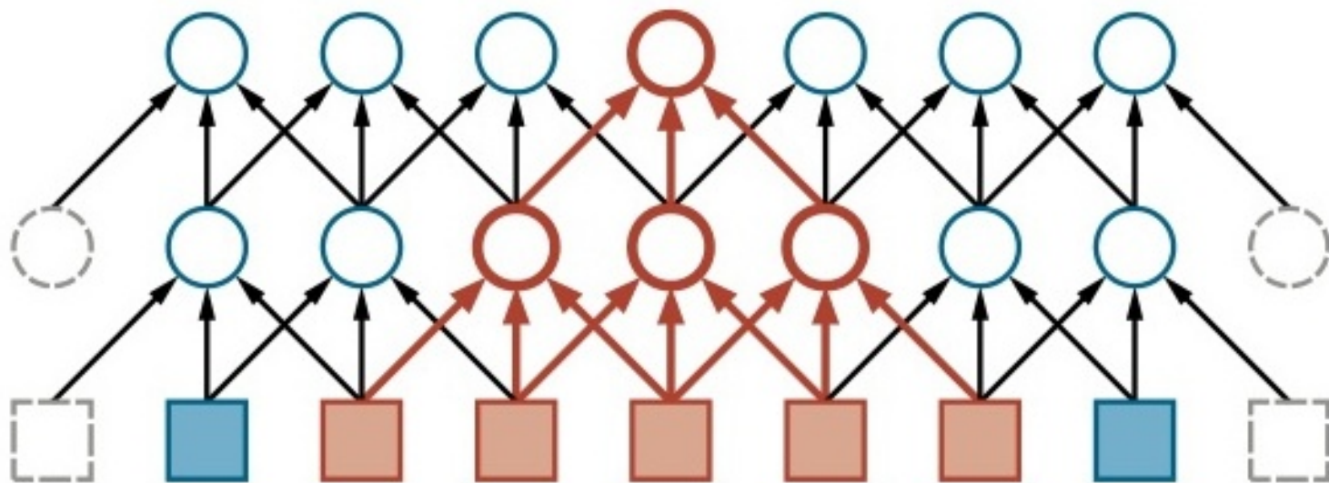
Figure 3: Hai tầng đầu tiên của một mạng Nơ-ron Tích chập (CNN) kết nối cục bộ các điểm dữ liệu.
