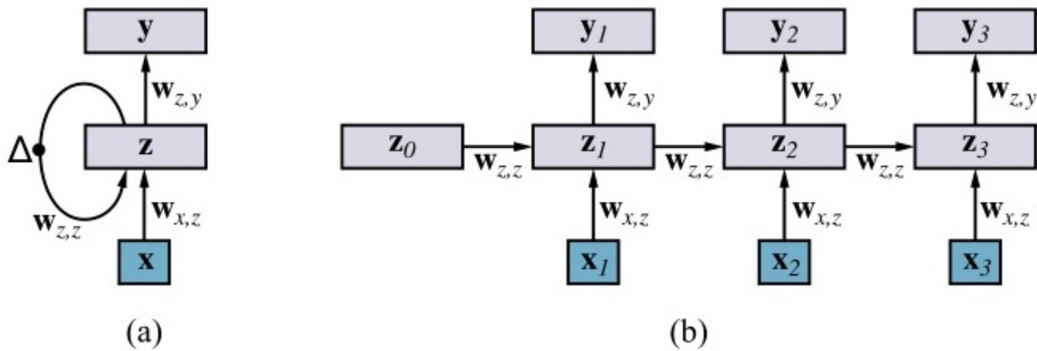
Figure 6: Sơ đồ của một Mạng Nơ-ron Hồi quy (RNN) có vòng lặp thời gian truyền trạng thái ẩn.
