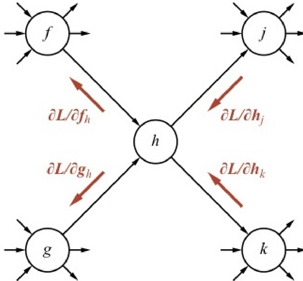
Figure 4: Minh họa quá trình Lan truyền ngược (Backpropagation) thông tin gradient trên đồ thị tính toán.
