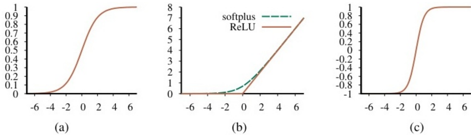
Figure 1: Các hàm kích hoạt thường được sử dụng trong học sâu: Hàm Sigmoid, Tanh, ReLU, Softplus.
