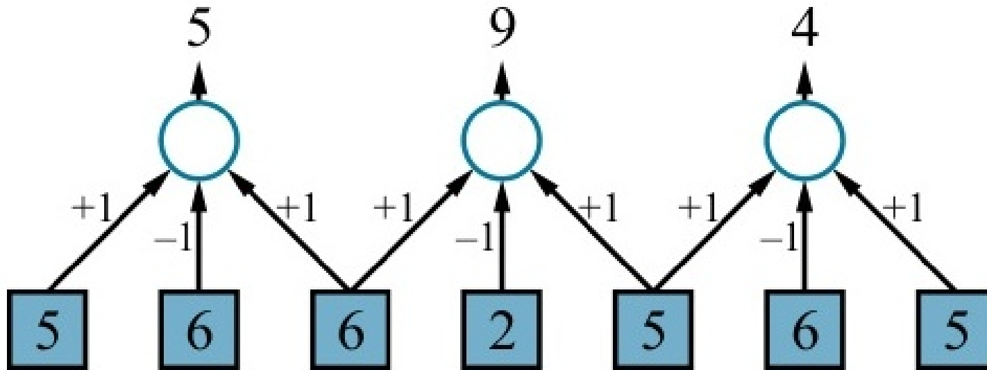
Figure 2: Hoạt động của Tích chập (Convolution) trượt bộ lọc qua ảnh để trích xuất đặc trưng.
