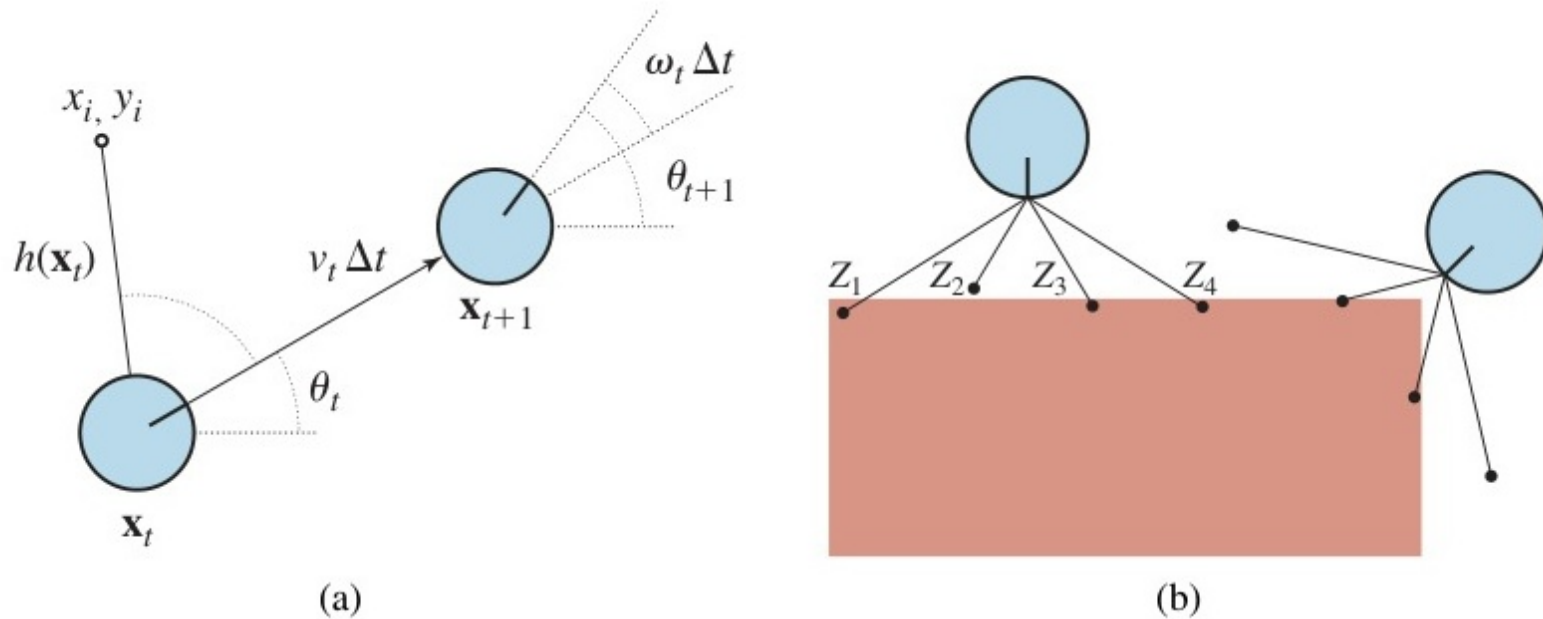
Figure 5: Phép đo xa bằng 4 tia laser giúp thu hẹp các khả năng vị trí (Pose) hiện tại của robot.
