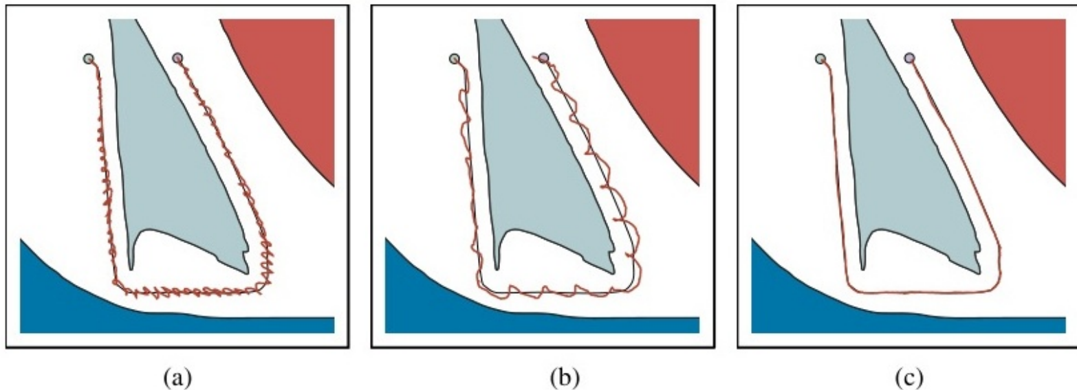
Figure 22: Minh họa lỗi vọt lố (overshoot) và đi zigzag của bộ điều khiển tỷ lệ đơn giản.
