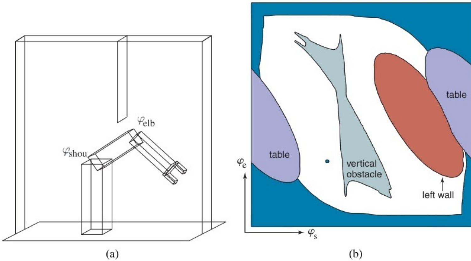
Figure 12: Các vùng tối là cấu hình va chạm của một cánh tay 2 khớp khi đối mặt với chướng ngại vật thẳng đứng.
