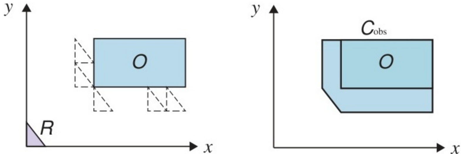
Figure 11: Chướng ngại vật trong C-space được mở rộng để bù đắp cho kích thước thực của robot tam giác.
