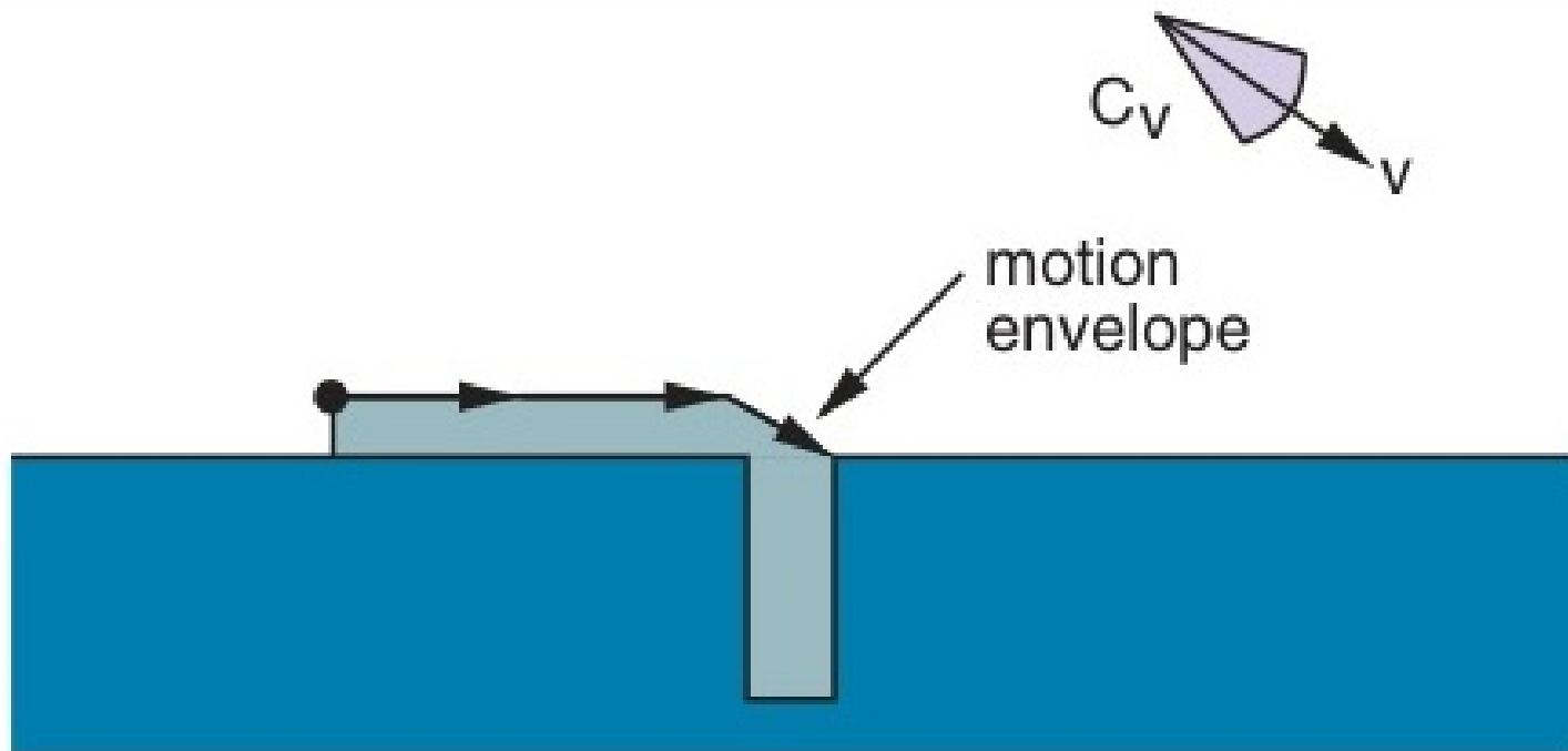
Figure 25: Bước 2: Trượt dọc theo tường cho đến khi trượt thành công vào bên trong lỗ.
