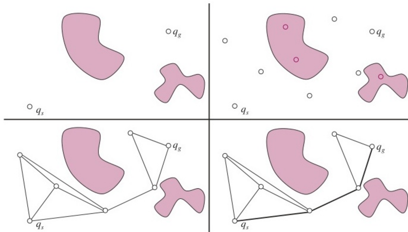
Figure 17: Thuật toán PRM: Rải điểm (mốc), nối mạng, và tìm đường trong cấu hình an toàn.
