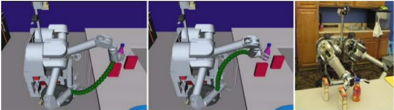
Figure 21: Bài toán tay máy lấy chai nước. Trái: Quỹ đạo ban đầu cứng kèn. Giữa & Phải: Quỹ đạo mềm mại sau khi tối ưu hóa.
