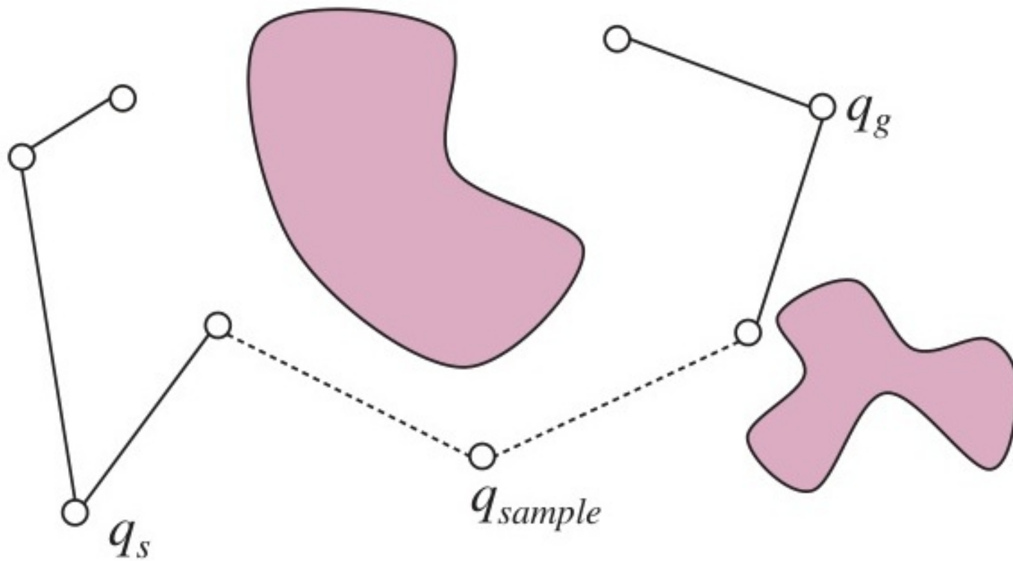
Figure 18: Hai cây RRT đang lan rộng và kết nối lại với nhau ở giữa không gian cầu hình.
