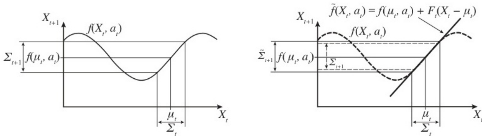
Figure 8: Tuyến tính hóa mô hình chuyển động phi tuyến bằng một hàm tuyến tính tiếp tuyến.
