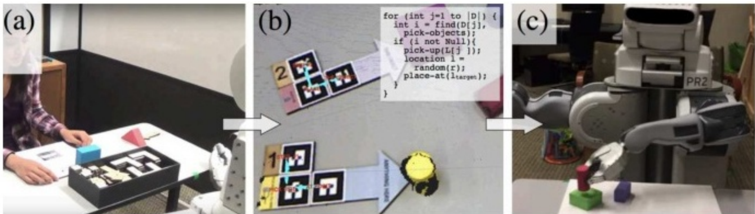
Figure 31: Lập trình tác vụ robot dựa trên việc xếp các khối trực quan trên bàn làm việc.
