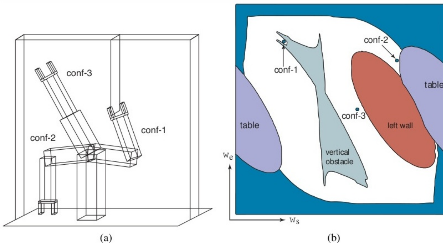
Figure 13: Ba cấu hình của tay máy trong không gian làm việc (trái) và biểu diễn của chúng như 3 điểm trong C-space (phải).
